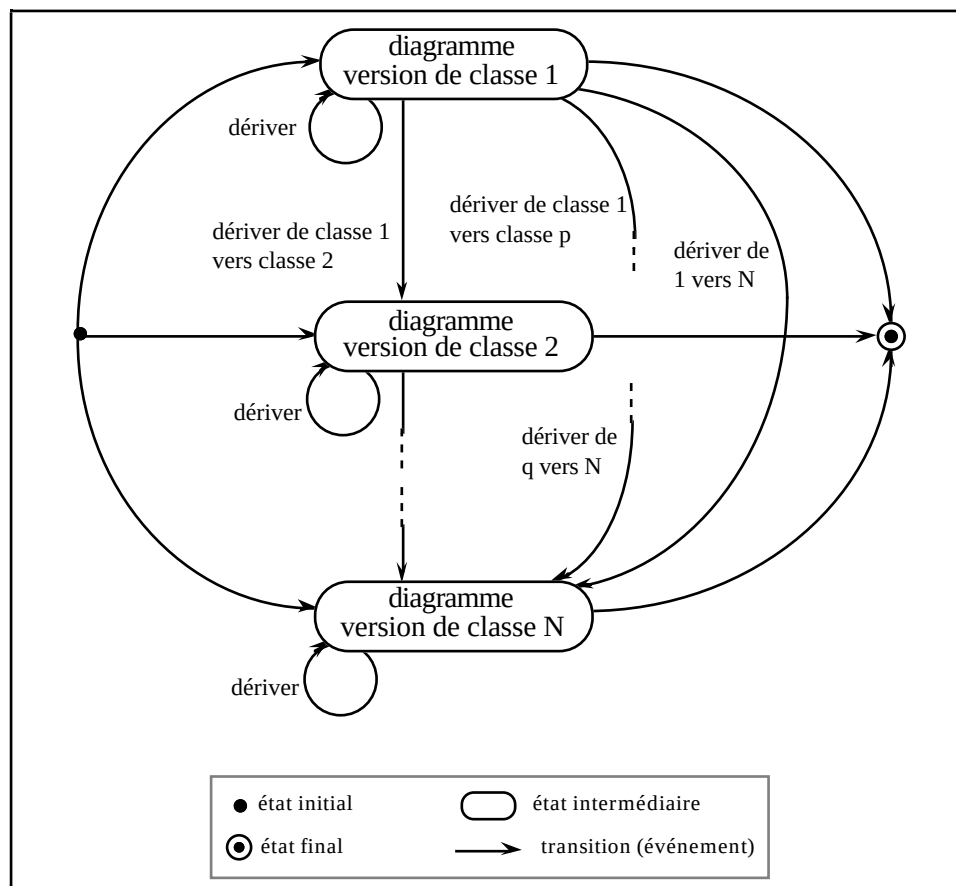
Figure II-31 : Diagramme d'état regroupant les diagrammes des versions d'une classe
