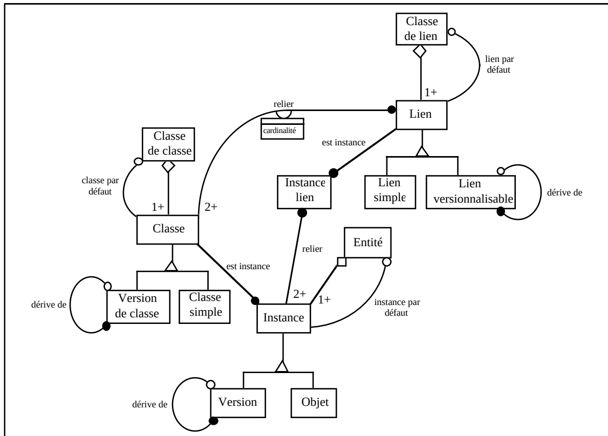
Figure IV-2 : Le méta-modèle
