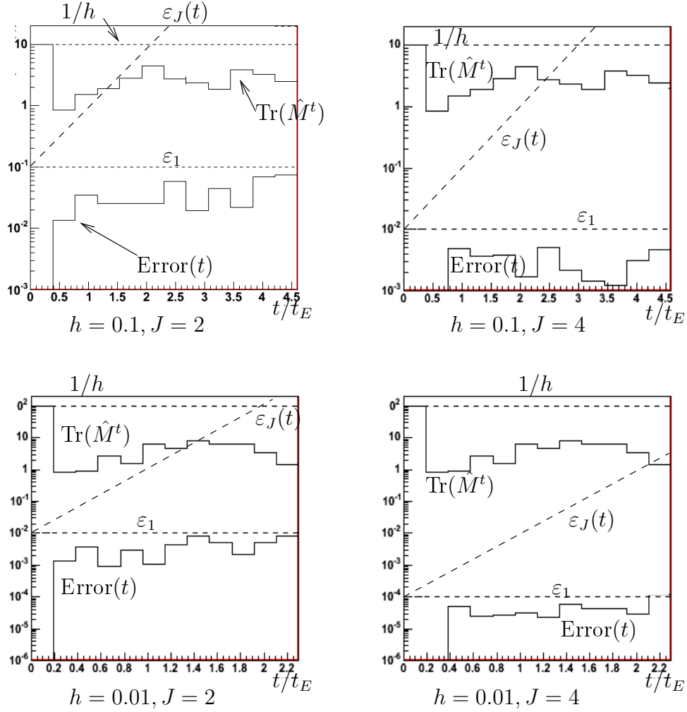
FIG. 28 – Comparaison de \text{Tr}(\hat{M}^t) calculé numériquement avec la formule semi-classique T_{\text{semi},t,J} . On représente |\text{Tr}(\hat{M}^t)| et \text{Error}(t) = |\text{Tr}(\hat{M}^t) - T_{\text{semi},t,J}| , pour t = 0, 1, \dots, 11 (il y a jusqu'à 39601 points périodiques). On représente la majoration N = 1/h de la trace, la majoration de l'erreur |\text{Error}(t)| \leq \varepsilon_{t,J} = h^{\frac{1}{2}(J-t/t_E)} , et \varepsilon_1 = h^{J/2} . On a choisi la constante de Planck h = 0.1 puis h = 0.01 , et calculé les formes normales semi-classiques des orbites périodiques jusqu'à l'ordre J = 2 et J = 4 . On observe le fait étonnant que \text{Error}(t) < \varepsilon_1 , bien que seulement \text{Error} < \varepsilon_{t,J} soit prouvé.
