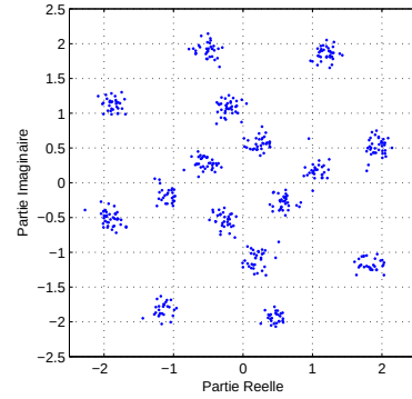
FIG. 4.10 – Constellation des échantillons reçus sur la seconde antenne. Communication MIMO (2,2) utilisant une modulation QPSK et un codage de type Multiplexage Spatial ( N=512 , \text{SNR}=20\text{dB} ).
