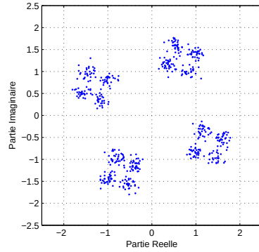
FIG. 4.9 – Constellation des échantillons reçus sur la première antenne. Communication MIMO (2,2) utilisant une modulation QPSK et un codage de type Multiplexage Spatial ( N=512 , \text{SNR}=20\text{dB} ).
