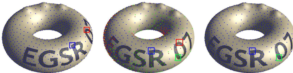
FIG. 4.5 – Distribution de points temporellement cohérente. (Gauche) Les points sont distribués en espace image. Ici on utilise la luminance pour guider la densité. Les points sont ensuite projetés sur l’objet 3D. (Milieu) L’objet est déplacé et les points reprojetés en espace image. Les points rouges sont supprimés, les points bleus sont conservés et les points verts sont ajoutés. Les points jaunes ne eux sont plus visibles. (Droite) Résultat finale de la distribution.
