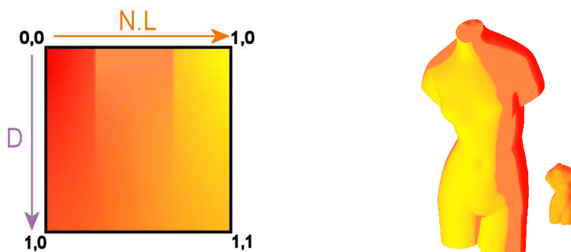
FIG. 2.7 – Xtoon : (à gauche) une texture 2d est utilisée pour contrôler l'éclairage ( N.L ) en fonction d'un paramètre de détail D . Par exemple (à droite) D peut être la profondeur depuis la caméra.
