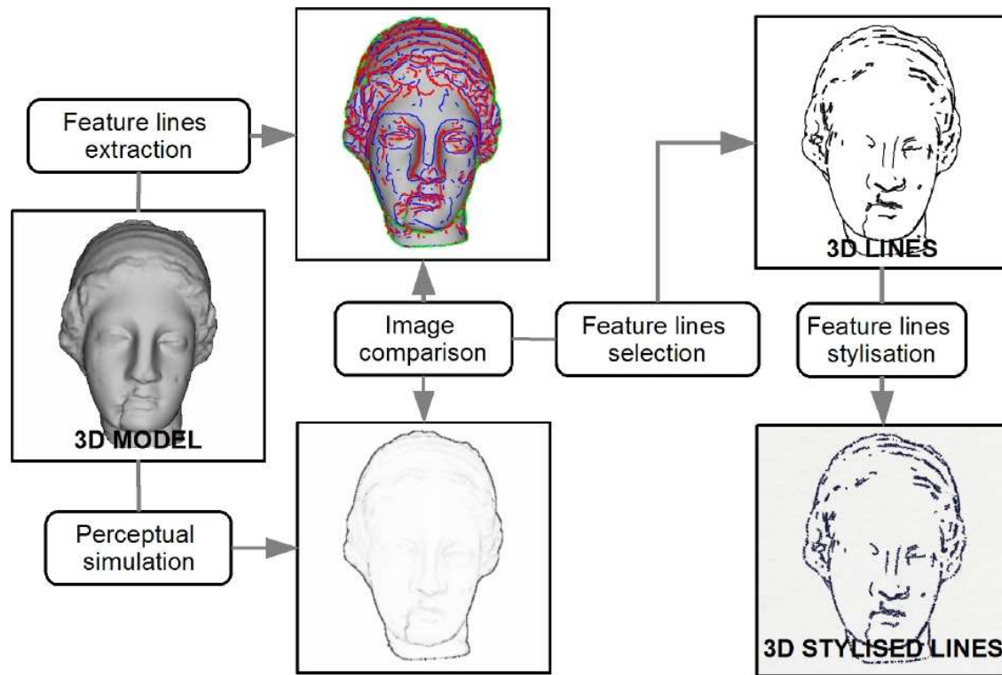
FIG. 3.7 – Pipeline d'extraction de lignes caractéristiques.
