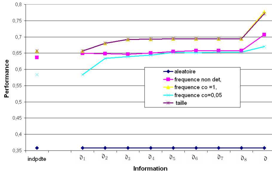
Figure III.24 : Performances globales des heuristiques.
