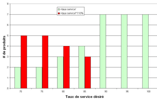
(c) Information totale, \delta (instances homogènes).
