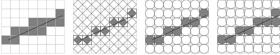
FIG. 4.5 – Quelques exemples de modèles analytiques : supercouverture, naïf fermé, pythagoricien et engendré par un pentagone.
