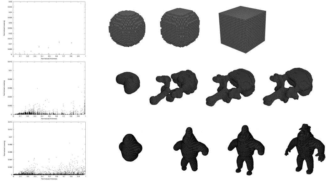
FIG. 8.9 – Illustration du filtrage en dimension 3 : graphes de filtrage et reconstruction du plus grossier au plus fin des objets discrets.
