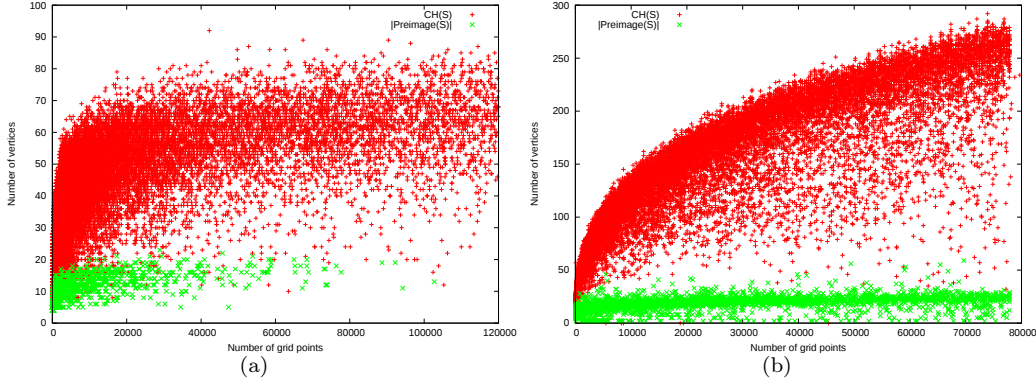
FIG. 5.9 – Analyse comparée de |CH(S)| et |P(S)| pour la dimension 3 pour les plans discrets à base hyper-rectangulaire (a) et co-sphérique (b).
