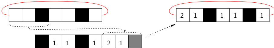
FIG. 7.21 – Illustration de la première étape pour la transformée en distance torique : sélection du point de rupture, recodage en vecteur et réécriture du résultat.
