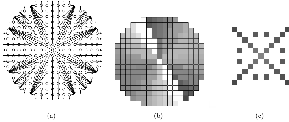
FIG. 7.8 – Résultats sur un disque discret.
