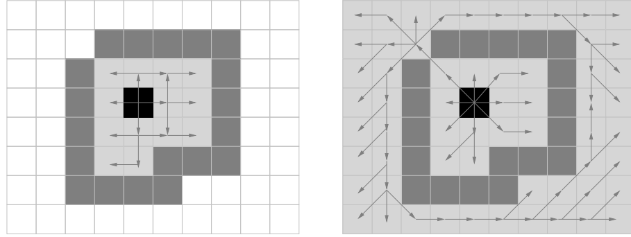
FIG. 3.8 – Illustration d’un remplissage d’objet à partir du pixel noir en (1)–connectié ( gauche ) et en (0)–connectié ( droite ). Les flèches illustrent un exemple de propagation selon la connectivité considérée.
