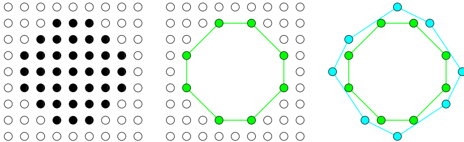
FIG. 5.10 – Illustration du processus global de filtrage pour la reconnaissance de disques discrets.
