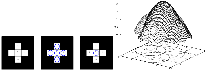
FIG. 7.15 – De gauche à droite, une forme discrète X et sa transformée en distance euclidienne ; les 5 centres des boules dont le dôme touche l'enveloppe supérieure des paraboloides, dessinée à droite ; l'axe médian discret est formé du seul point central encerclé ; forme continue Y et enveloppe supérieure des paraboloides bordant la forme \hat{Y} .
