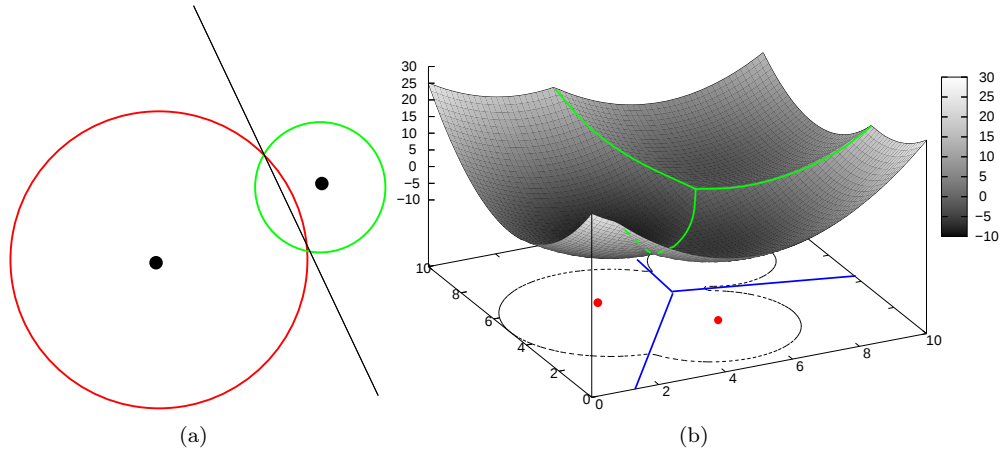
FIG. 7.19 – (a) Diagramme de puissance associé à deux boules de rayons différents. (b) Représentation surfacique du diagramme avec des paraboloïdes elliptiques.
