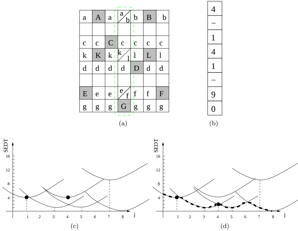
FIG. 7.6 – Représentation de la décomposition en dimension pour le calcul du diagramme de VORONOÏ discret. (a) : Image en entrée (les pixels de \overline{X} sont en gris), et résultat de l'étiquetage selon l'axe des x . Les collisions sont indiquées par des doubles lettres. (b) : la valeur de transformée en distance de la colonne i = 4 . (c) : L'ensemble des paraboles pour la colonne i = 4 . Les points indiquent les collisions ( \#\Pi_{Sp} > 1 ) détectées dans la dimension précédente. (d) : l'enveloppe inférieure des paraboles et détection des nouveaux points tels que \#\Pi_{Sp} > 1 : le point j = 7 n'est plus sur une arête du diagramme, le point j = 1 est préservé et un nouveau point équidistant+ de plusieurs sites a été détecté j = 4 .
