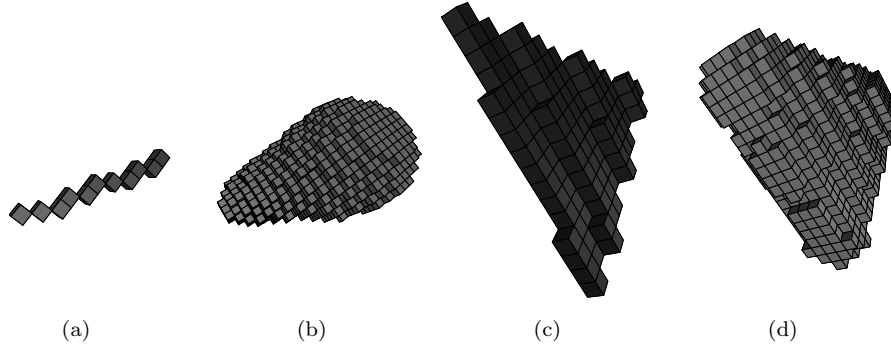
FIG. 8.11 – Pseudo-tronc de cône et pseudo-triangle 3D.
