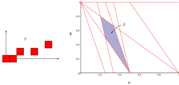
FIG. 5.2 – Préimage d'un ensemble de points discrets S .
