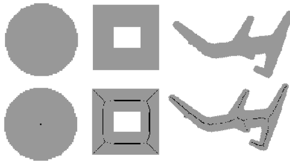
FIG. 7.17 – Extraction de l'AMD en dimension 2 : la première ligne présente les objets discrets, la seconde présente les centres de boules du AMD (pixels en noir).
