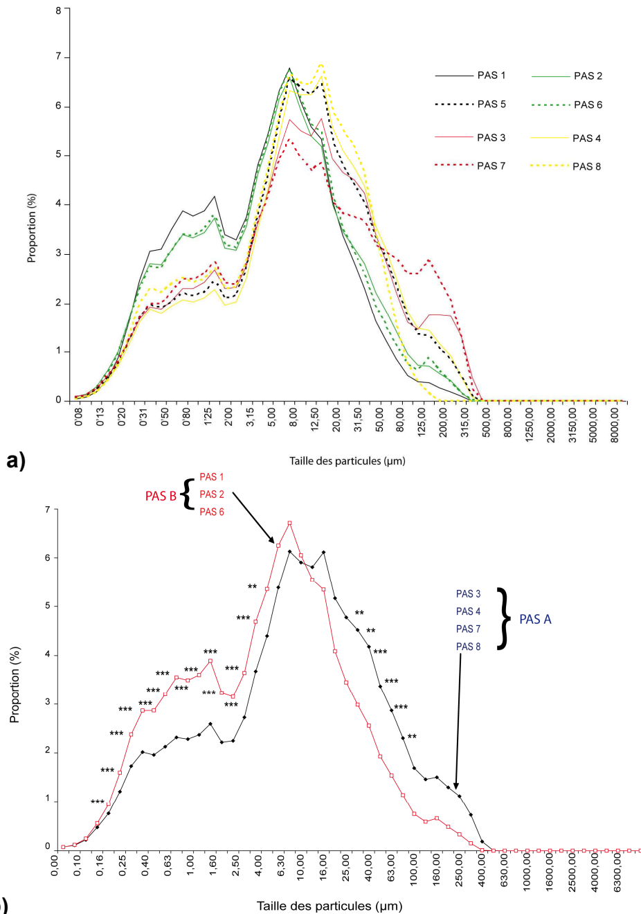
Figure III 3 : Comparaison des courbes granulométriques \mathcal{L} des 8 stations de la zone de clapages PAS 1 à 8 en mai 2004. a) 8 courbes de PAS; b) Courbes moyennes des 2 classes déterminées par l'algorithme de classification par les k-moyennes.
