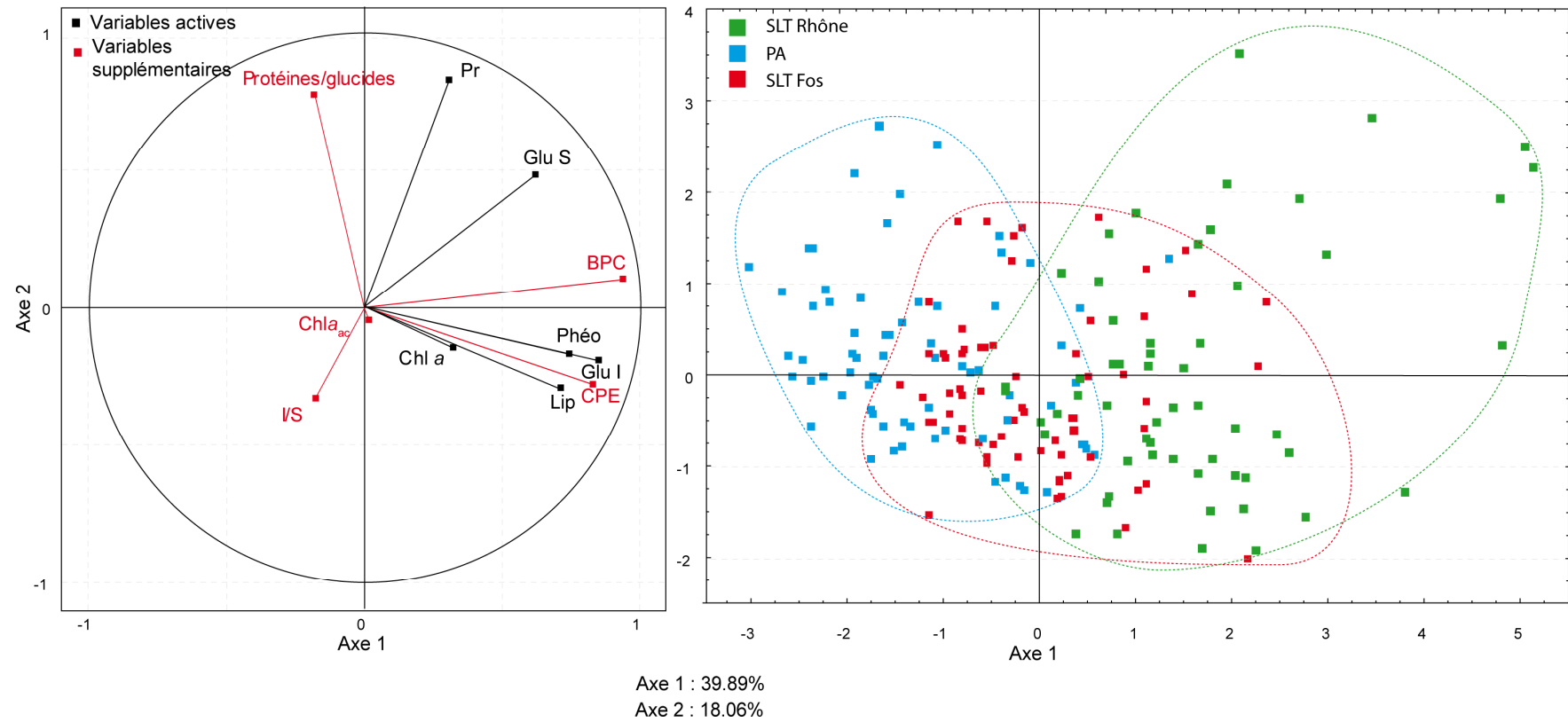
Figure III 22 : ACP normée réalisée avec 6 variables actives (Pr, Glu I , Glu S , Lip, Chla, Phéo) et 5 variables supplémentaires : (\frac{I}{S}, \frac{Pr}{Glu}, Chla_{ac}, BPC et CPE) . N = 198 : SLT Fos, PA et SLT Rhône – 2 centimètres superficiels.
