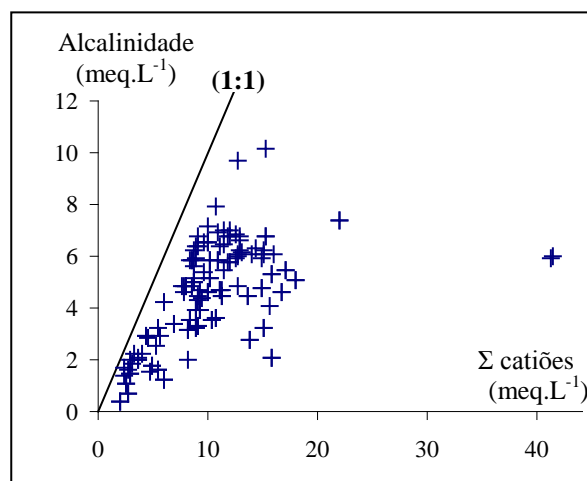
Figura IV-20: Alcalinidade vs \Sigma cátions [Na^+ + K^+ + Ca^{2+} + Mg^{2+}] para as amostras de água do aquífero aluvial.
