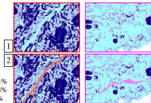
Figura VI-6: Mapa de declividades das bacias do Forquilha e V. Alegre para os intervalos [0-4], [4-8] e > 8%; Detalhes do mapa de declividades das bacias do Forquilha (vermelho) e V. Alegre (roxo) sem [1] e com [2] os limites dos aquíferos aluviais (áreas coloridas) definidos a partir das observações de campo e de foto- interpretação das imagens SPOT 5 (2002 e 2003) com resolução espacial 5 m.
