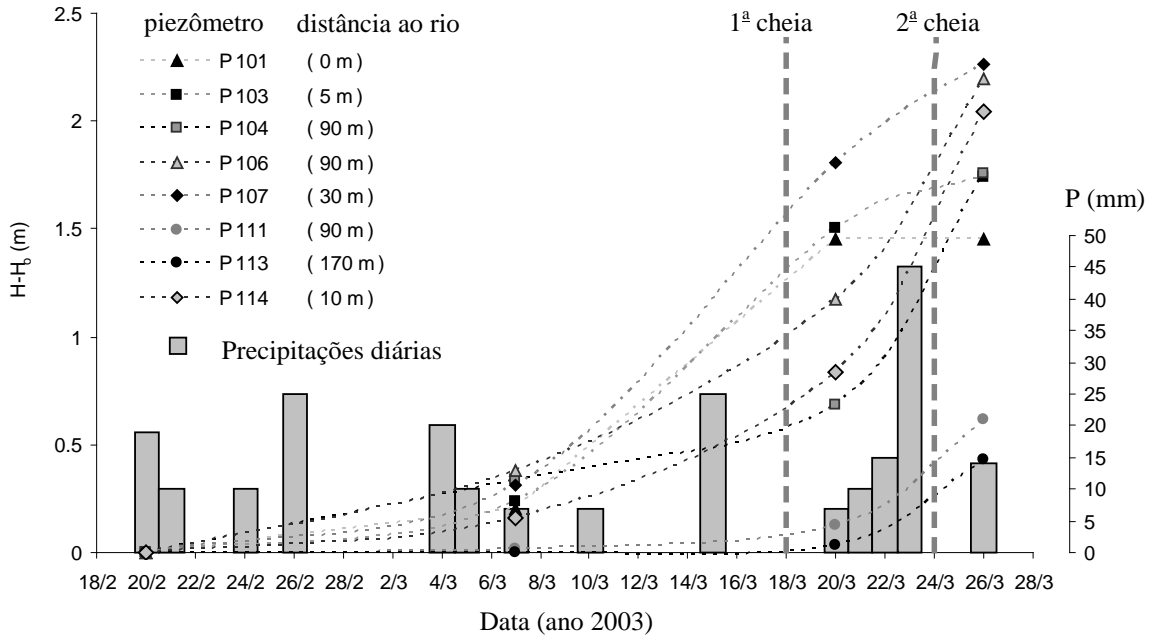
Figura IV-5: Evolução dos níveis piezométricos (H) de 20/02/2003 (início da estação chuvosa) até 26/03/2003 com relação ao nível do 20/02/2003 (H 0 ) para diferentes piezômetros localizados em distâncias de 0 a 170 m do riacho e precipitações diárias registradas em São Bento.
