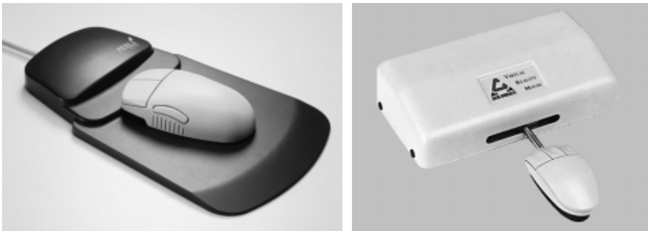
Figure 2.2 souris à retour de force : la Feelit de Immerse Corporation et la Virtual Reality Mouse de Control Advancements
