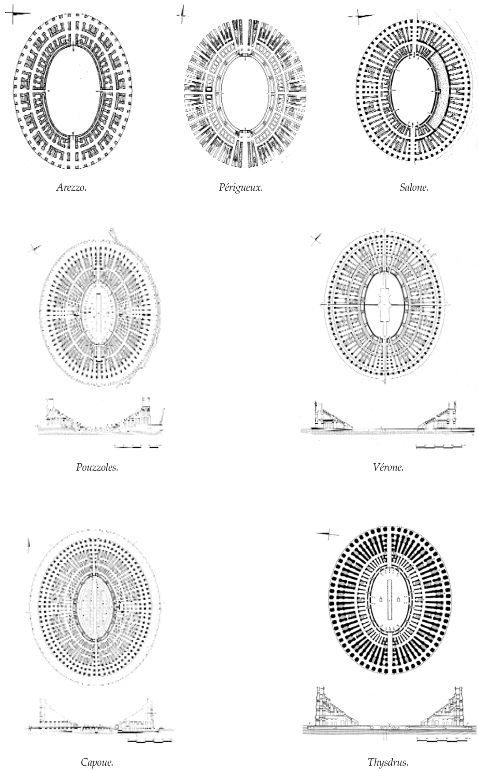
Fig. 374. Plans et coupes des amphithéâtres dits « à structure creuse », d'après J.-Cl. GOLVIN, 1987.
