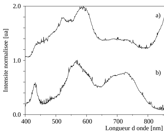
FIG. 3.5 – Spectres typiques du rayonnement de transition cohérent obtenu pour L = 30 mm.
