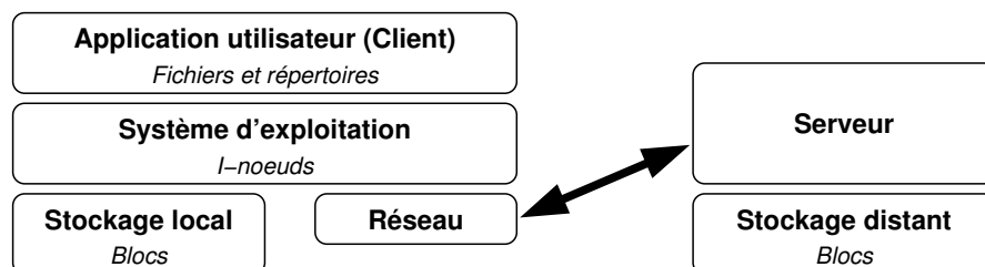
FIG. 2.1: Stockage local et distribué.
