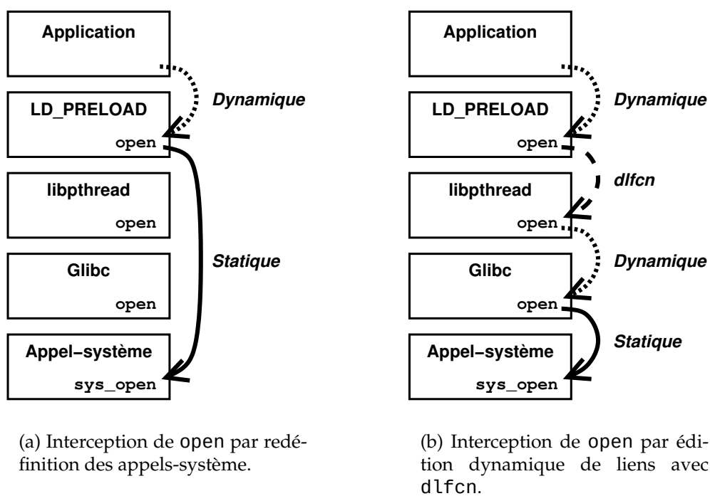
FIG. C.2: Interception de l'appel open par une bibliothèque préchargée par la variable d'environnement LD_PRELOAD .
