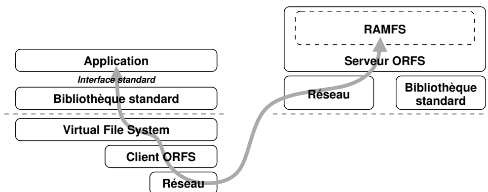
FIG. 5.5: Modèle de ORFS accédant à un serveur de fichiers en mémoire (RAMFS).
