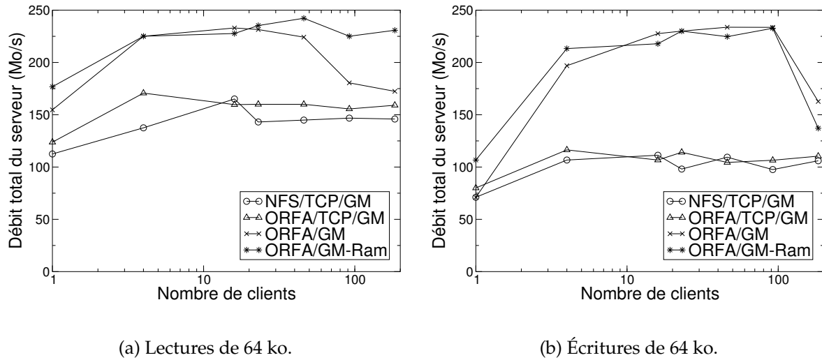
FIG. 4.5: Performances des lectures et écritures séquentielles dans un fichier pour des requêtes de 64 ko (de 1 à 184 clients).
