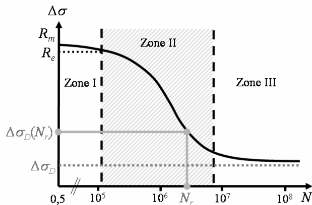
Figure 1.2 : domaines de fatigue
