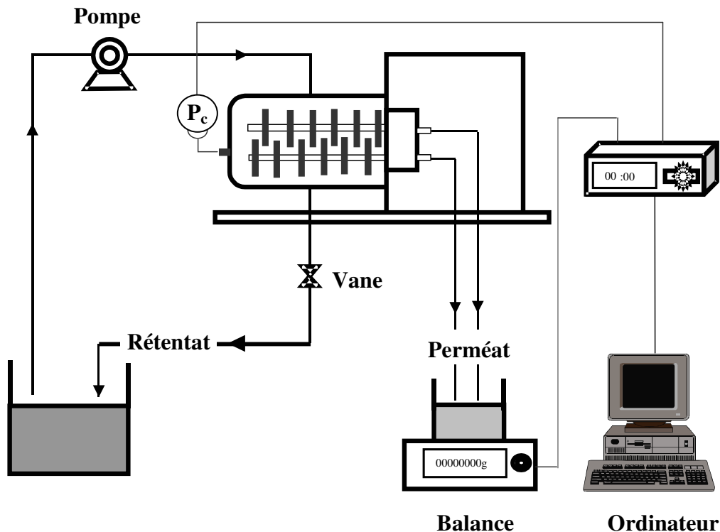
Figure 2.4 Montage expérimental lors des essais sur MSD
