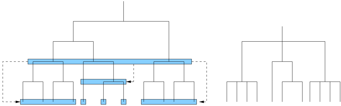
Figure 6.2: Selection de niveaux avec l'algorithme 4. La figure de droite est l'arbre initial. Les niveaux présentant des minima du critère ICL sont représentés par des rectangles gris. La figure de droite représente l'arbre obtenu après la sélection des niveaux : seuls les niveaux ayant un minimum du critère ICL apparaissent.
