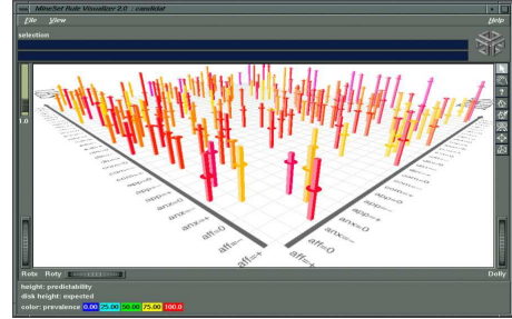
(b) Mineset 3
