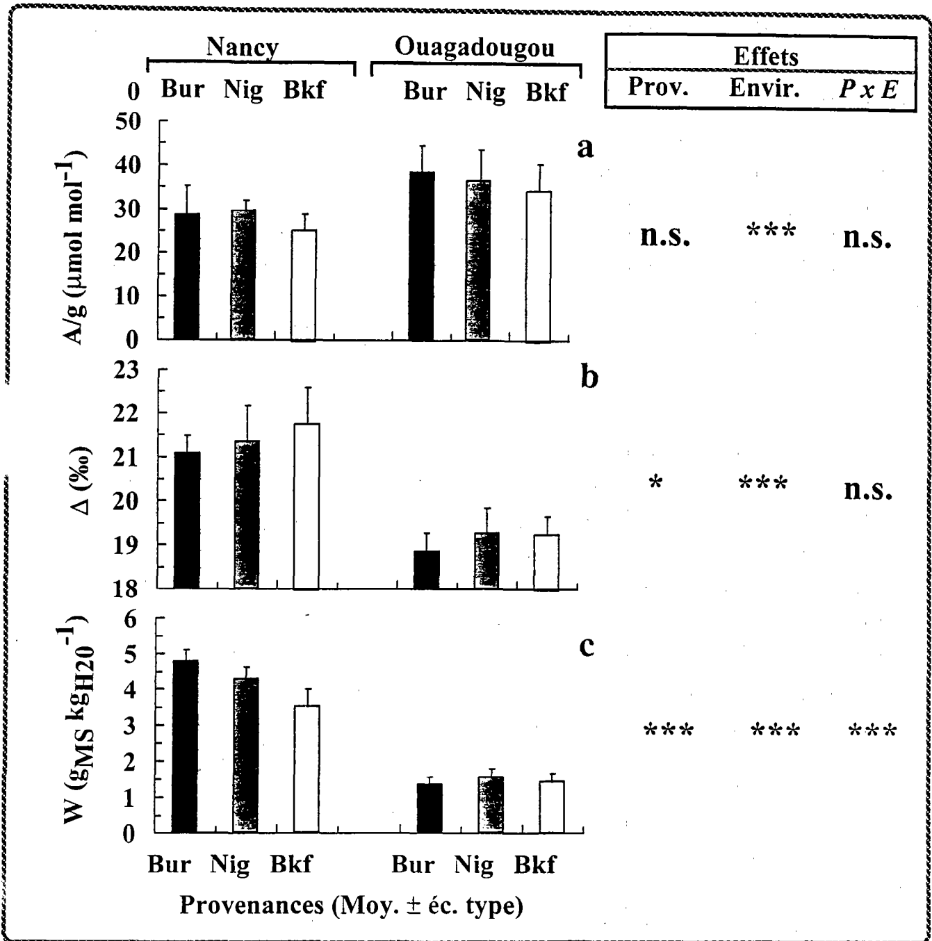
Figure 42 : Comparaison de A/g, \Delta et W de provenances de Faidherbia albida en pots, dans deux sites expérimentaux, INRA-Nancy, France & INERA-Productions Forestières-Ouagadougou, Burkina Faso.
