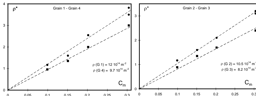
Figure 7-20. Densités de dislocations réelles dans les grains 1, 2, 3 et 4.
