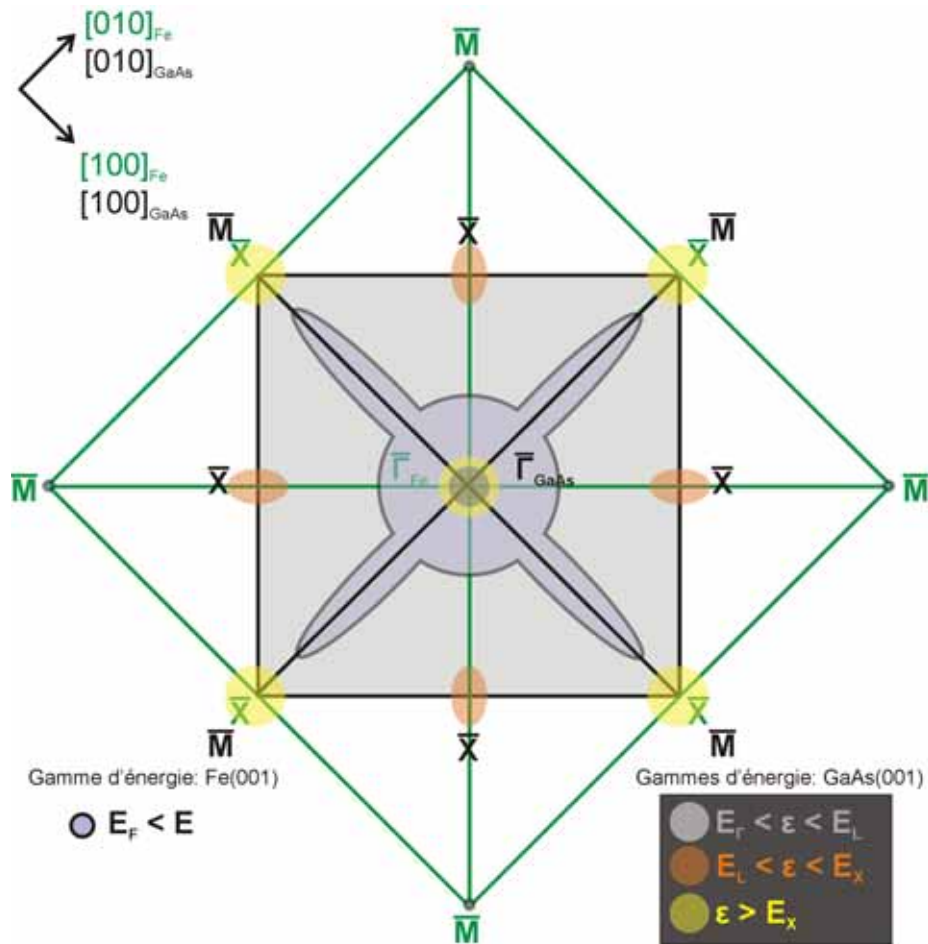
Figure 70: Superposition des zones de Brillouin 2D de Fe(001) et GaAs(001). Les densités d'états dans GaAs(001) et les zones des points \bar{k} des électrons autorisés dans Fe(001) sont indiquées par les mêmes disques que pour les figures 48 et 69, en rappelant ici les énergies des électrons correspondant à ces zones.
