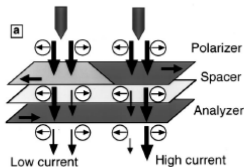
Figure 78: Schéma du modèle à deux courants pour la GMR sur une vanne de spin montrant des variations de courant BEEM directement reliées à l'orientation des aimantations respectives des deux couches ferromagnétiques (d'après [12]).
