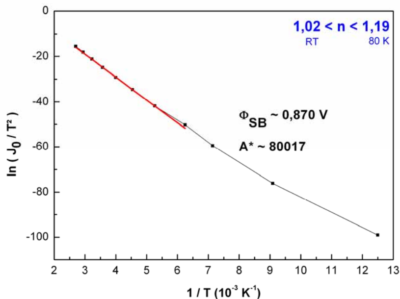
Figure 34: Courbe de Richardson obtenue à partir des caractéristiques J(V) à différentes températures, sur un plot de surface S \sim 10^7 \text{ m}^2 d'un échantillon Au/GaAs(001).
