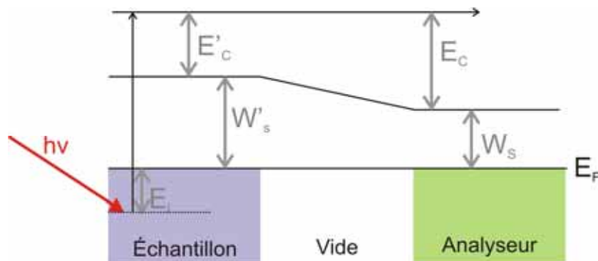
Figure A.2: Schéma du potentiel vu par un photoélectron d'énergie de liaison E_l éclairé par des photons d'énergie h\nu . E_C' et E_C correspondent à l'énergie cinétique du photoélectron à la sortie de l'échantillon et à l'entrée de l'analyseur, respectivement. W_s' et W_s sont respectivement les travaux de sortie de l'échantillon et de l'analyseur.
