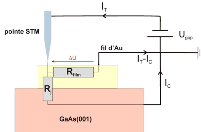
Figure 16: Schéma du contact du fil d'Or sur un plot métallique. La résistance de jonction et la résistance dans le plan du film sont notées R_J et R_{film} , respectivement.
