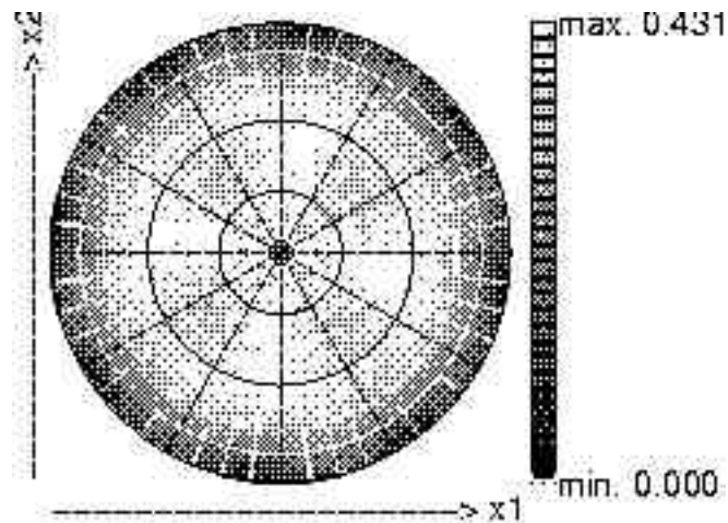
Figure 4-11. Figure de pôles d'un tenseur \mathbb{C} tétraogonal dans sa configuration tétraogonale 4 Le même tenseur est tourné autour de \mathbf{x}^3 cette configuration est appelée "tétraogonale 4" par les cristallographes.
