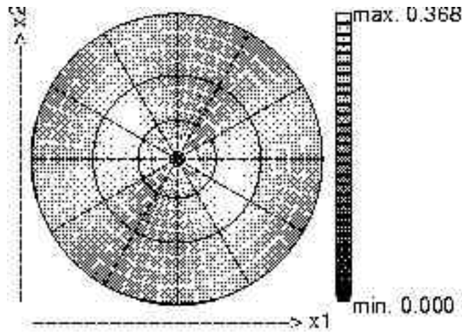
Figure 4-15. Figure de pôles d'un tenseur \mathbb{C} monoclinique dans sa base "naturelle" Le seul plan de symétrie de ce tenseur (table 8-7) apparaît : le plan orthogonal à \mathbf{x}^3 .
