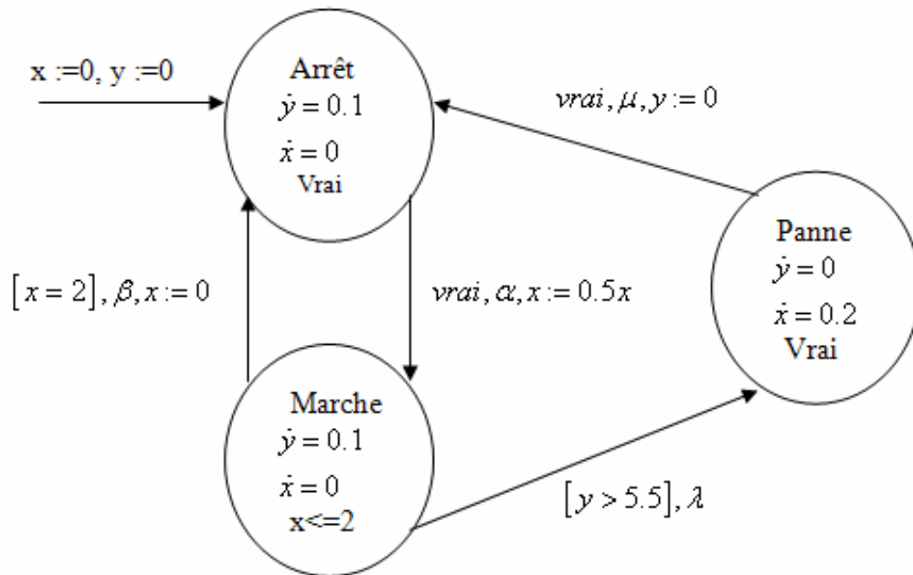
Figure 2.1 Exemple d'automate hybride modélisant une machine simple
