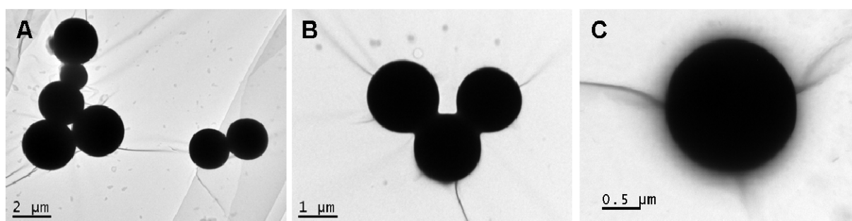
Figure 38. Observation par microscopie électronique à transmission des structures supramoléculaires résultant de l'assemblage entre le LYS et l'apo \alpha -LA pour une concentration protéique totale de 0,2 mM. Le LYS et l'apo \alpha -LA ont été mélangés dans des proportions équimolaires à 45°C. Les barres d'échelle sont de 2 \mu\text{m} (A), 1 \mu\text{m} (B) et 500 nm (C).
