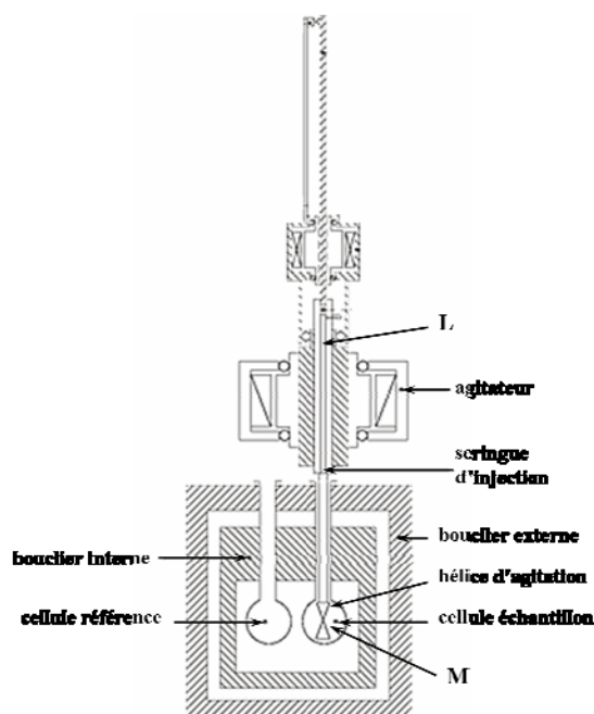
Figure 16. Schéma du microcalorimètre et de la seringue d'injection.
