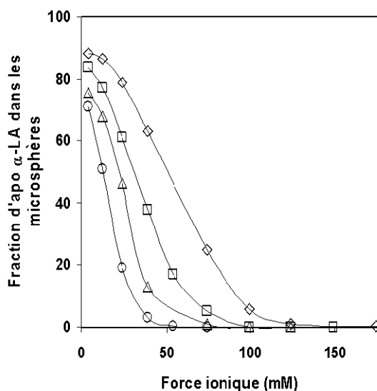
Figure 29. Fraction d'apo \alpha -LA incluse dans les microsphères LYS/apo \alpha -LA en fonction de la force ionique de la solution pour différentes concentrations protéiques totales : 0,085 mM (○), 0,15 mM (Δ), 0,3 mM (□) et 0,53 mM (◇). Le LYS et l'apo \alpha -LA étaient mélangés en proportion équimolaire à 45°C.
