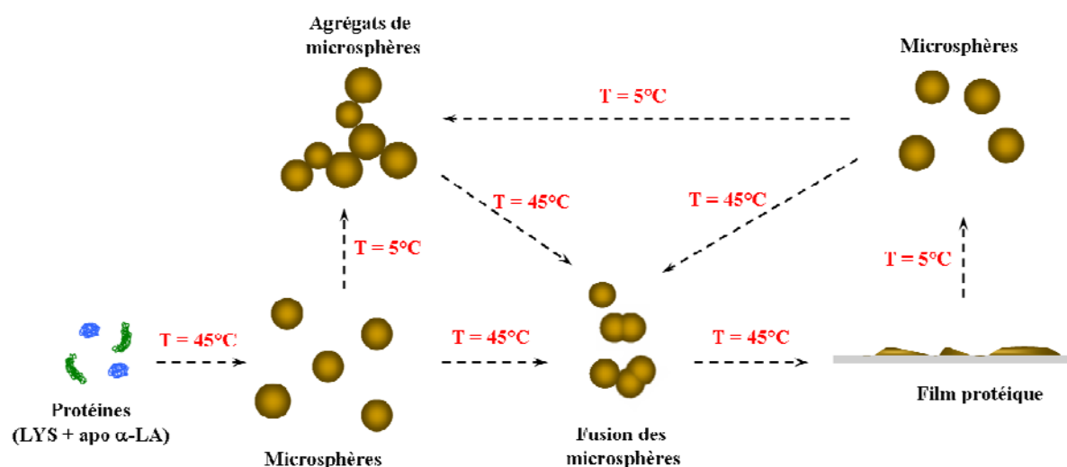
Figure 33. Schéma bilan représentant l'influence de la température sur la stabilité des microsphères résultant de l'assemblage entre l'apo α-LA et le LYS à 45°C.
