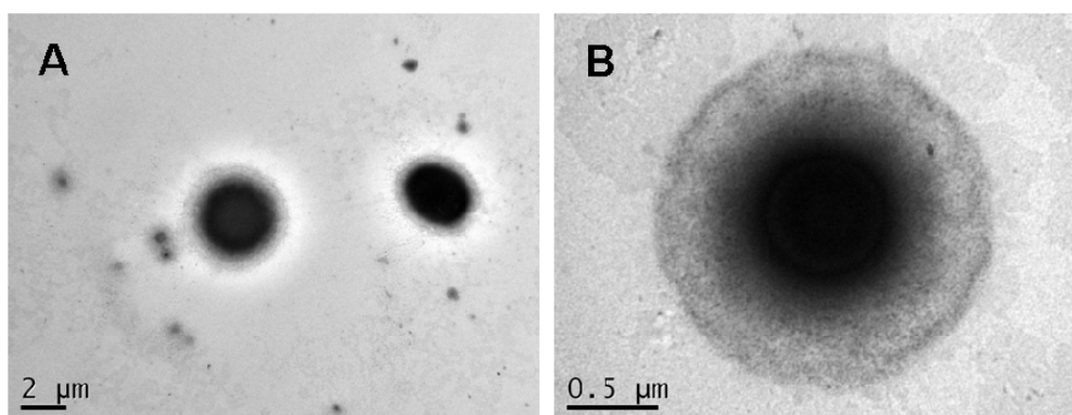
Figure 34. Clichés de microscopie électronique à transmission obtenus après la déstabilisation des microsphères préformées entre le LYS et l'apo \alpha -LA à 45°C par l'ajout d'une solution de calcium. Le rapport molaire final \text{Ca}^{2+} /apo \alpha -LA est de 1.
