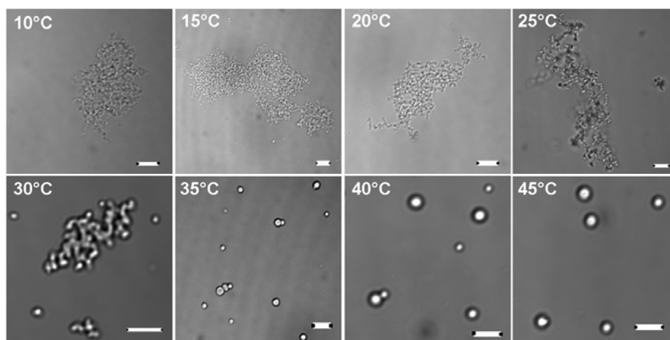
Figure 25. Observation par microscopie optique des structures supramoléculaires résultant de l'assemblage entre le LYS et l'apo \alpha -LA en fonction de la température. Les barres d'échelle sont de 5 \mu m (10°C, 15°C, 20°C et 25°C) et 3 \mu m (30°C, 35°C, 40°C et 45°C).
