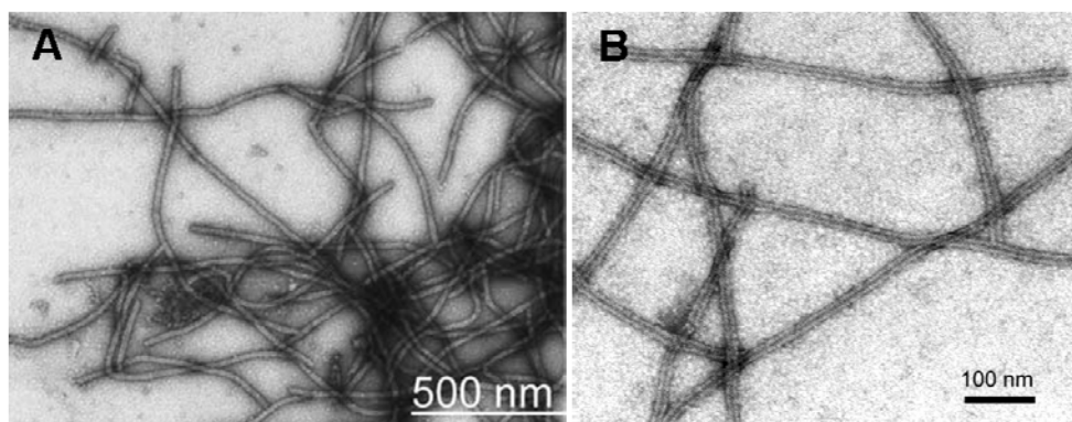
Figure 10. Observation de nanotubes résultant de l'assemblage de l' \alpha -lactalbumine partiellement hydrolysée par microscopie électronique à transmission (Graveland-Bikker et al., 2004; Graveland-Bikker et al., 2006).
