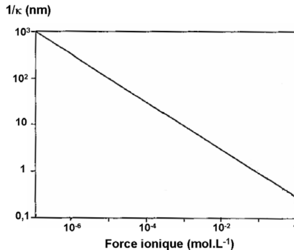
Figure 4. Influence de la force ionique sur la longueur de Debye-Hückel ( \kappa^{-1} ).
