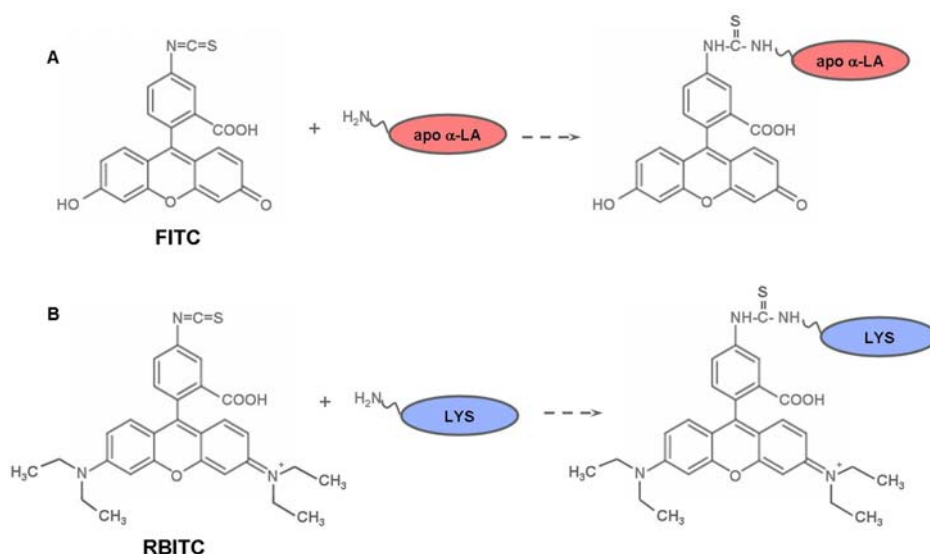
Figure 22. Schéma de la réaction de marquage de l'apo \alpha -LA par la fluorescéine isothiocyanate (A) et du LYS par la rhodamine B isothiocyanate (B).
