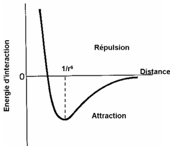
Figure 2. Energie potentiel en fonction de la distance interatomique (Potentiel de Lennard-Jones).
