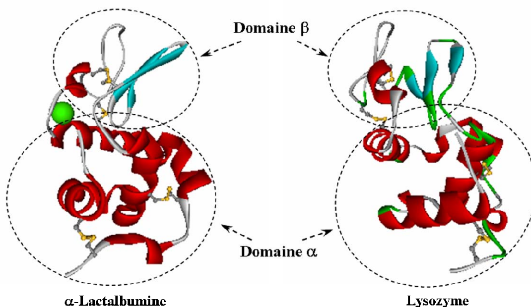
Figure 14. Structures secondaire et tertiaire de l' \alpha -lactalbumine (pdb : 1F6S) et du lysozyme (pdb : 6LYZ). Le calcium de l' \alpha -lactalbumine est représenté par une « sphère » verte au sein de la structure.
