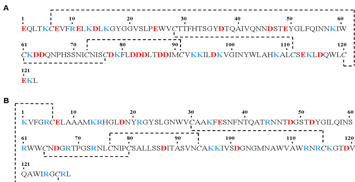
Figure 13. Structures primaires de l' \alpha -lactalbumine (A) et du lysozyme (B). Les acides aminés colorés en rouge et en bleu correspondent respectivement aux acides aminés acides et basiques. Les pointillés représentent les ponts disulfures.
