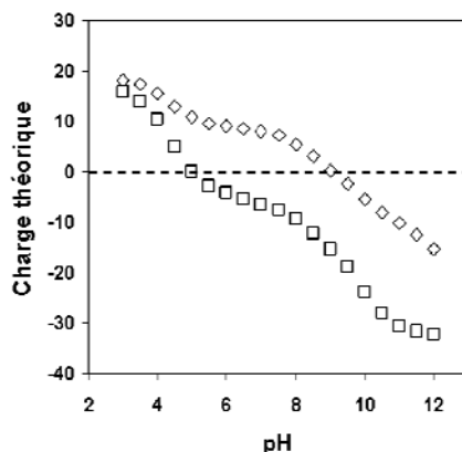
Figure 27. Charges théoriques du LYS (◇) et de l'α-LA (□) calculées à l'aide logiciel « protein calculator v3.3 ».
