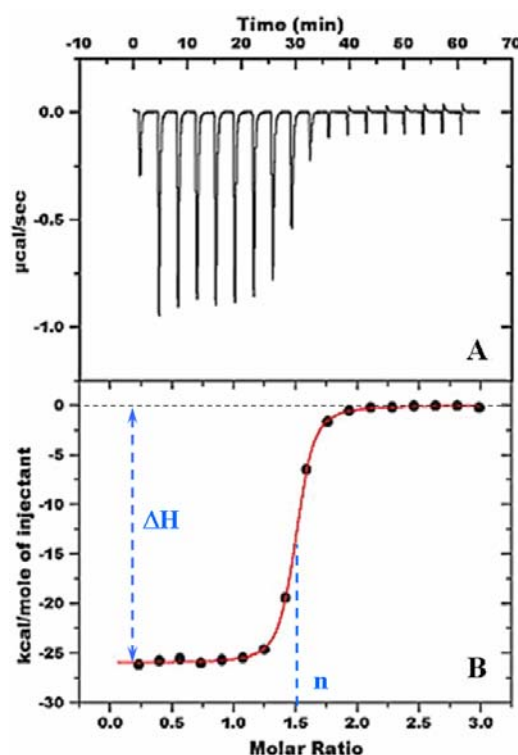
Figure 18. Exemple de profil ITC. Les données brutes sont représentées dans la figure 18A, chaque pic correspond à l'injection de ligand dans la cellule échantillon contenant la macromolécule. La figure 18B représente l'intégration de l'aire contenue sous chaque pic en fonction du rapport molaire (Ligand/Macromolécule).
