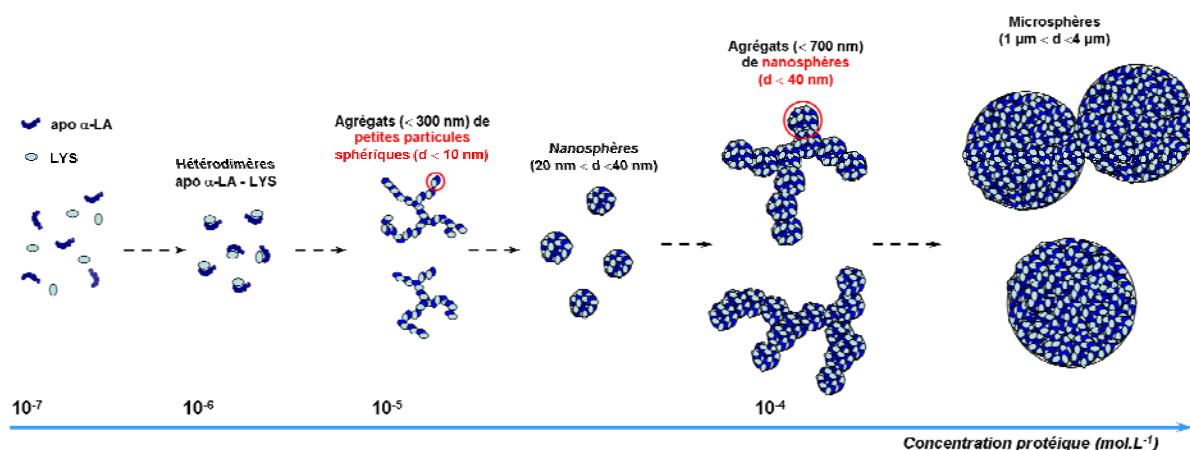
Figure 39. Mécanisme d'assemblage du LYS et de l'apo \alpha -LA de l'échelle moléculaire à l'échelle macroscopique.
