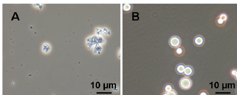
Figure 40. Structures supramoléculaires résultant de l'assemblage entre le LYS et l'apo \alpha -LA à 45°C : observation par microscopie à contraste de phase immédiatement (A) et 30 min (B) après mélange des protéines. La concentration protéique totale était de 0,53 mM pour un rapport équimolaire en LYS et apo \alpha -LA.
