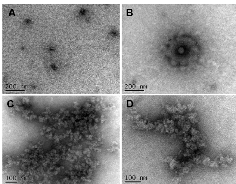
Figure 37. Observation par microscopie électronique à transmission des structures supramoléculaires résultant de l'assemblage entre le LYS et l'apo \alpha -LA pour une concentration protéique totale de 0,1 mM. Le LYS et l'apo \alpha -LA ont été mélangés dans des proportions équimolaires à 45°C. Les barres d'échelle sont de 200 nm (A et B) et 100 nm (C et D).
