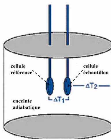
Figure 17. Schéma des deux dispositifs thermoélectriques présents au sein de la chambre adiabatique du microcalorimètre.
