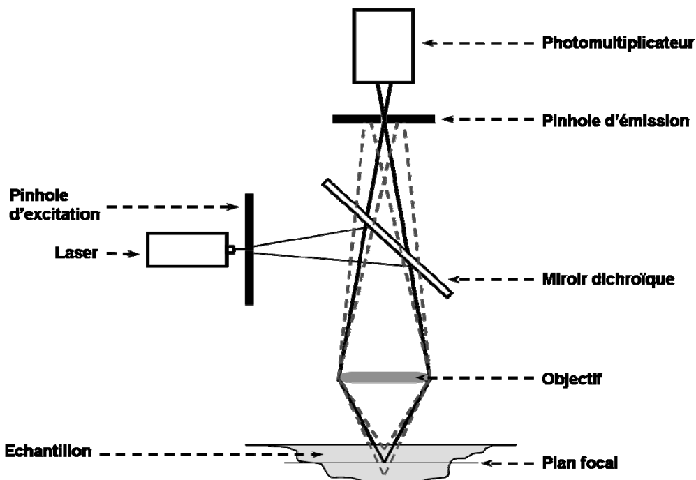
Figure 21. Principe de fonctionnement du microscope confocal à balayage laser.
