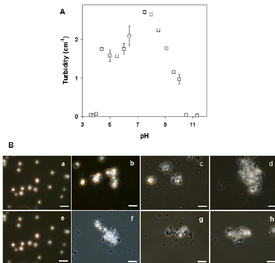
Figure 30. Influence du pH sur la stabilité des microsphères résultant de l'assemblage entre l'apo \alpha -LA et le LYS à 45°C. Turbidité des mélanges LYS/apo \alpha -LA après modification du pH par ajout de NaOH ou de HCL (A). Observation par microscopie optique à contraste de phase des structures supramoléculaires après la modification du pH : pH 7,5 (a et e), pH 6,5 (b), pH 5,5 (c), pH 4,4 (d), pH 8,5 (f), pH 9,5 (g), pH 10,0 (h).
