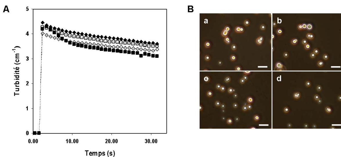
Figure 31. Cinétique d'assemblage entre le LYS et les acides poly-L-glutamiques PG28 ( \diamond , \blacksquare ) et PG60 ( \square , \blacksquare ) pour des rapports de concentration LYS/polymère identique (symboles ouverts) et de charge LYS/polymère identique (symboles pleins) (A). Observation par microscopie à contraste de phase des structures supramoléculaires LYS/PG28 (a) et LYS/PG60 (c) formées pour un rapport de concentration LYS/polymère identique, et LYS/PG28 (b) et LYS/PG60 (d) formées pour un rapport de charge identique (B). La barre d'échelle représente 10 \mu\text{m} .
