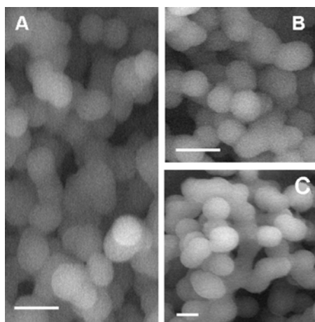
Figure 8. Observation par microscopie à balayage environnementale de particules sphériques résultant de l'assemblage de différentes protéines à leur point isoélectrique lors de traitement thermique (90°C) en présence de NaCl (0,1 M) : \beta -lactoglobuline (A), sérum albumine bovine (B) et lysozyme de blanc d'œuf de poule (C) (Krebs et al., 2007). Les barres d'échelle sont de 1 \mu m.
