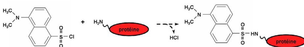
Figure 20. Schéma de la réaction de marquage du LYS, de l'holo et apo \alpha -LA par le chlorure de dansyl.
