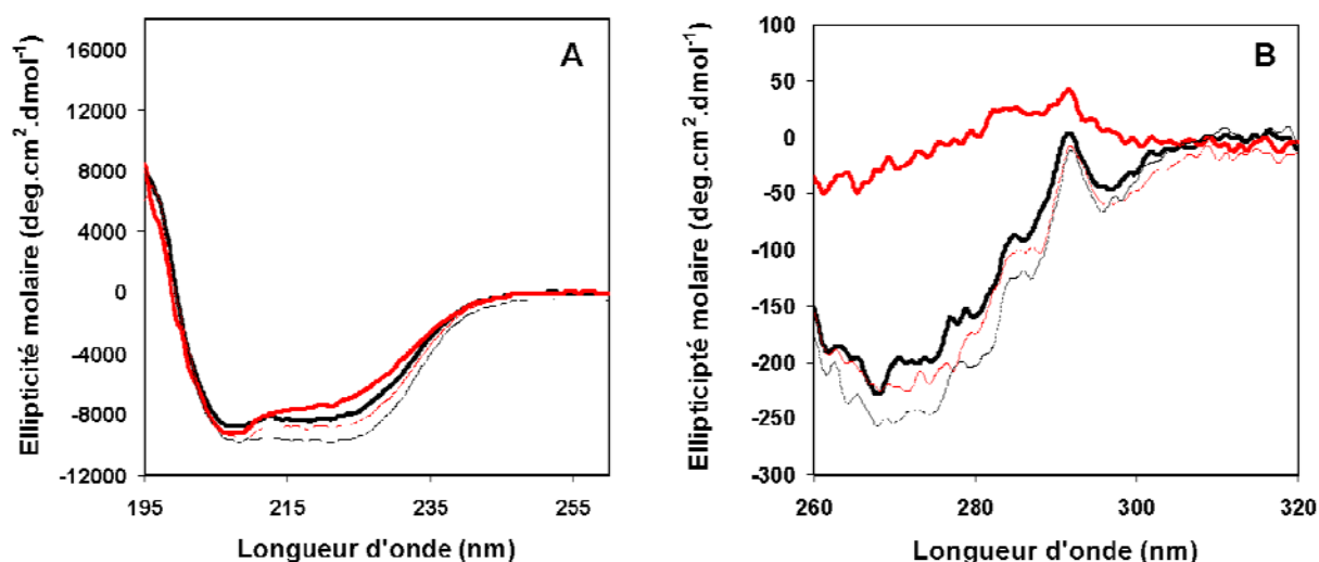
Figure 24. Spectres de dichroïsme circulaire de l'apo \alpha -LA (gras) et de l'holo \alpha -LA (fin) à 10°C (—) et 45°C (---) dans l'UV lointain (A) et le proche UV (B). Les spectres étaient acquis pour une concentration protéique de 0,148 et 1,48 g.L -1 respectivement dans l'UV lointain et l'UV proche et dans un tampon 30 mM Tris/HCl (pH 7,5), 15 mM NaCl.
