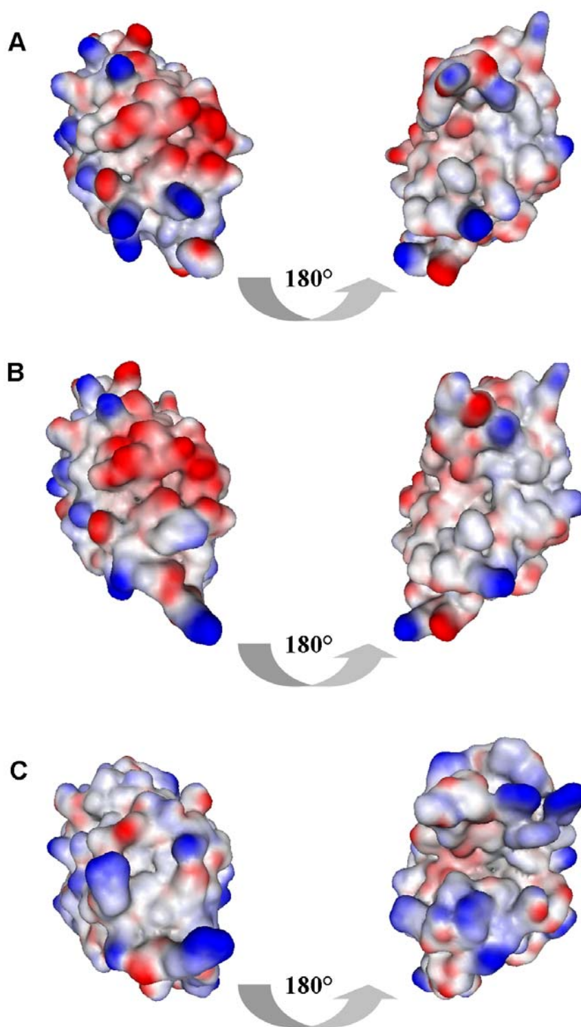
Figure 15. Potentiel électrostatique de surface de l'holo \alpha -lactalbumine (A), de l'apo \alpha -lactalbumine (B) et du lysozyme (C) calculé à pH 7,5 pour une force ionique de 39 mM par le programme Delphi inclut dans le logiciel Accelrys Molecular Graphics System.
