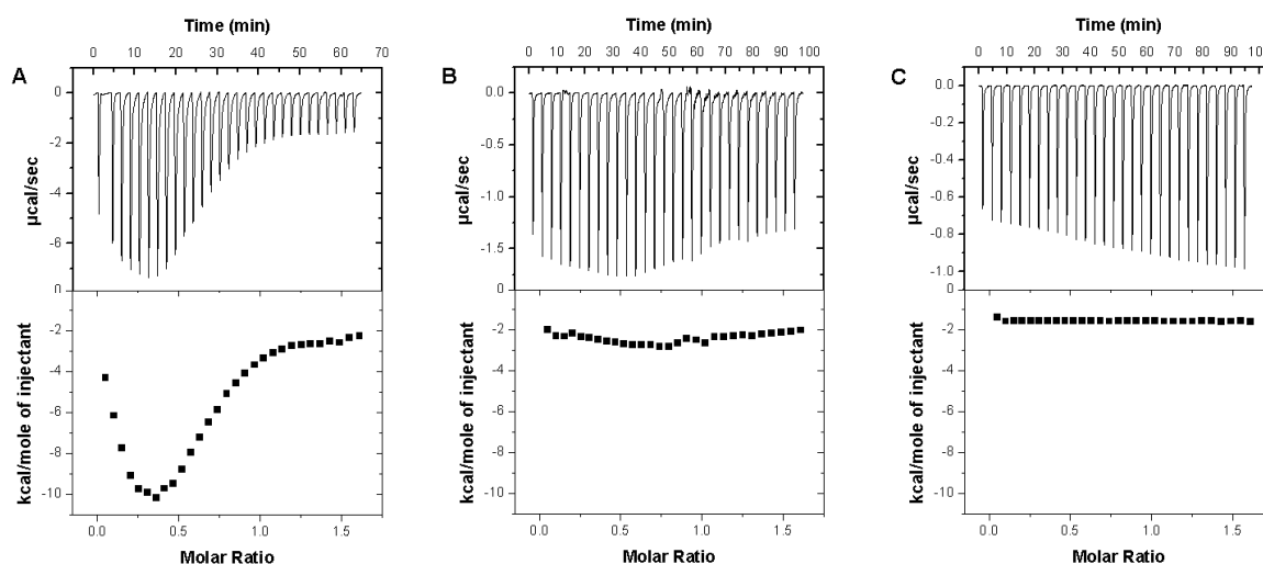
Figure 28. Interaction entre l'apo \alpha -LA et le LYS à 45°C observée par microcalorimétrie dans du tampon 30 mM Tris/HCl (pH 7,5) contenant 15 mM NaCl ( I = 39 mM ; A), 50 mM NaCl ( I = 74 mM ; B) et 100 mM NaCl ( I = 124 mM ; C). La figure du haut représente les signaux bruts résultant de l'ajout de LYS (2,3 mM) par incréments de 10 \mu l dans la cellule contenant l'apo \alpha -LA (0,32 mM). La figure du bas représente l'intégration de l'aire de chaque pic en fonction du rapport molaire LYS/apo \alpha -LA.
