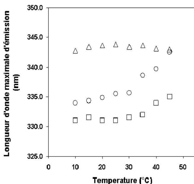
Figure 23. Longueur d'onde maximale d'émission des résidus tryptophanes du LYS ( \Delta ), de l'holo \alpha -LA ( \square ) et de l'apo \alpha -LA ( \circ ) en fonction de la température après excitation à 295 nm. Les spectres étaient acquis pour une concentration protéique de 0.03 g.l -1 dans un tampon 30 mM Tris/HCl (pH 7,5), 15 mM NaCl.
