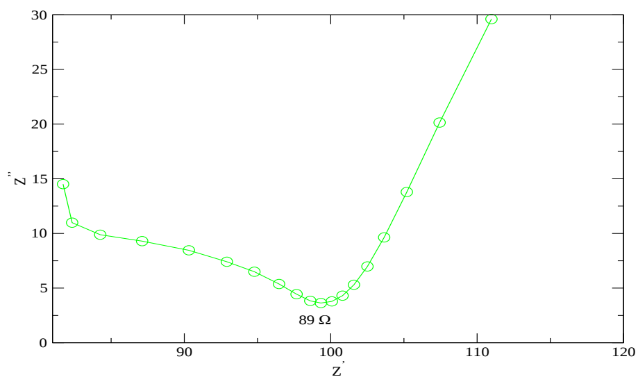
Figure 7.21: Spectre d'impédance de la membrane AW dans la cellule de mercure pour C_T = 0,01N et X_{NO_3^-} = 0,5
