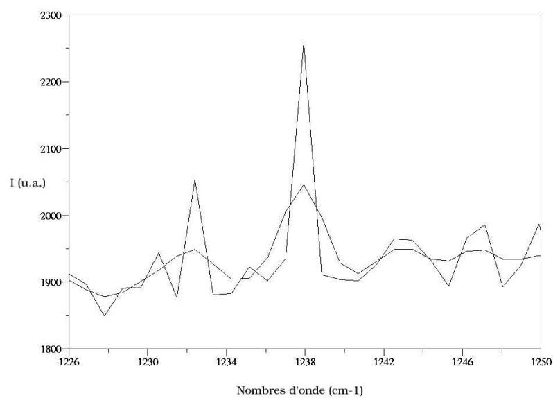
Figure 5.13: Spectre Raman expérimental et spectre Raman corrigé par un filtre gaussien
