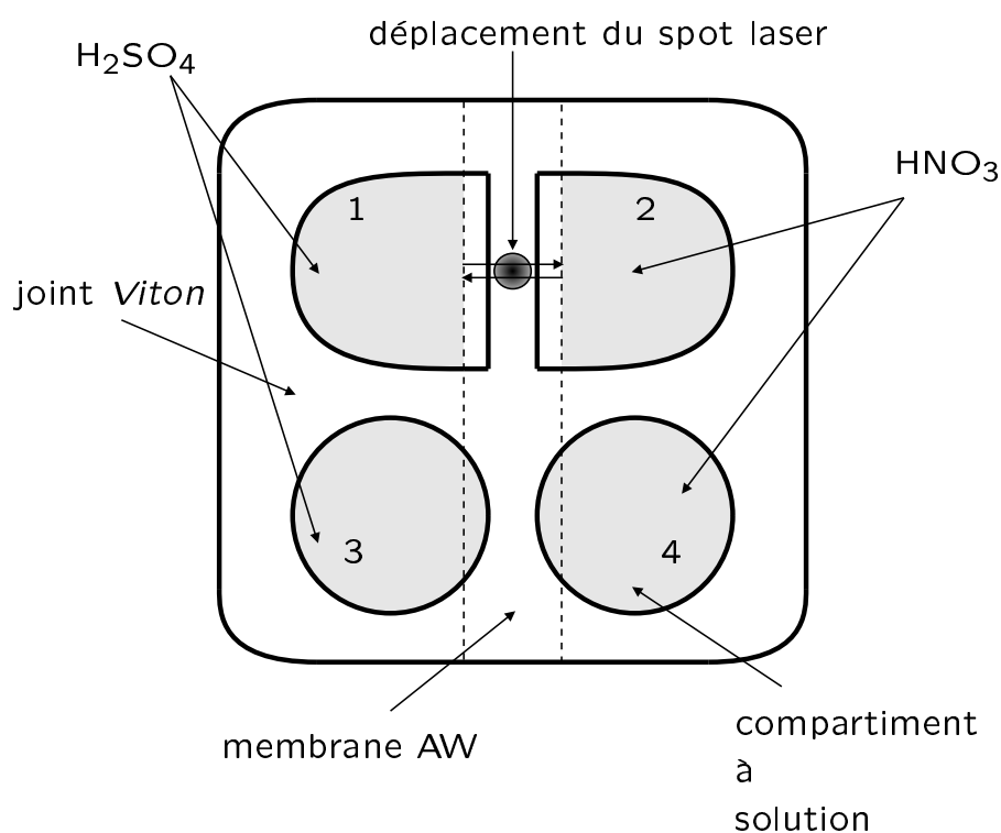
Figure 8.11: Déplacement du spot laser lors d'une cartographie dans le cas d'une dialyse croisée \text{HNO}_3\text{-H}_2\text{SO}_4
