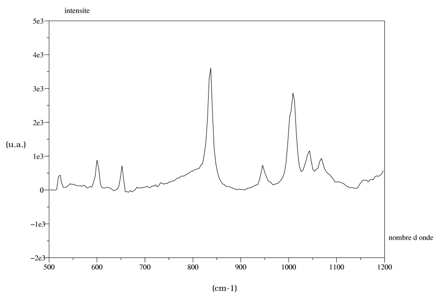
Figure 8.31: Représentation du spectre approchée de la cible de la membrane protonée pure
