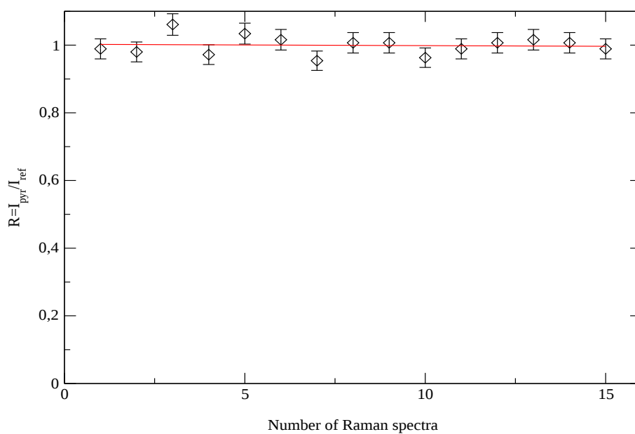
Figure 7.4: Tests d'homogénéité en latéral (coefficient de variation : 3%)
