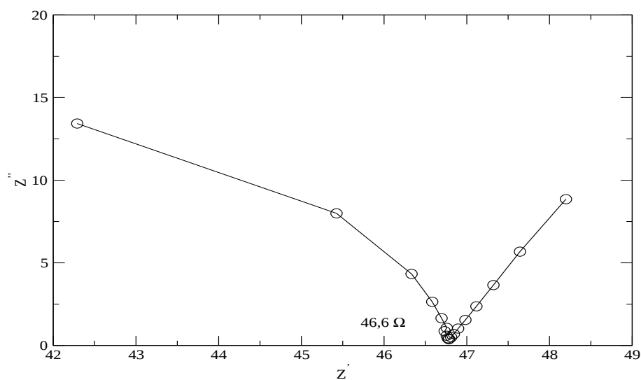
Figure 7.25: Spectre d'impédance de la membrane AW dans la cellule de mercure pour C_T = 0,1\text{N} et X_{NO_3^-} = 0
