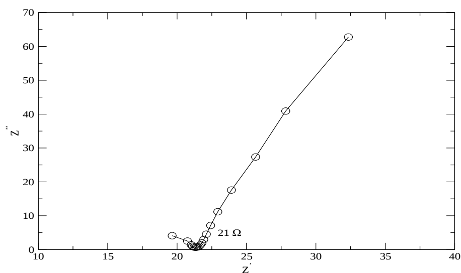
Figure 7.26: Spectre d'impédance de la membrane AW dans la cellule de mercure pour C_T = 0,1\text{N} et X_{NO_3^-} = 1
