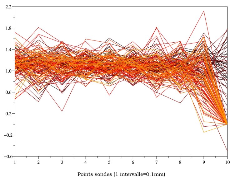
Figure 8.34: Représentation de l'évolution de la concentration pour la membrane à l'état protonée
