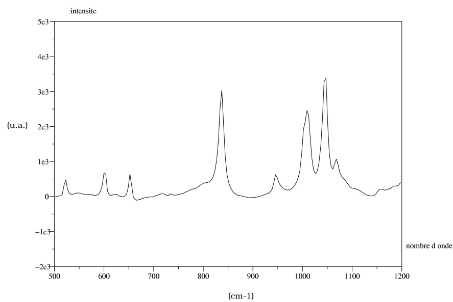
Figure 8.25: Représentation du spectre moyen Raman lors de l'expérience de dialyse croisée \text{HNO}_3\text{-NaCl}
