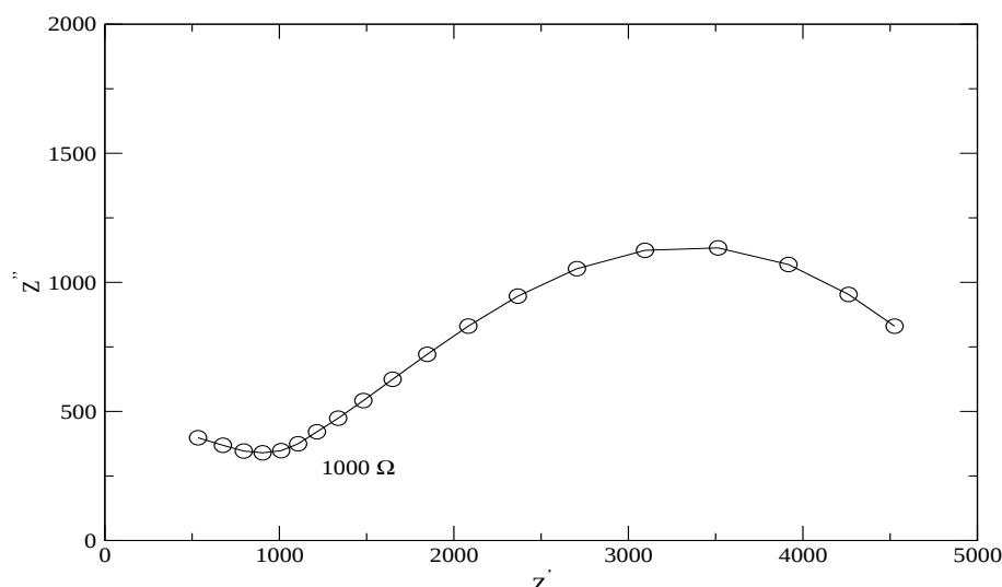
Figure 7.18: Spectre d'impédance de la membrane AW dans la cellule de mercure pour C_T = 0,001N et X_{NO_3^-} = 0,5
