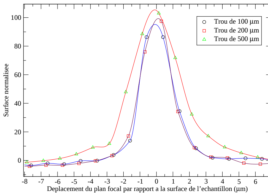
Figure 6.6: Test de confocalité avec l'objectif 100 sur une plaquette de silicium
