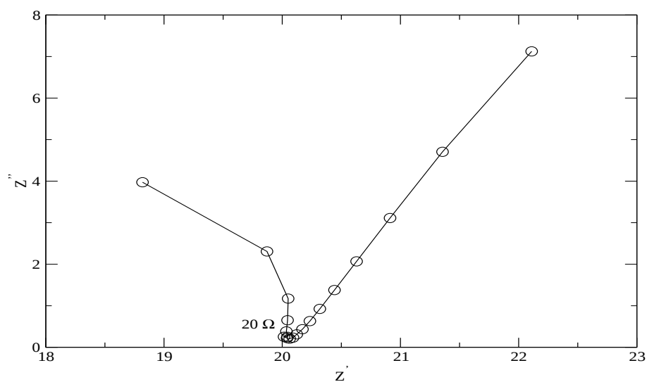
Figure 7.31: Spectre d'impédance de la membrane AW dans la cellule de mercure pour C_T = 1\text{N} et X_{\text{NO}_3^-} = 0
