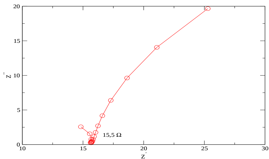
Figure 7.29: Spectre d'impédance de la membrane AW dans la cellule de mercure pour C_T = 0,5N et X_{NO_3^-} = 1
