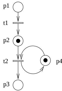
FIG. 4.1: Exemple utilisé de modèle RdP généralisé
