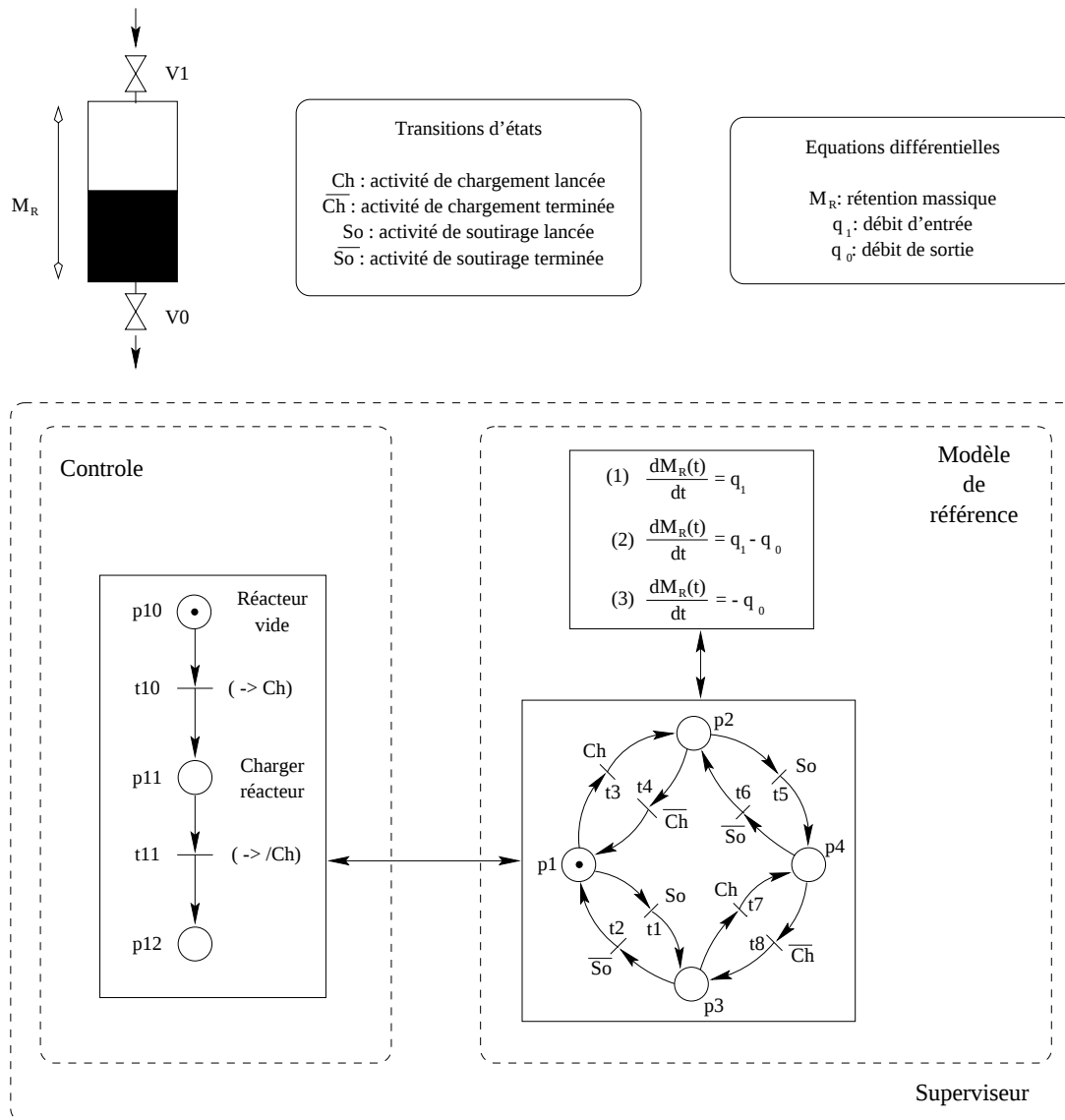
FIG. 5.3: Exemple sur une unité de stockage [Andreu96]
