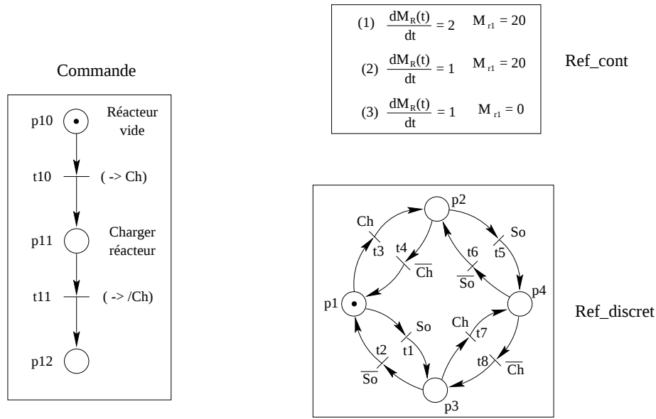
FIG. 5.5: Exemple de validation : une unité de stockage
