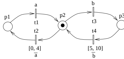
FIG. 5.4: Exemple de rdP temporel à événements
