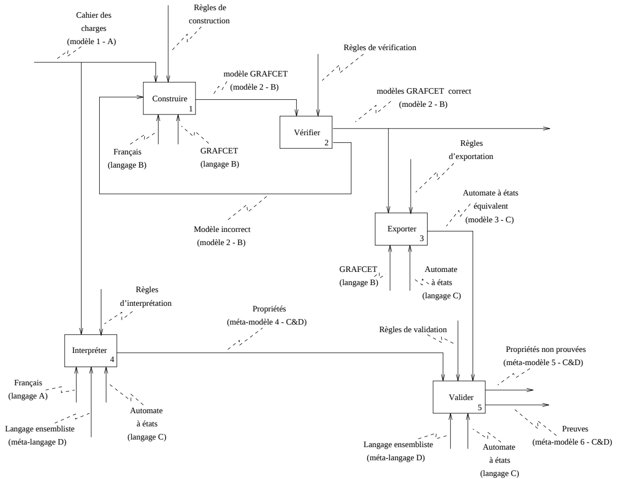
FIG. 2.11: Validation de modèle GRAFCET par automate équivalent
