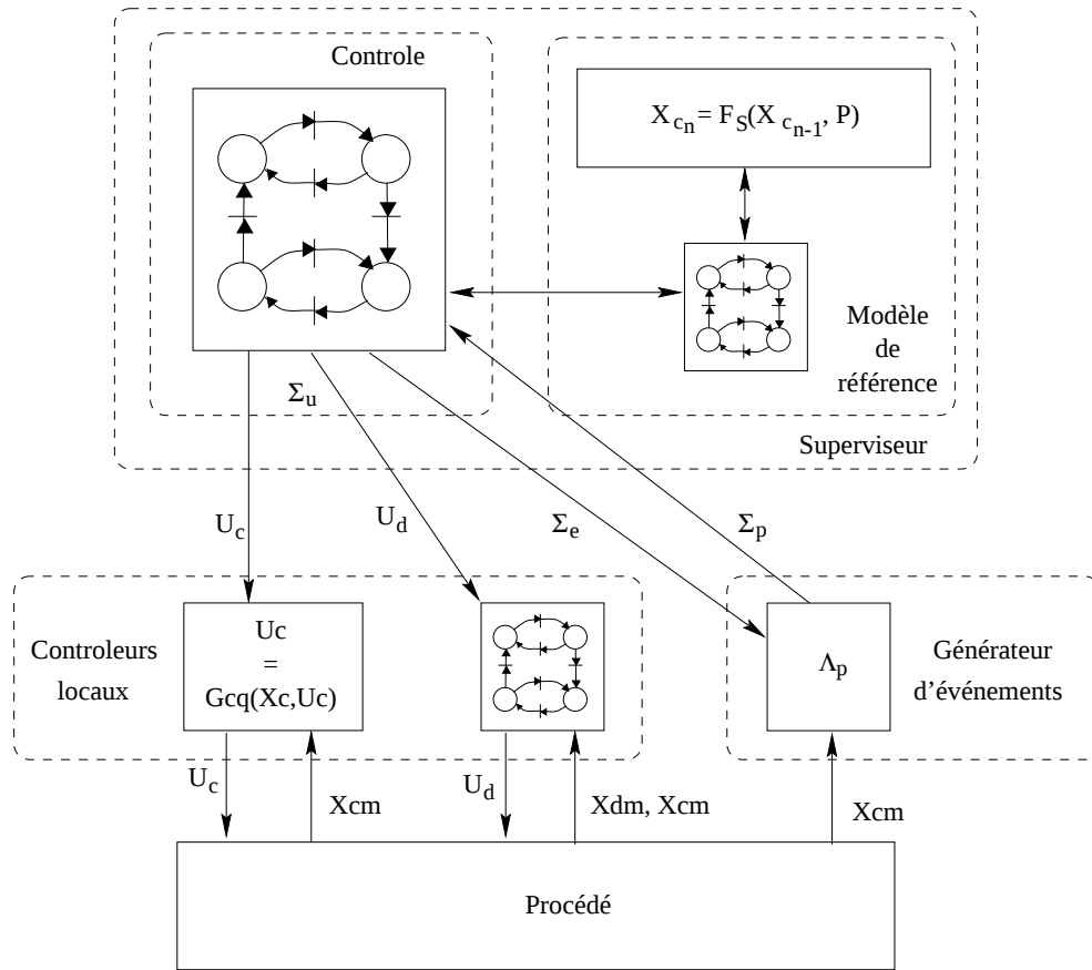
FIG. 5.1: Supervision basée sur un modèle hybride [Andreu96]
