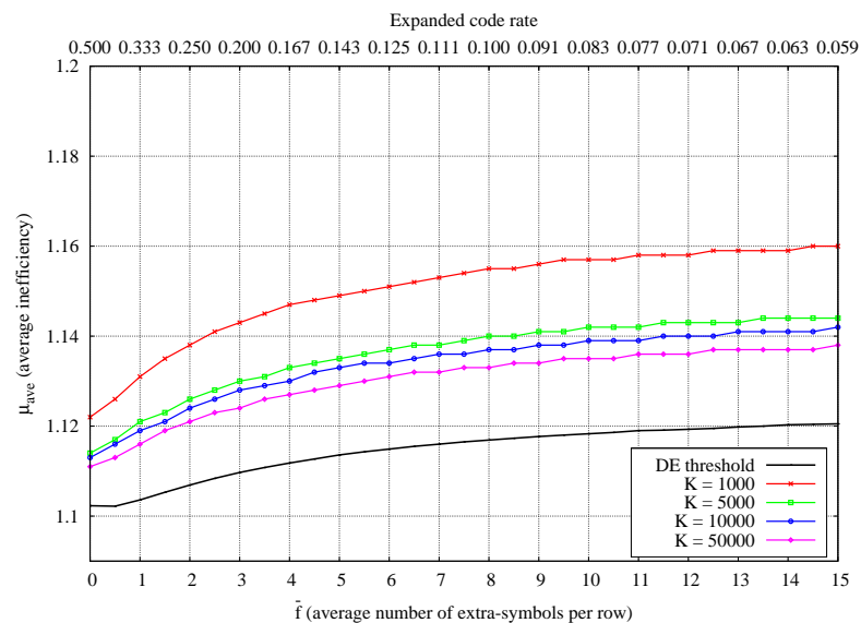
FIG. 8.7 – Inefficacité moyenne en fonction du nombre moyen d'extra-symboles par ligne dans le cas d'une distribution uniforme.
