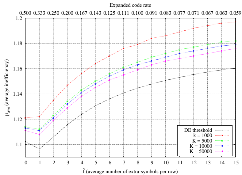
FIG. 8.6 – Inefficacité moyenne en fonction du nombre moyen d'extra-symboles par ligne dans le cas d'une distribution régulière
