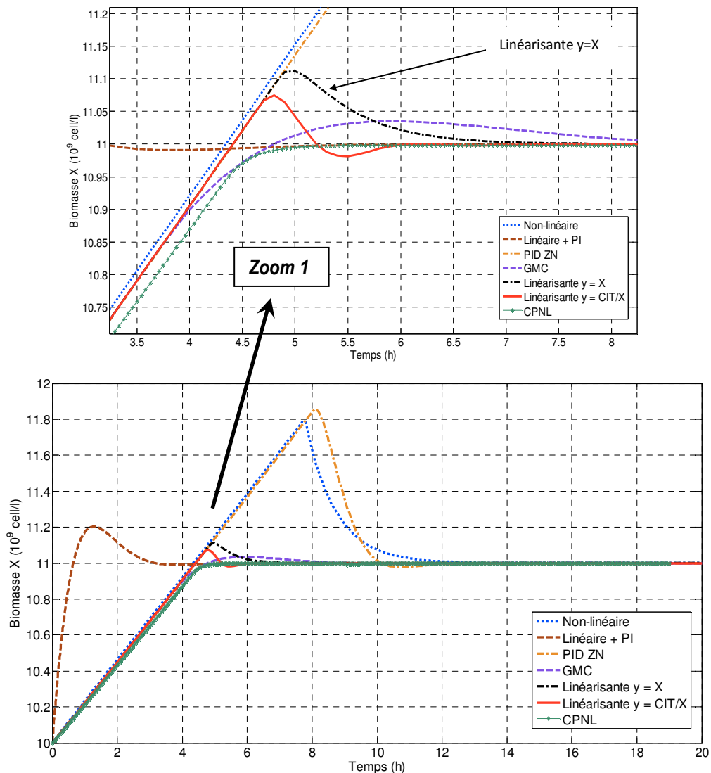
Figure 4.10 : Evolution de la concentration cellulaire pour un échelon sur la consigne (passage de 10 à 11 \cdot 10^9 cellules/l à t = 0 ) avec un zoom.
