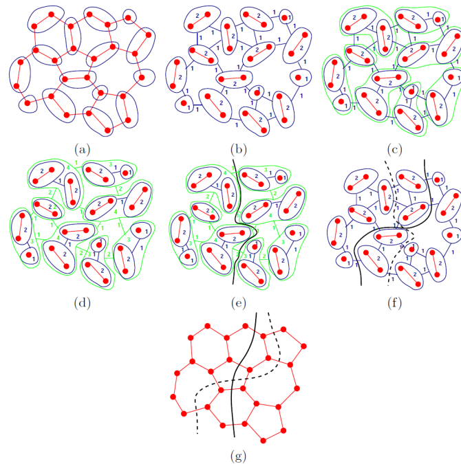
FIG. 7.1: Passage du graphe à sa simplification, partitionnement, puis rétablissement et affinage du partitionnement.
