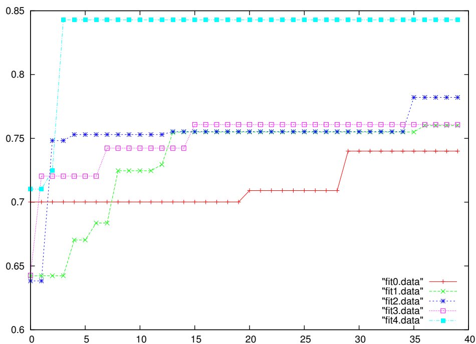
FIG. 10.1: Évolution de la valeur pbest pour cinq particules sur un graphe en grille 5 \times 8 .
