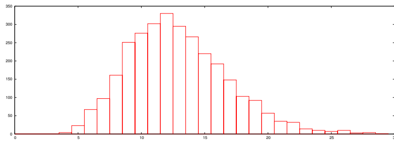
FIG. 11.5: Distribution de degrés des sommets d'un graphe aléatoire de 3000 sommets.
