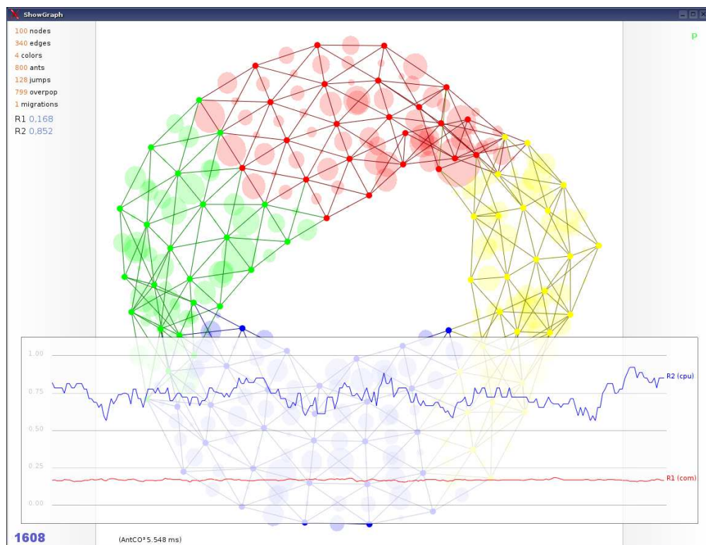
FIG. 13.6: Capture d'écran de la seconde implantation du modèle sur le graphe «mœbius».
