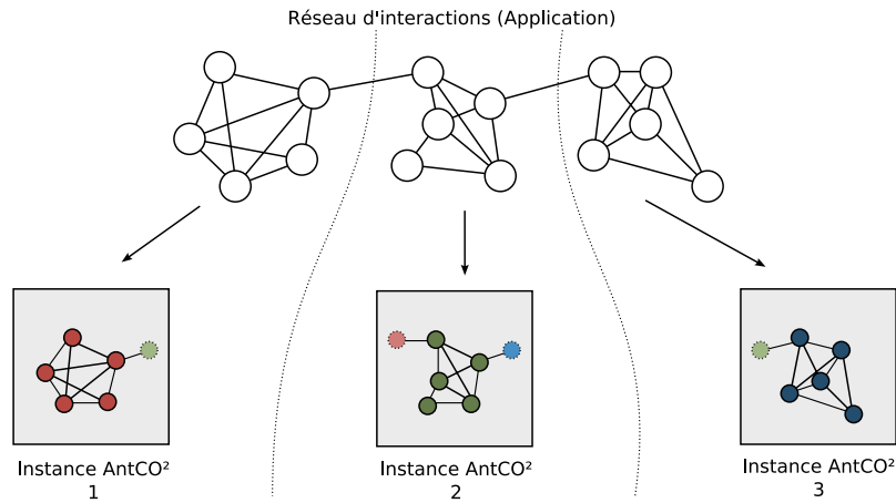
FIG. 9.9: Découpage et recouvrement du graphe sur les différentes instances d' AntCO 2 .
