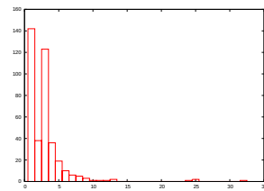
(c) Distribution de degrés.
