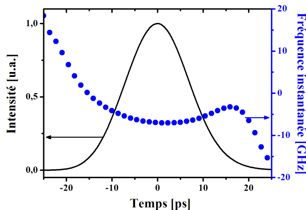
FIG. 4.25 – Fréquence instantanée et enveloppe temporelle obtenue par la mesure à l'analyseur optique de spectre complexe. La variation de la fréquence instantanée est très faible aux alentours du pic d'intensité.
