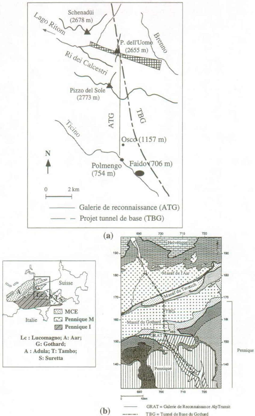
Figure 3.12 : Plan de situation (a) et contexte tectonique (b) de la galerie de reconnaissance AlpTransit Gothard (ATG) de Polmengo [d'après Schneider 1993].
