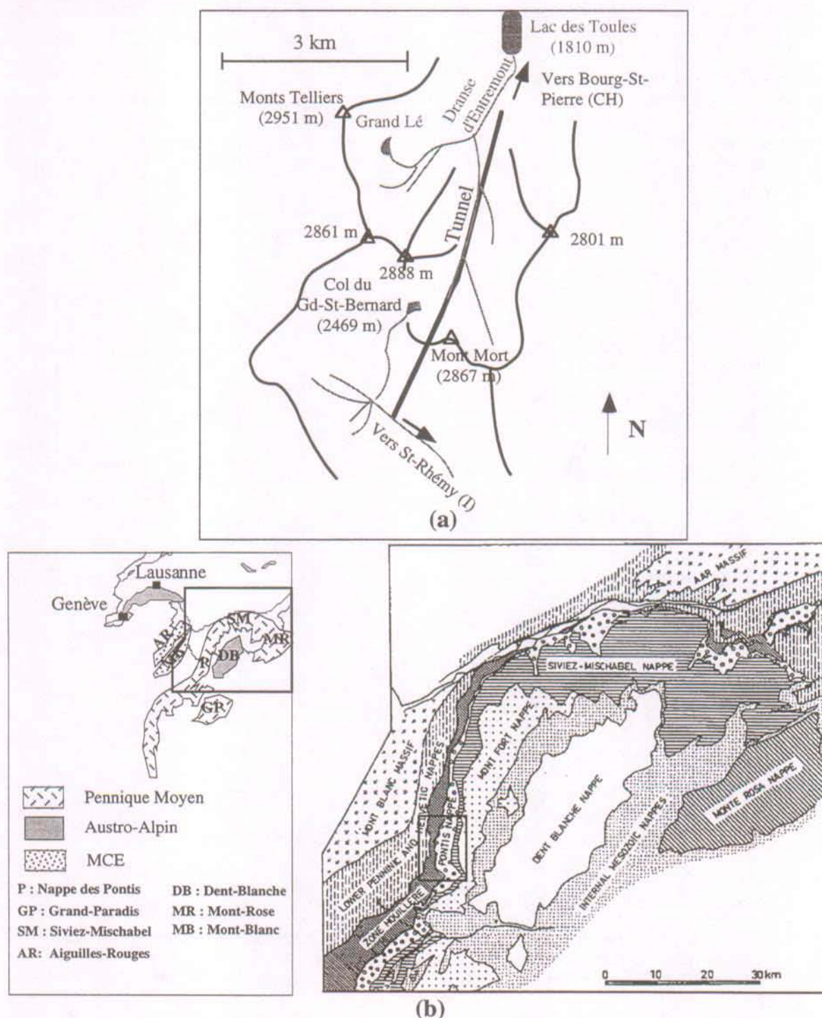
Figure 3.6 : Plan de situation (a) et contexte tectonique (b) du tunnel routier du Gd-St-Bernard [d'après Thélin et al. 1993].
