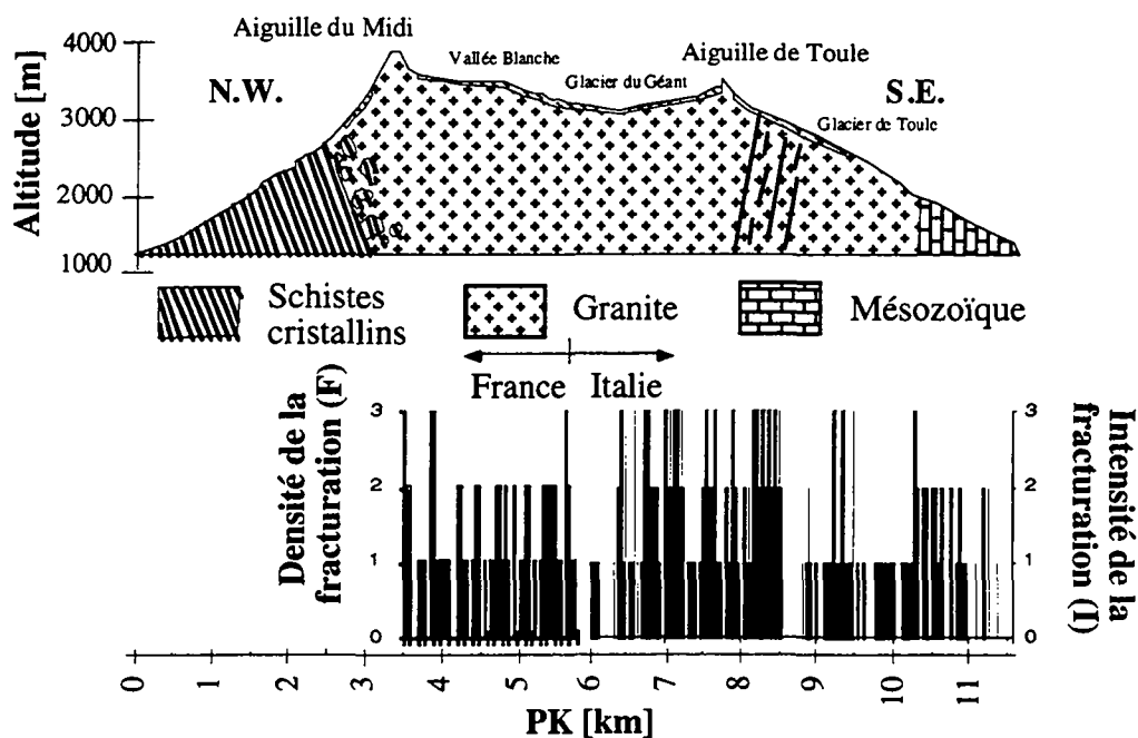
Figure 4.3 : (a) Coupe géologique du tunnel routier du Mont-Blanc. Trois unités principales se distinguent.
