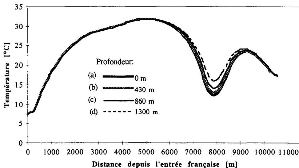
Figure 7.12 : Effet de l'extension en profondeur [m] de la zone tectonisée sur les températures calculées en 1960.
