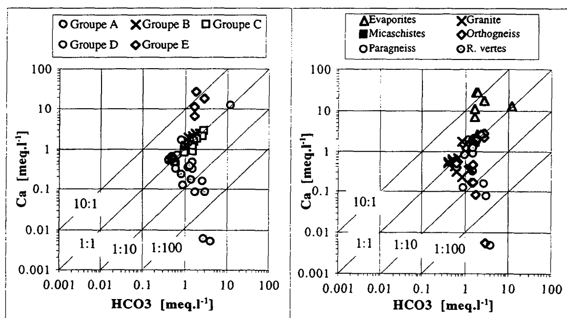
Figure 6.19 : Rapport entre Ca et \text{HCO}_3 pour les différents groupes chimiques (a) et les diverses pétrographies (b).
