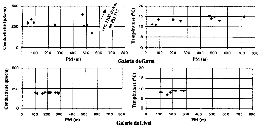
Figure 4.21 : Profils des conductivités électriques et températures des venues d'eau dans les galeries de Livet et de Gavet.
