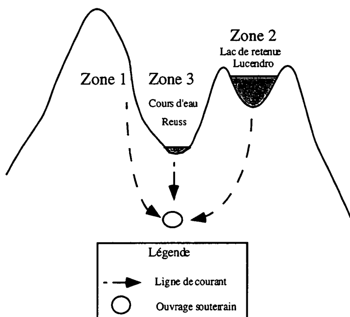
Figure 4.43 : Représentation schématique des trois zones d'anomalies isotopiques.
