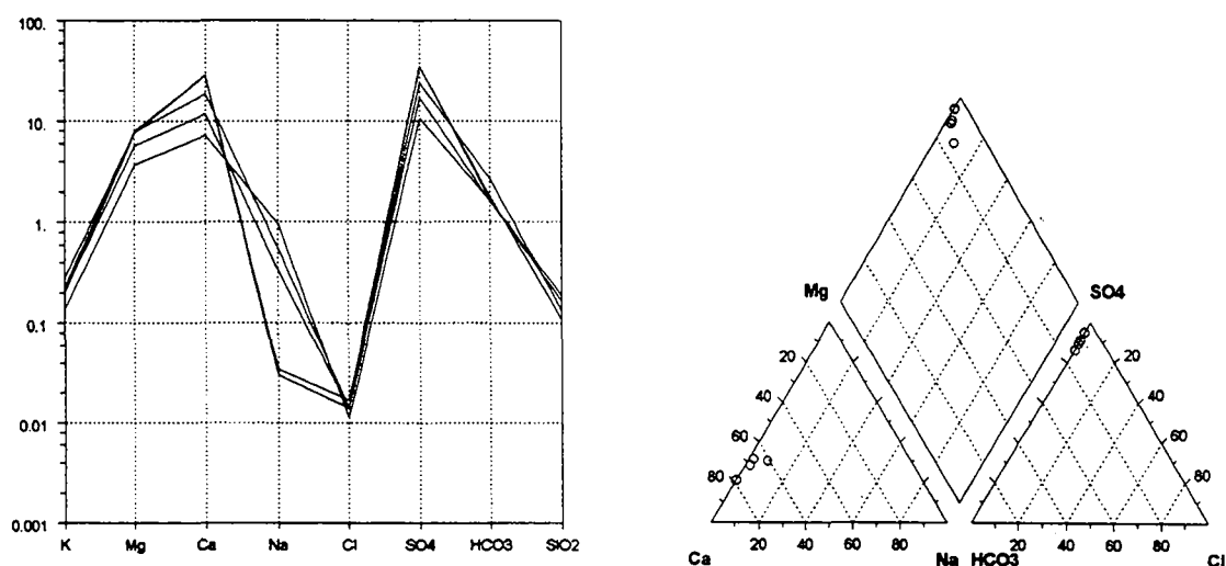
Figure 6.16 : Représentation sur diagrammes de Schoeller et Piper des eaux du groupe E.
