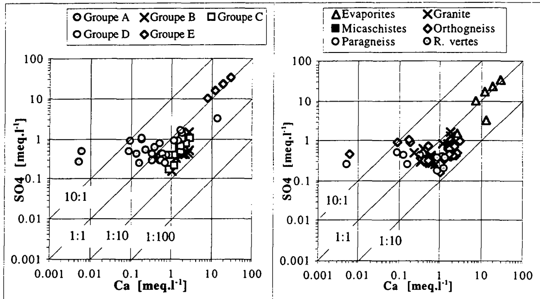
Figure 6.25 : Rapport entre \text{SO}_4 et Ca pour les différents groupes chimiques (a) et les diverses pétrographies (b).
