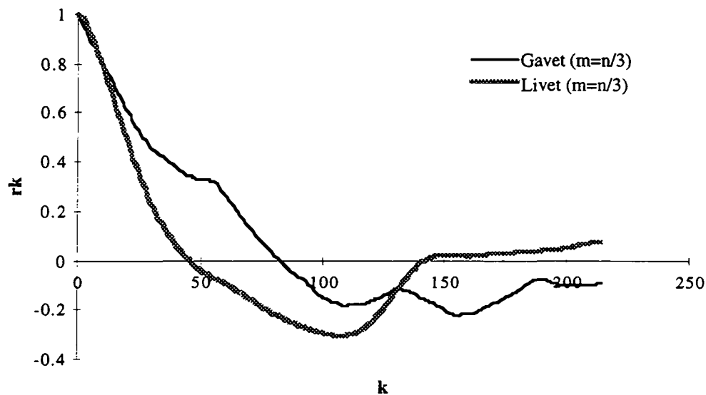
Figure 6.69 : Autocorrélogrammes des débits à Livet (du 27 avril 1995 au 17 septembre 1997) et Gavet (du 23 novembre 1995 au 27 août 1997).
