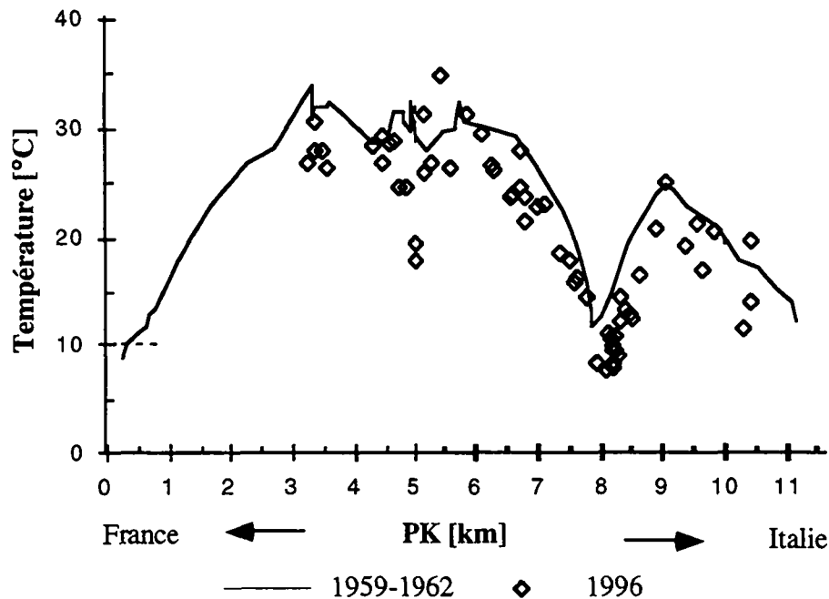
Figure 4.6 : Profils de températures des venues d'eau dans le tunnel du Mont-Blanc. Traits pleins : mesures effectuées dès le percement (1959-1962). Losanges : mesures effectuées en 1996. Une forte anomalie de températures apparaît sur les deux profils au PK 8,0-F. En 1996, une seconde anomalie apparaît au PK 5,0-F.
