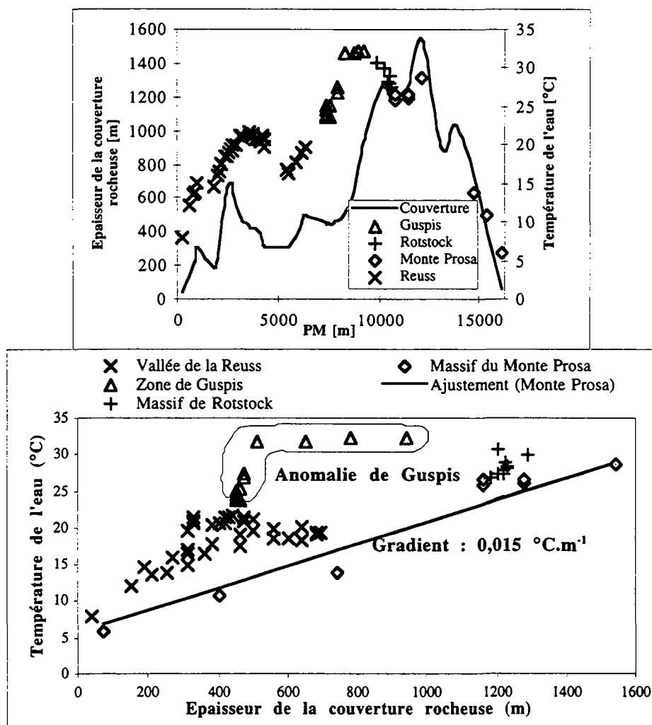
Figure 6.77 : Cas du Gothard N2. Profil des températures des venues d'eau et de la couverture rocheuse (a). Evolution de la température de l'eau en fonction de la couverture rocheuse (b).
