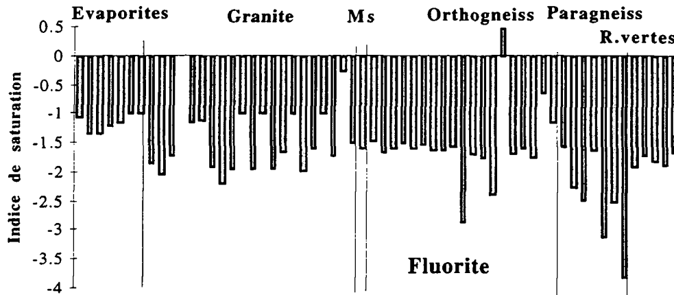
Figure 6.35 : Indices de saturation des eaux par rapport à la fluorine.
