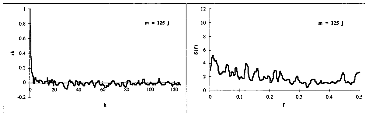
Figure 6.68 : Autocorrélogramme et spectre de densité des précipitations à la station de Livet entre le 1er février 1995 et le 22 septembre 1997 ( m = 125 jours).
