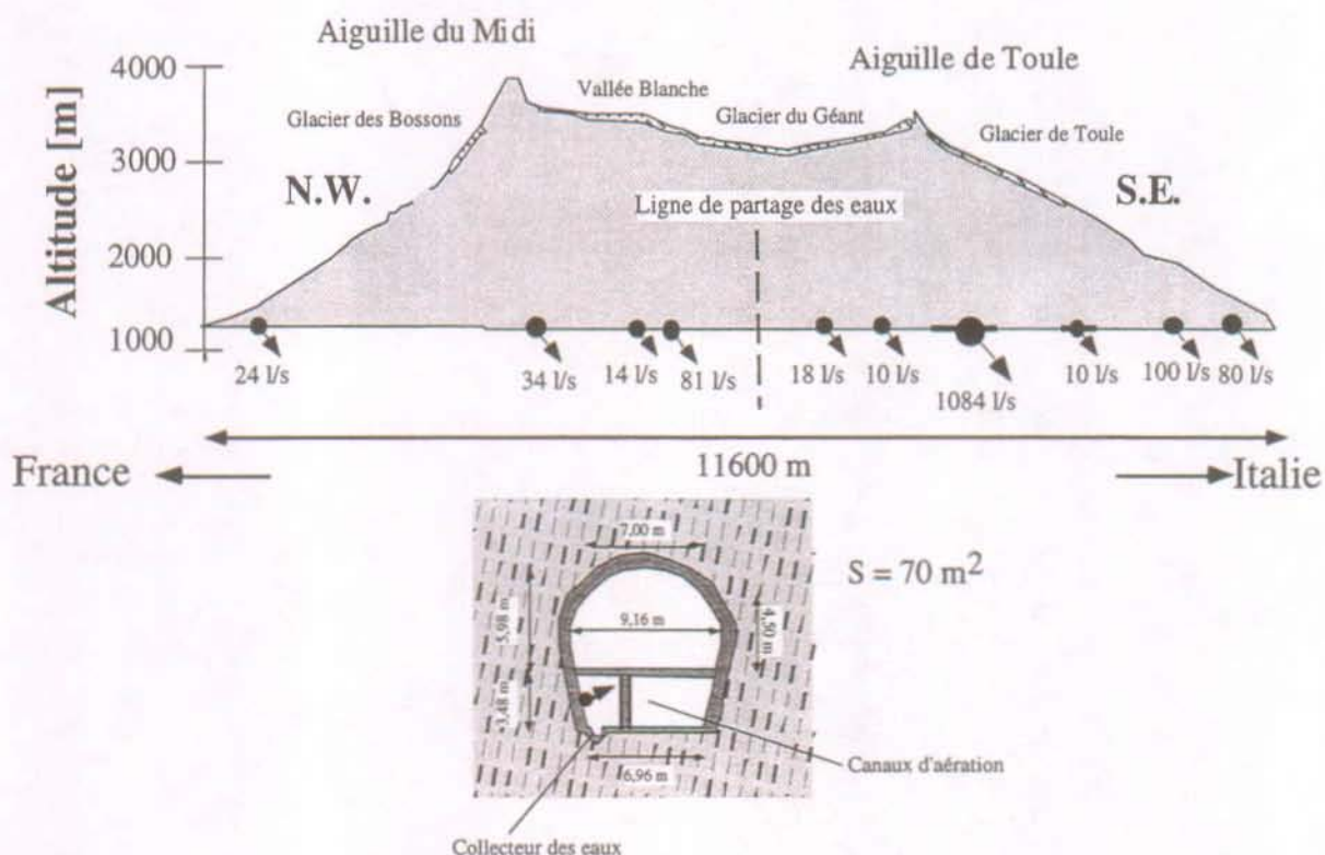
Figure 3.5 : Coupe du tunnel routier du Mont-Blanc. Les venues d'eau indiquées ont été mesurées à l'avancement [Gudefin 1967].
