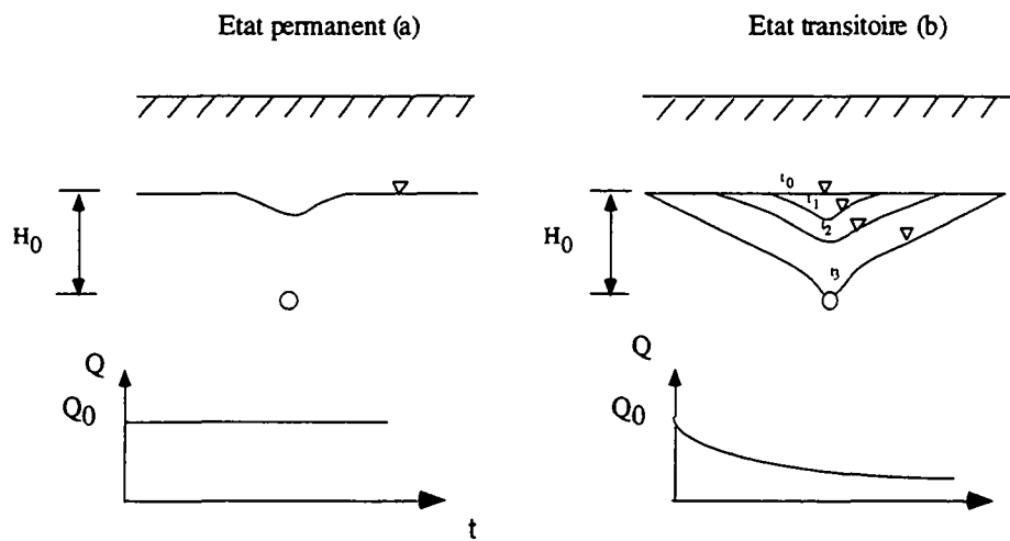
Figure 5.4 : Interactions entre un ouvrage souterrain et une nappe d'eau souterraine. Cas permanent d'un ancien ouvrage (a) et cas transitoire d'un ouvrage récent (b). D'après Freeze et Cherry [1979].
