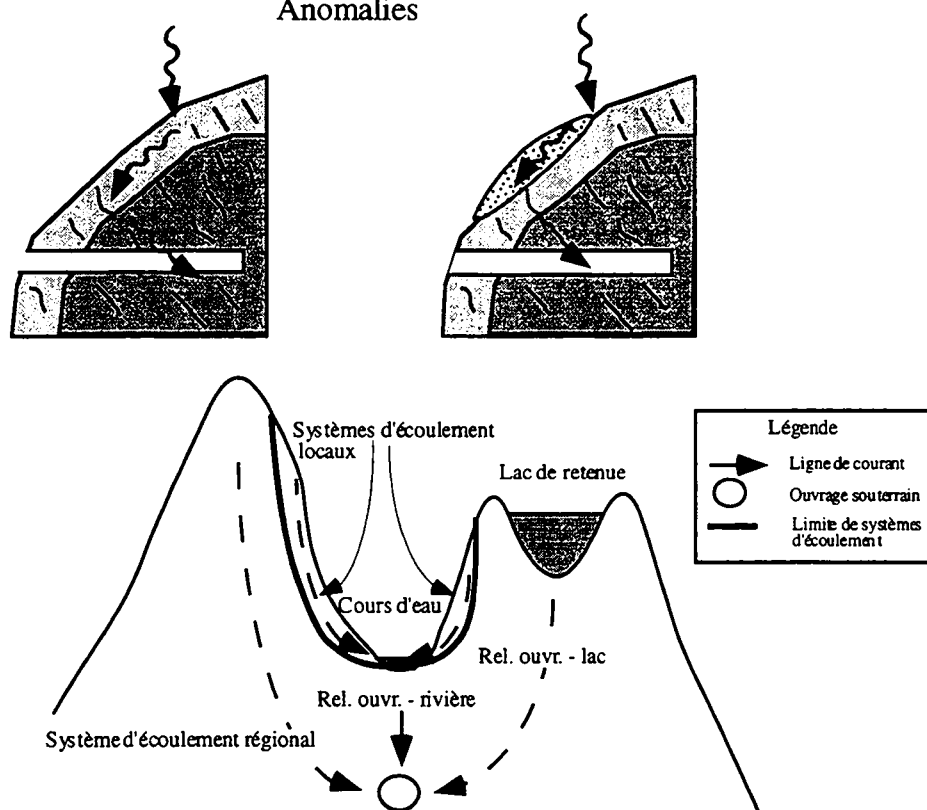
Figure 6.103 : Modèles d'écoulement entre les zones d'alimentation et les tunnels alpins.
