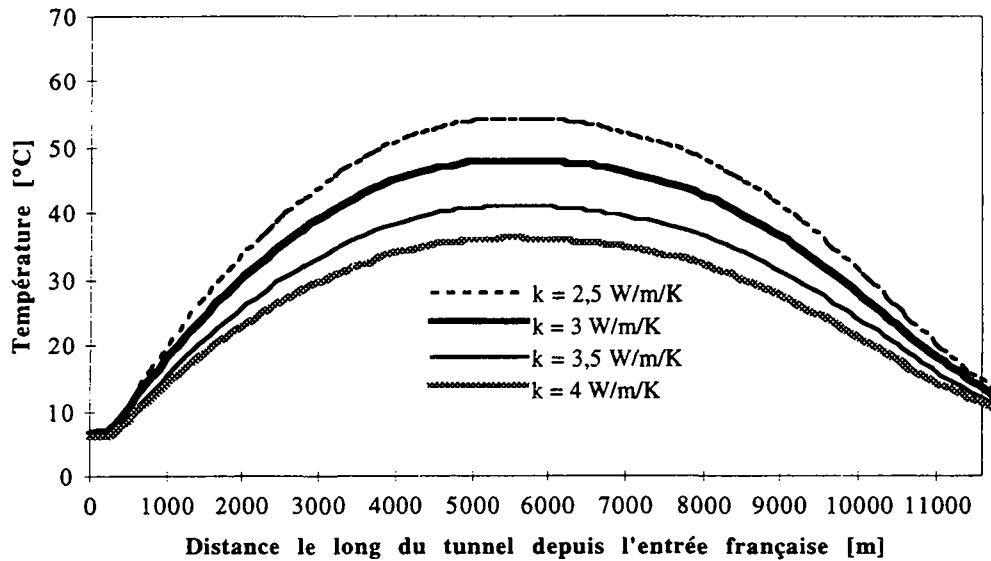
Figure 7.4 : Sensibilité des températures calculées à la conductivité thermique des terrains [ \text{W.m}^{-1}.\text{K}^{-1} ].
