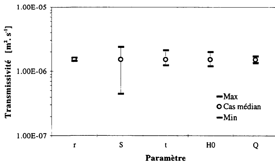
Figure 5.11 : Variations des transmissivités calculées en fonction des incertitudes sur les différents termes de la relation de Jacob et Lohman en état transitoire.
