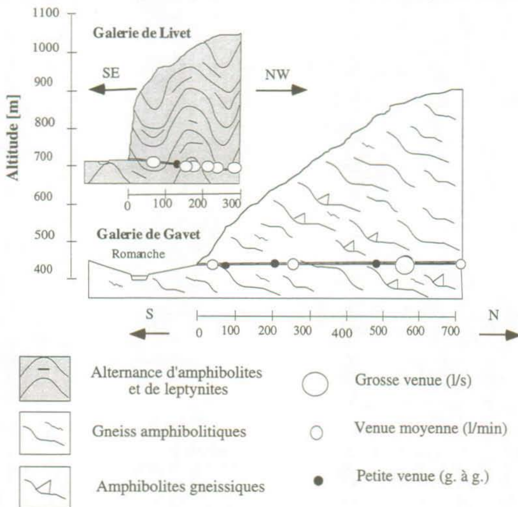
Figure 4.19 : Coupes géologiques schématisiques des deux galeries de Livet et Gavet et localisation des principales venues d'eau.
