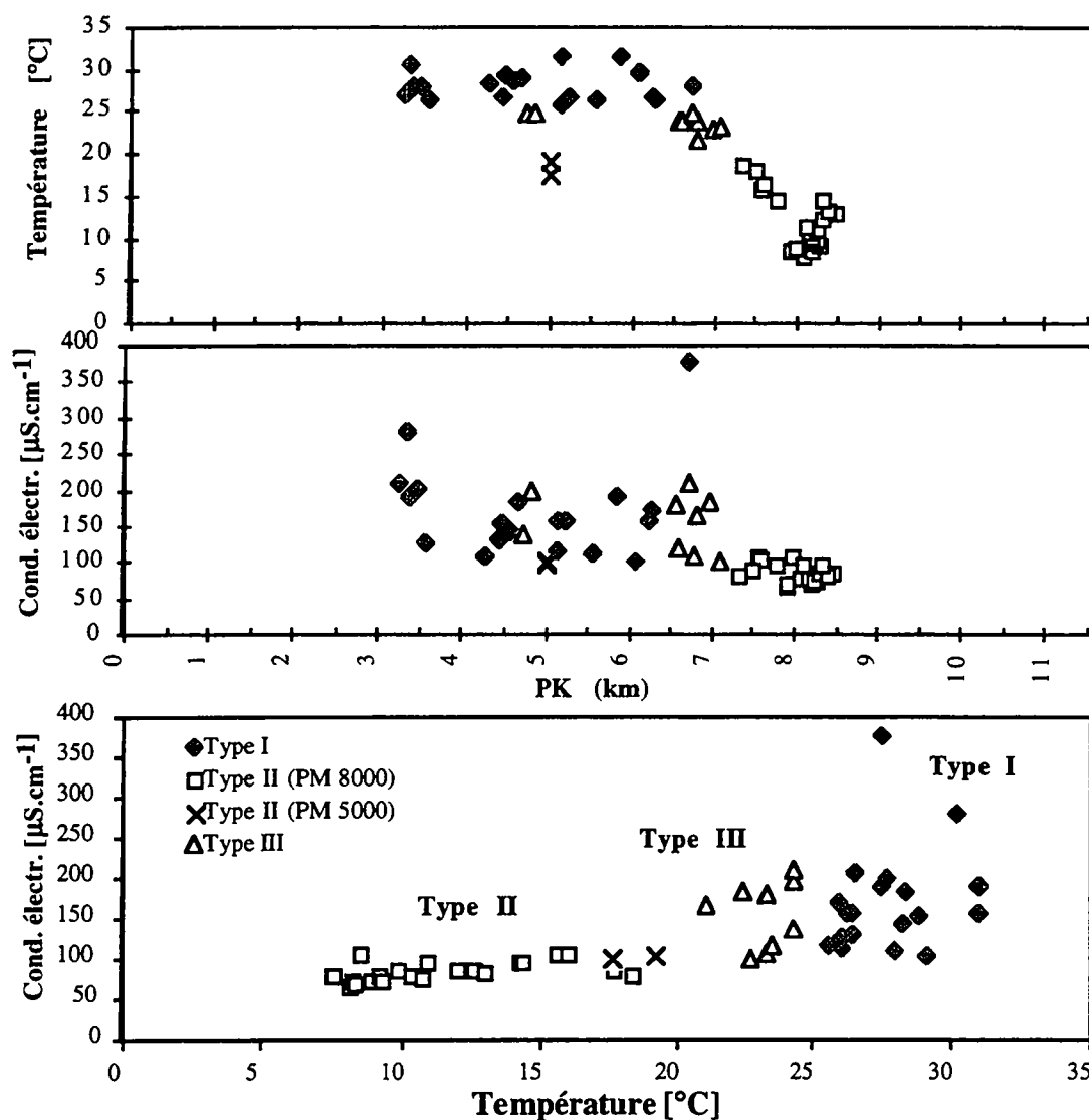
Figure 4.8 : Profils des températures et conductivités électriques des venues d'eau dans la partie centrale du granite du Mont-Blanc. Mesures effectuées le 26 janvier 1996. Diagramme de la conductivité électrique corrigée à 20°C en fonction de la température.
