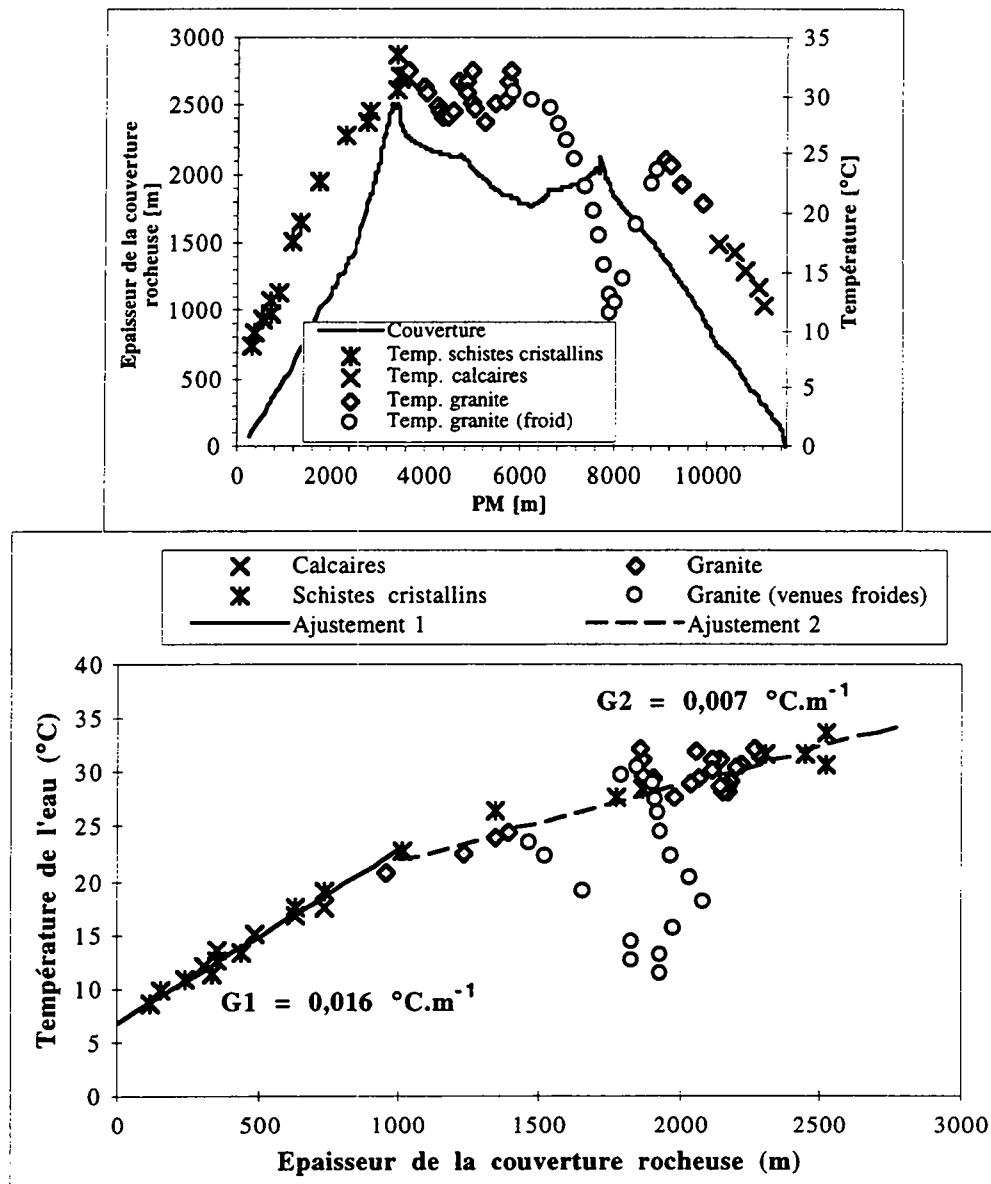
Figure 6.76 : Cas du Mont-Blanc. Profil des températures des venues d'eau et de la couverture rocheuse (a). Evolution de la température de l'eau en fonction de la couverture rocheuse (b).
