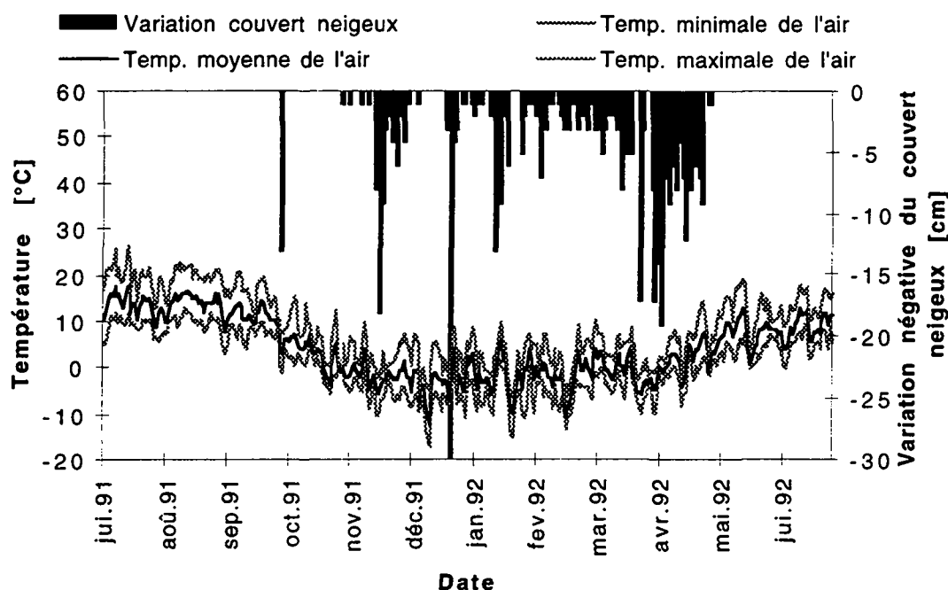
Figure 6.97 : Evolution des variations négatives de l'épaisseur du couvert neigeux et des températures horaires moyennes, minimales et maximales de l'air à la station météorologique du San Bernardino (91-92).
