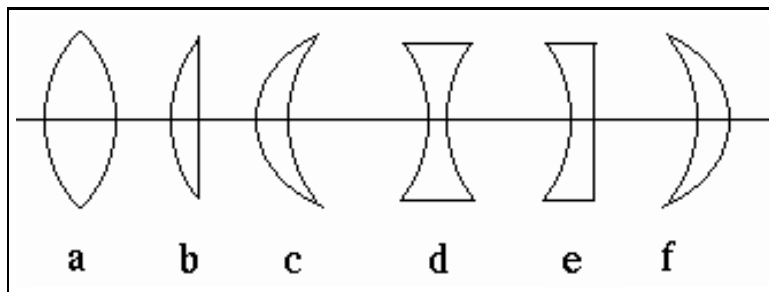
FIG. 1.6 – (a): bi-convexe, (b): plan-convexe, (c): ménisque positif, (d): bi-concave, (e): plan-concave, (f): ménisque négatif
