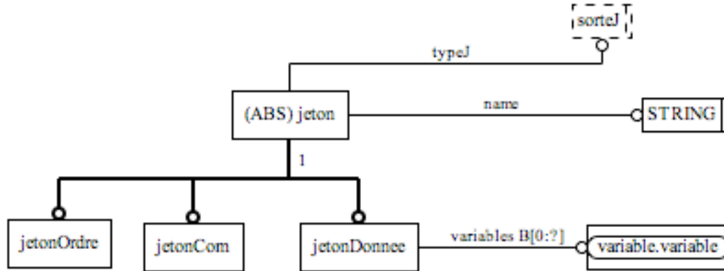
Figure 5.2.2 : Schéma EXPRESS-G de l'entité jeton
