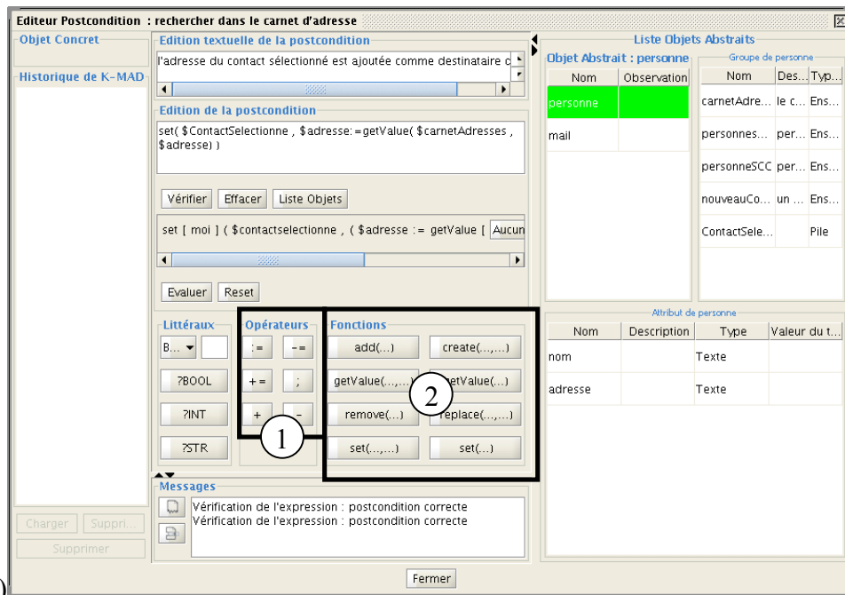
Figure 4.1.6 : Les calculettes de a) pré et b) post-conditions
