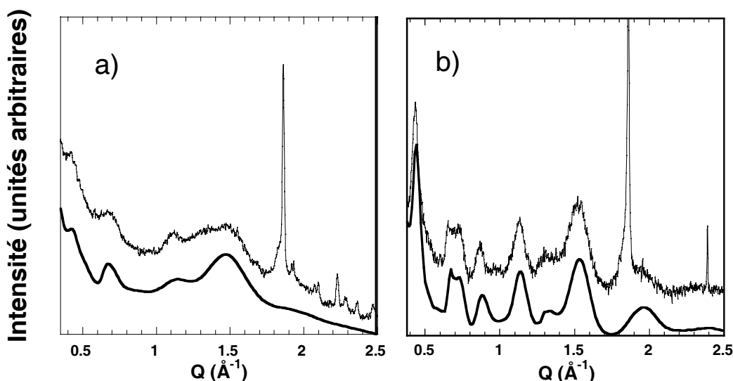
FIG. 2.29: a ) Diffractogramme expérimental de l'échantillon de peapods fabriqué à Strasbourg (haut), ainsi qu'un calcul de l'intensité diffractée (bas). b ) Idem pour l'échantillon de peapods fabriqué à Tokyo. Voir le texte pour le détail des paramètres utilisés lors des calculs.
