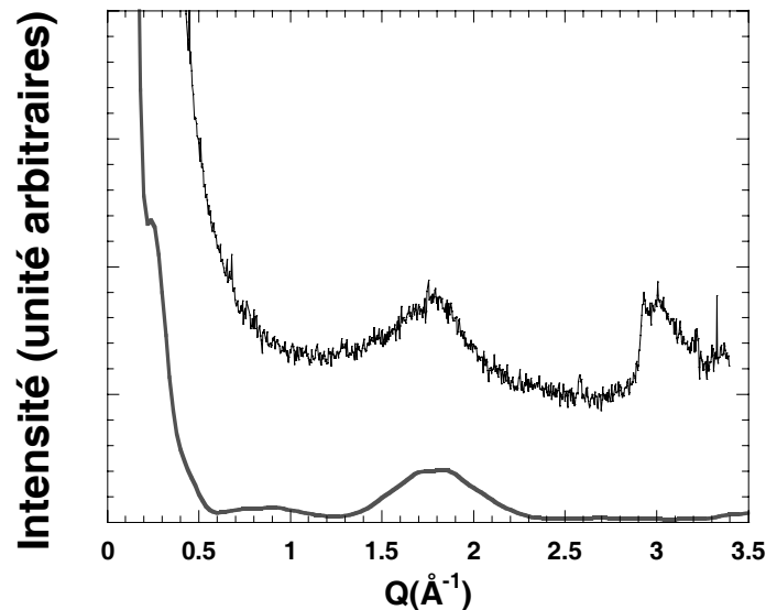
FIG. 2.15: Haut : Diffractogramme neutrons d'un échantillon de DWNT produit par CCVD. Bas : Simulation du diagramme de diffraction d'un échantillon contenant un mélange de nanotubes à 1, 2, 3 et 4 parois (voir le texte pour le détail de la composition).
