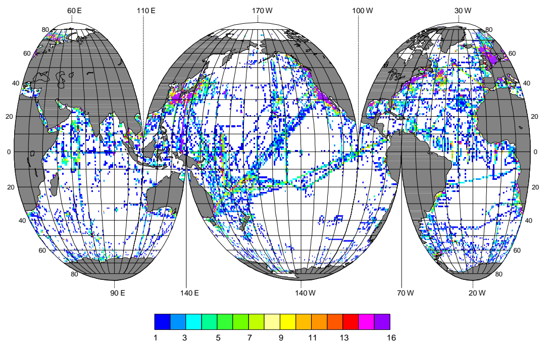
Figure 28 : Nombre de mesures bateau dans des pavés de 1°x1° utilisées pour construire la climatologie de Levitus (WOA, 1998). Number of ship measurements in 1°x1° rasters used to built the Levitus climatology.
