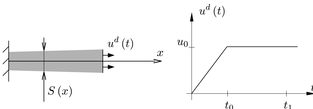
Figure 4.4 – Problème poutre
