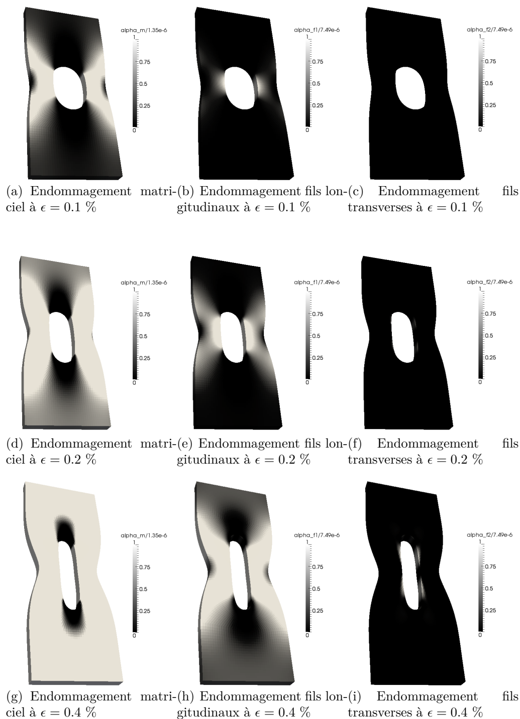
Figure 4.43 – Calcul d'une plaque trouée dans LMT++ : champs d'endommagement adimensionnés pour différents niveaux de déformation imposée
