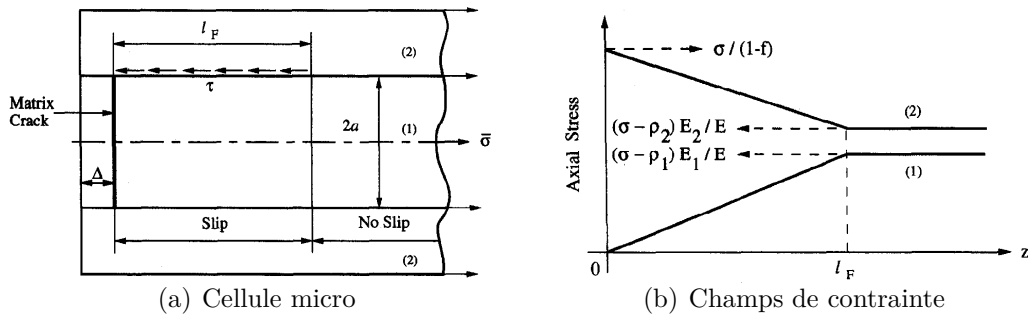
Figure 2.9 – Cellule micro fissurée et champs de contrainte associés [Hild et al. , 1996a]
