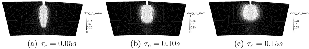
Figure 4.28 – Localisation contrôlée : influence de l'effet retard (Champs d'endommagement) ( n_{ddls} = 1500 , t_0 = 1s )
