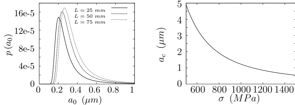
(a) Distributions des tailles initiales des défauts : effets d'échelles (b) Taille critique des défauts en fonction de la contrainte appliquée
