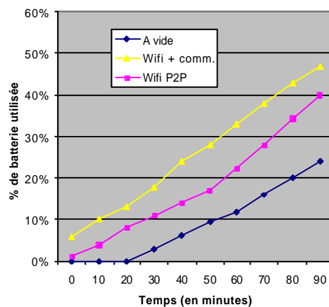
Figure 4.10. Evolution de la consommation d'énergie en fonction du temps
