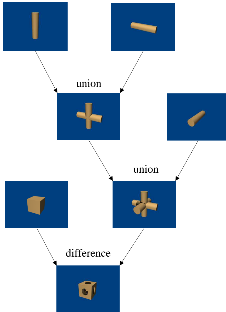
Figure 2.1 — Exemple d'arbre constructif avec les primitives dans les feuilles et les opérations dans les noeuds de l'arbre.
