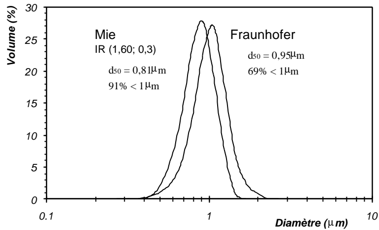
figure 3.31 – Granularités d'un polymère (latex), dont le diamètre moyen garanti est de 0,81 μm. Calculs effectués avec la théorie de Mie et l'approximation de Fraunhofer.
