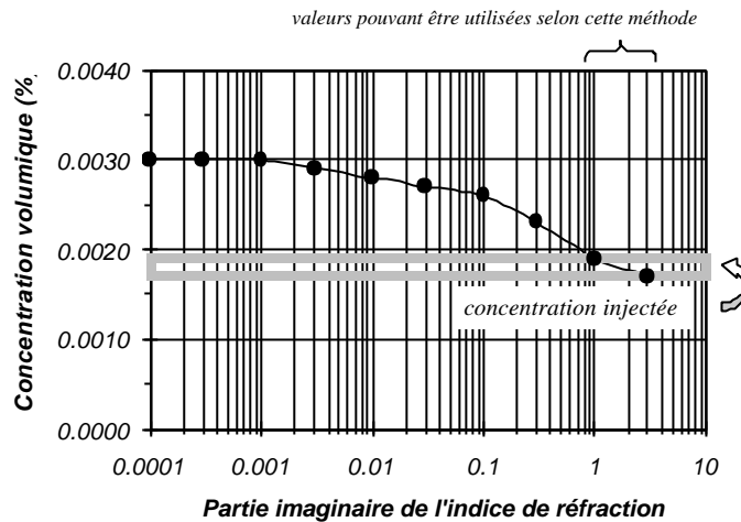
figure 3.36 – Application de la méthode obscuracion-concentration pour la mesure de la partie imaginaire de l'indice de réfraction d'un quartz broyé. Pour les particules de forme irrégulière, la méthode ne donne pas des résultats réalistes.
