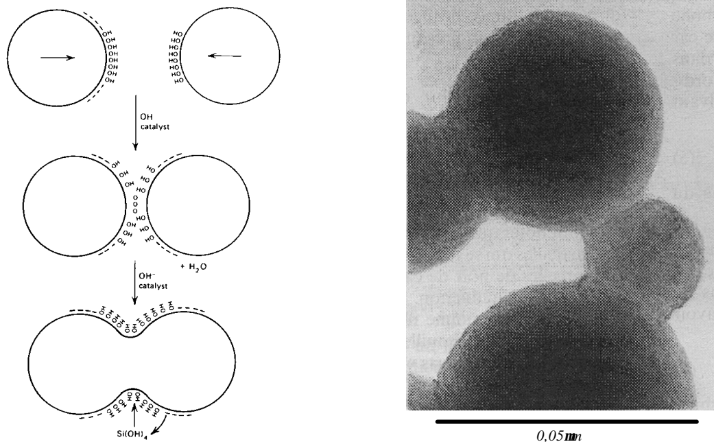
(a) formation d'un lien siloxane, catalysé par une base ( \text{OH}^- ) (b) agglomérat de particules élémentaires [Dubrous (1990)]. [Iler (1979)]
