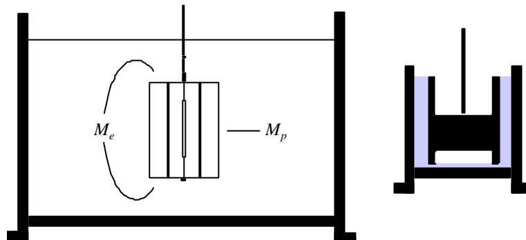
figure 5.10 – Comparaison des montages mobile à ailettes – cylindres coaxiaux.
