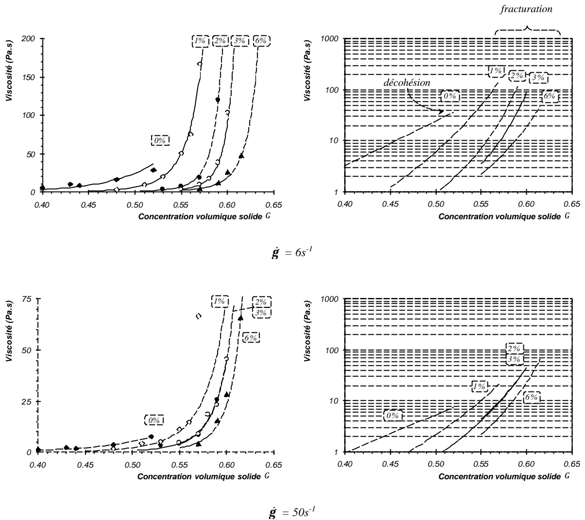
figure 7.13 – Viscosités apparentes, calculées à faible et fort taux de cisaillement ( 6 et 50s^{-1} ), de pâtes de ciment fluidifiées (SPI), en fonction de la concentration solide volumique. Les courbes de régression suivent la relation de Krieger-Dougherty (1959).
