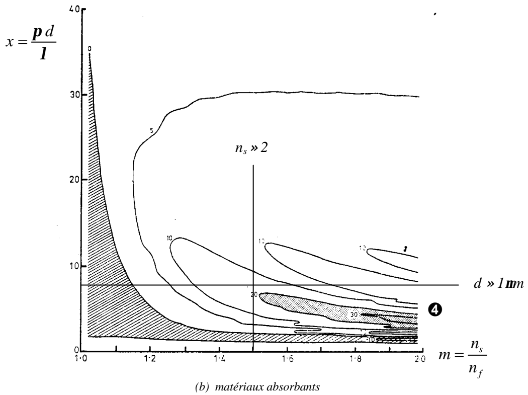
figure 3.25 - Erreurs relatives sur le calcul de l'intensité diffusée entre la théorie de Mie et l'approximation de Fraunhofer, en fonction du paramètre de taille des particules ( x ) et du rapport des indices de réfraction (parties réelles) entre le matériau et le fluide porteur. Les régions ombragées donnent les erreurs supérieures à 20%. [d'après Jones (1977)]
