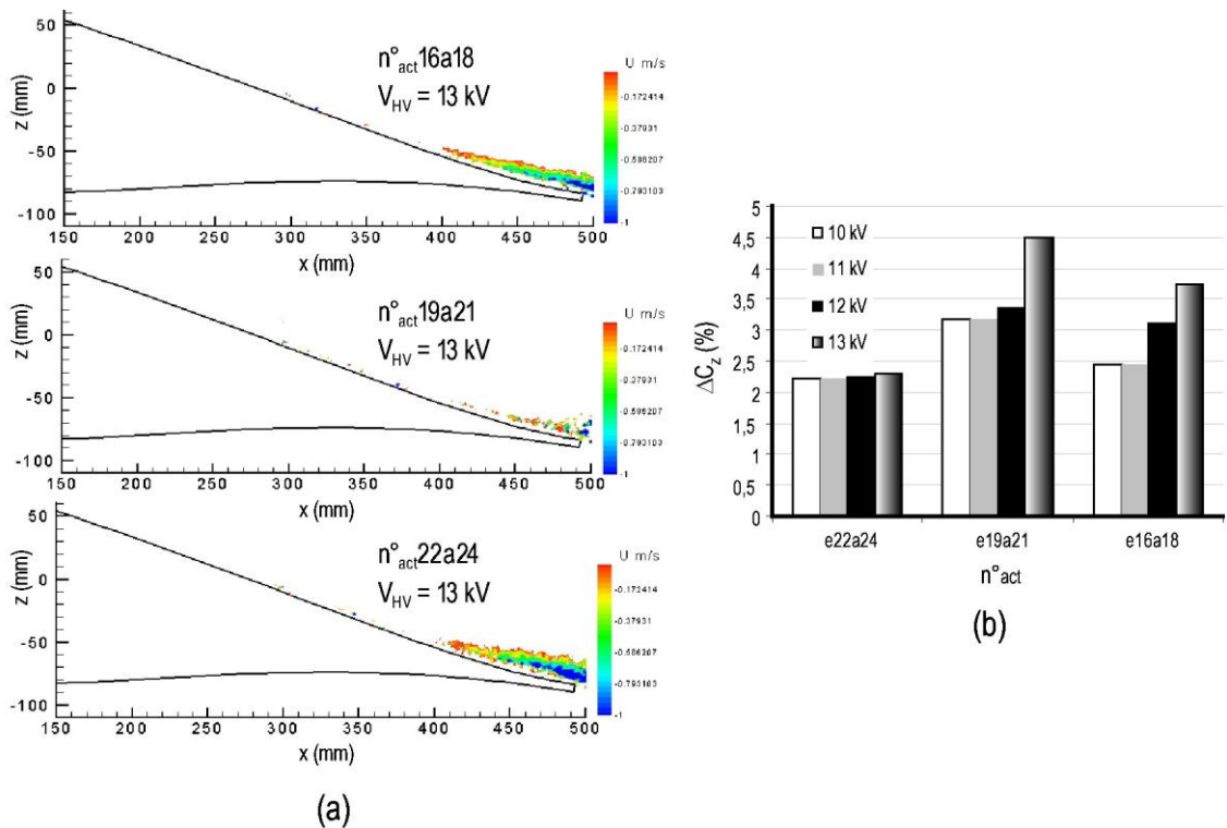
u e la position des actionneurs sur (a) la taille de la zone de recirculation et sur (b) le gain en portance ( \alpha_i = 10^{\circ} , U_{\infty} = 10 m/s)
