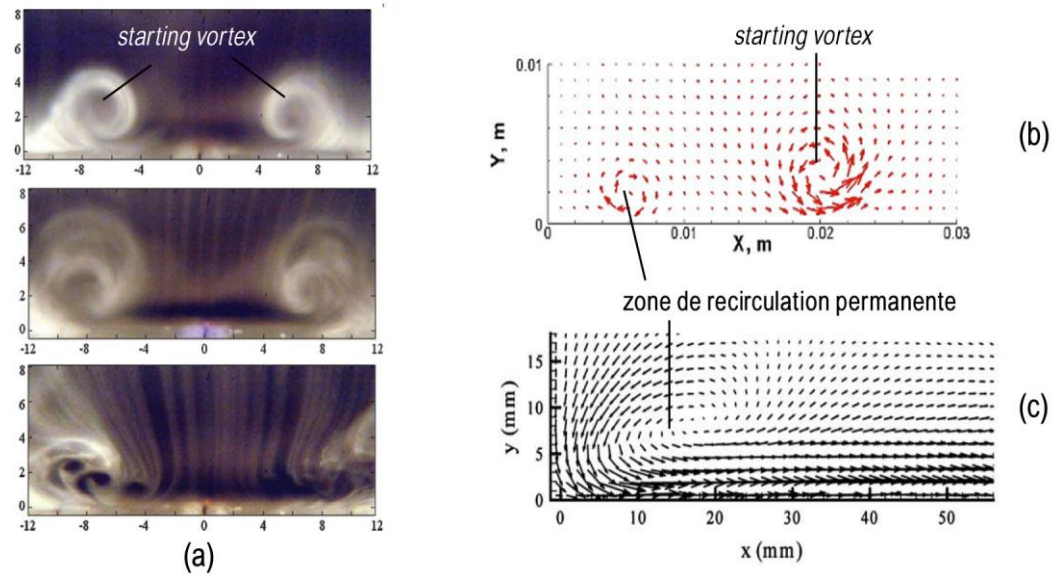
Figure 1.18 – (a) Visualisation du starting vortex par fumée [Jukes'08] et (b) par simulation numérique [Opaits'o8a] - (c) zone de recirculation au-dessus de la décharge (PIV) [Balcon'o9]
