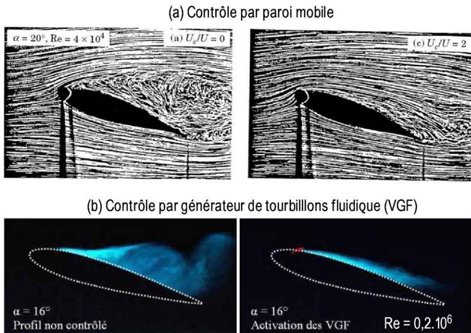
Figure 3.4 – Contr le de la s paration par (a) paroi mobile [Modi'97] et par (b) g n rateurs de tourbillons fluïdiques [Bourgeois'07]
