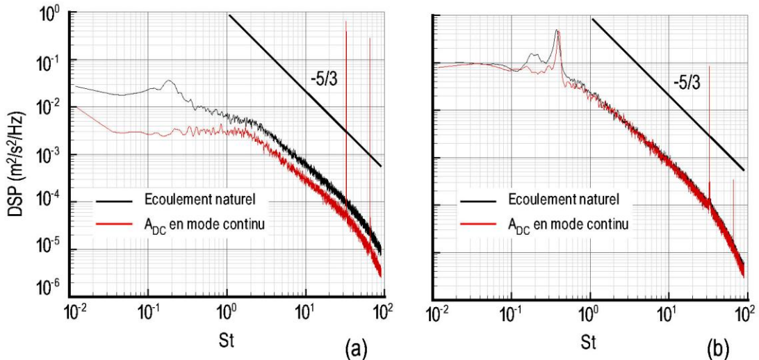
Figure 4.27 – Densités spectrales de puissance pour le mode continu (a) à hauteur de la lunette arrière et (b) au culot ( Re = 6,7 \cdot 10^5 )
