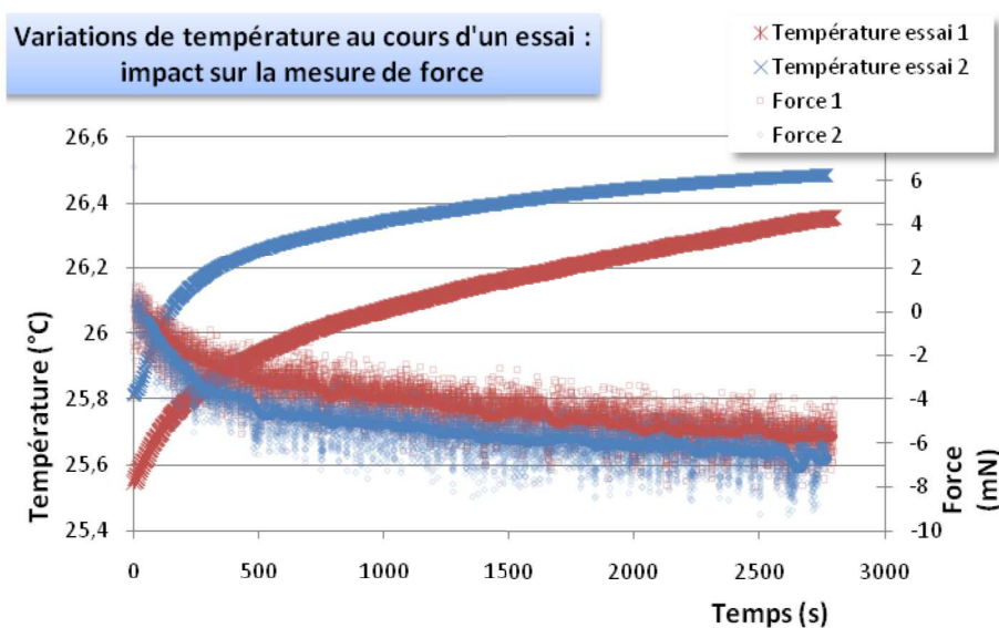
FIG. A7-8 – Caractérisation thermique n°3 – Variations enregistrées lors d'un essai de microtraction (à vide). Impact des variations de température sur les niveaux de force et comparaison avec bruit de mesure.
