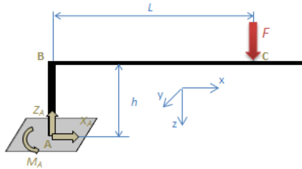
FIG. A3 - 1 – Prise en compte de la déformation de l'ancrage d'une micropoutre encastrée-libre à l'aide d'un portique console. La poutre est de dimension L \times w \times t , et l'ancrage de dimension h \times w \times t_s . Il est assimilé à une poutre courte.
