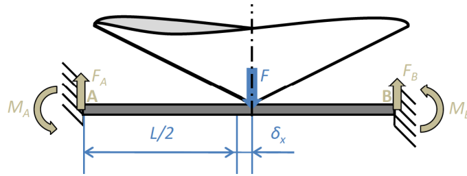
FIG. III - 8 – Schéma représentant une poutre doublement encastree en A et B. Une force F est appliquée de manière excentree à une distance \delta_x du centre de la poutre de longueur L .
