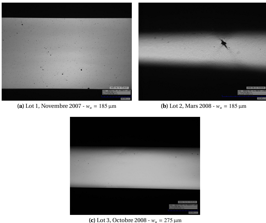
FIG. III4-16 – Comparaison de micrographies d'éprouvettes d'aluminium issues des trois lots différents (épaisseurs égales, t = 1 \mu\text{m} ). On observe une diminution globale de la densité de défaut, avec une probabilité de défauts isolés de taille critique persistante sur le lot 2. Le lot 3 présente une faible densité de défaut, et l'absence d'hétérogénéités dans l'éprouvette.
