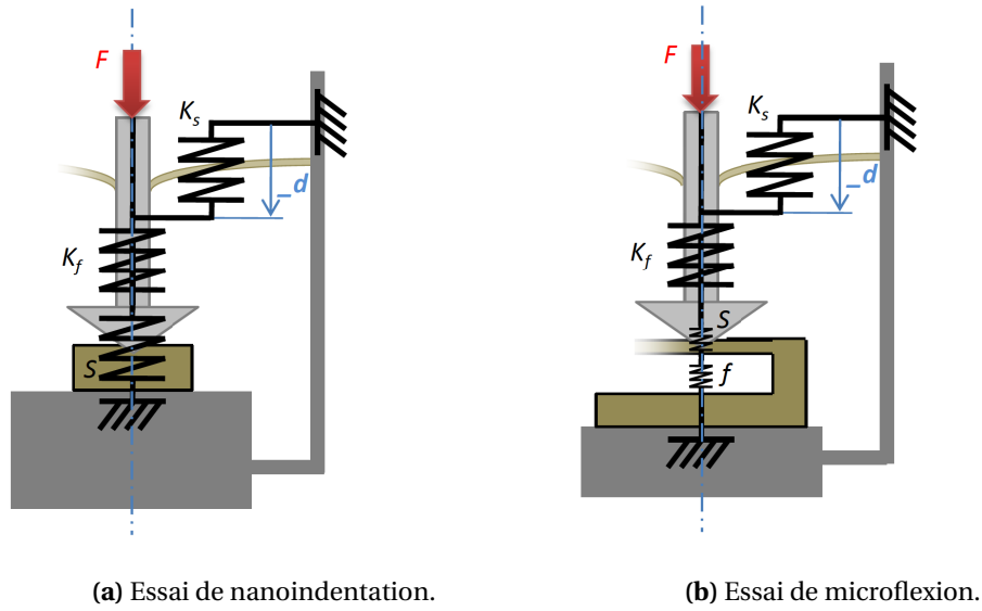
FIG. III - 2 – Représentation d'un essai d'indentation et d'un essai de microflexion (essai quasi-statique). Le déplacement d mesuré est (a) dans un cas égal à l'enfoncement du poinçon dans la matière, et (b) dans le second cas égal à la somme de cet enfoncement et de la flexion de la micropoutre. Il est calculé à partir de la mesure \_d et se trouve donc corrigé de la déformation de la colonne (équation III.3).
