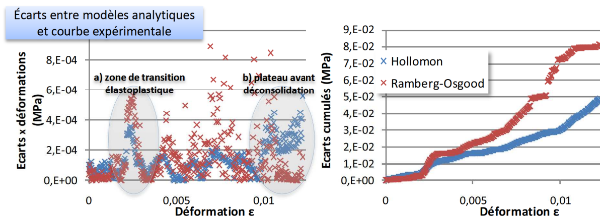
FIG. III3 - 5 – Caractérisation d'un film d'aluminium évaporé (éprouvette Alu800w3) : comparaison des approximations liées au choix d'une loi de type Hollomon ou de type Ramberg-Osgood. Deux zones particulières sont identifiées. La zone de transition élastoplastique est modélisée avec une meilleure précision par une loi de type Hollomon, tandis que la loi de Ramberg-Osgood est mieux adaptée à la description du plateau à charge maximale.
