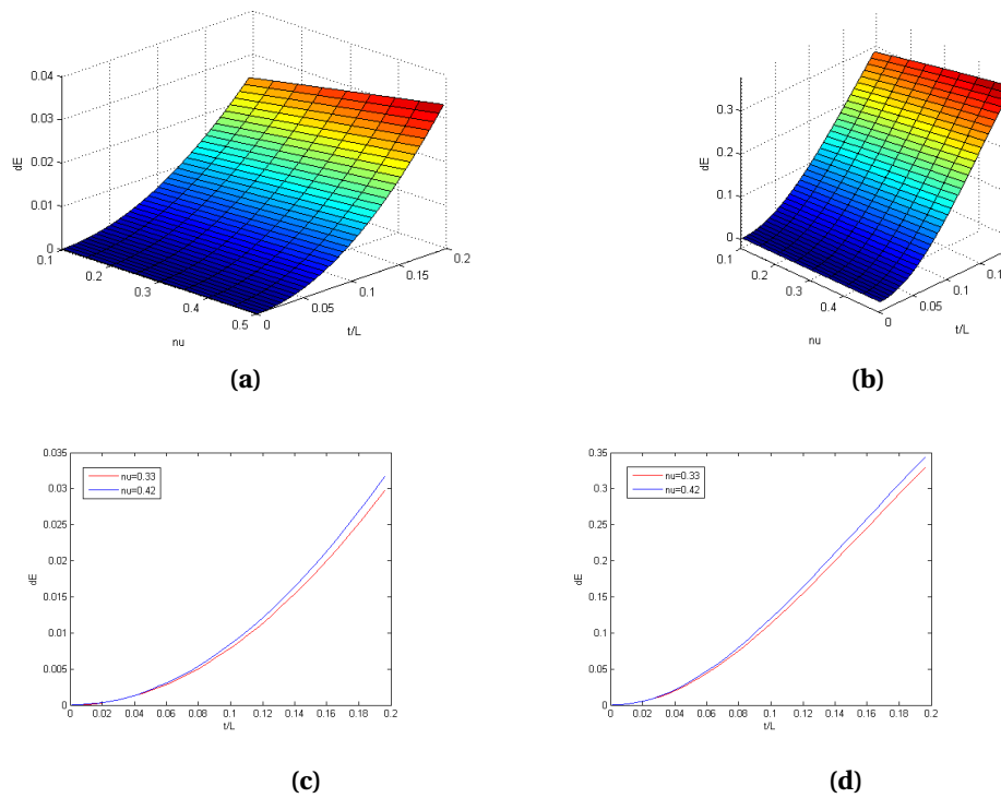
FIG. I3 - 11 – Erreurs introduites sur l'estimation du module d'élasticité E en fonction du coefficient de Poisson \nu et du rapport entre l'épaisseur et la largeur t/L pour une poutre (a) encastrée-libre et (b) encastrée-encastrée ; (c) et (d) sont les projections respectives pour \nu = 0,42 (Au) et \nu = 0,33 (Al).
