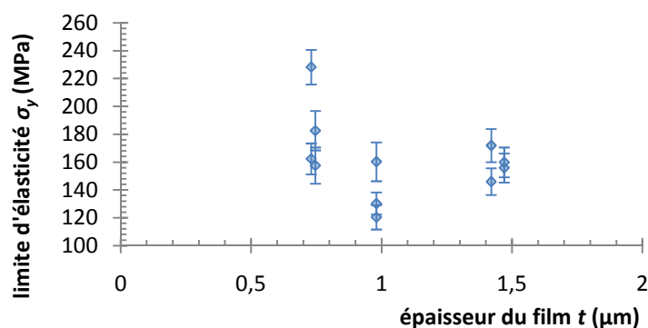
FIG. III3 - 7 – Ensemble des essais réalisés sur les éprouvettes d'aluminium. Aucune corrélation ne se distingue clairement entre la limite d'élasticité et l'épaisseur des films.
