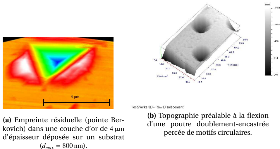
FIG. III - 11 – Différents cas d'utilisation du module Nanovision TM réalisés sur des structures en or fabriquées dans le cadre du projet MEMSFIAB.
