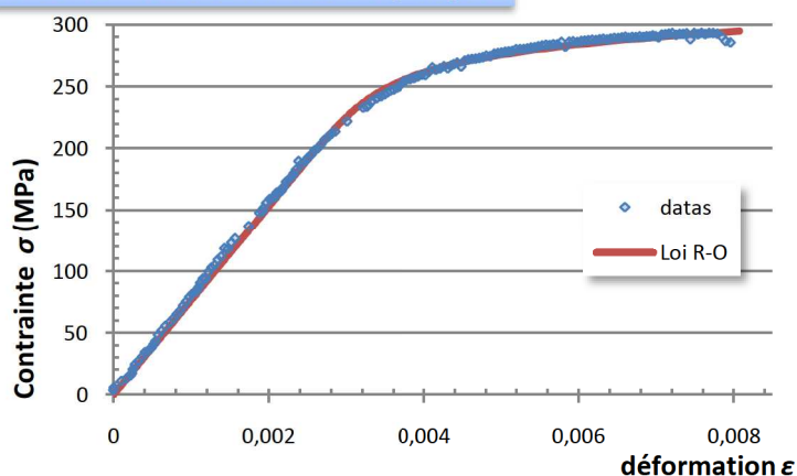
IV, 300-2: Modélisation Ramberg-Osgood
