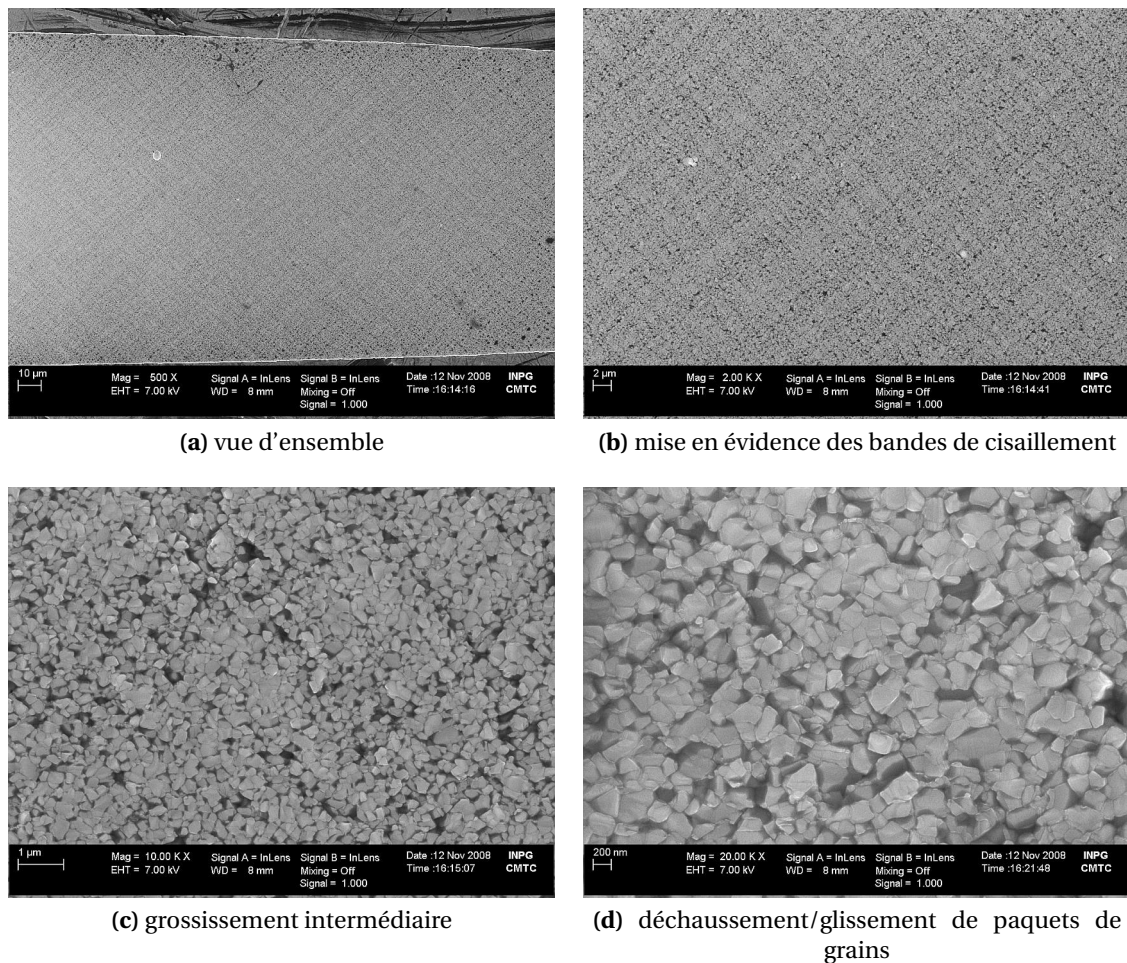
FIG. III4-18 – Éprouvette d'aluminium ayant subi un essai de traction. Les grossissements successifs mettent en évidence la nature des bandes de cisaillement observées à l'échelle macroscopique : on observe un glissement coopératif par paquets de grains le long de direction inclinées de 45^\circ par rapport à l'axe de traction.
