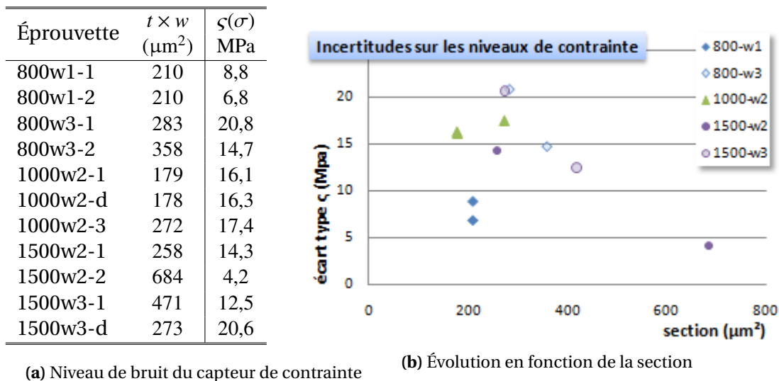
FIG. III1 - 9 – Niveau du bruit sur les mesures de contraintes en fonction de la section des éprouvettes.
