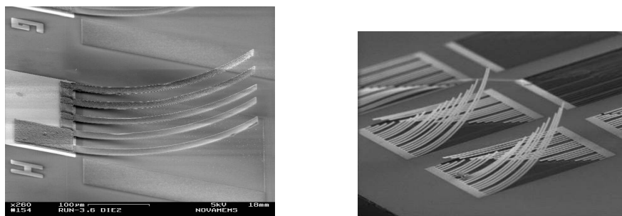
FIG. I2 - 2 – Exemples de poutres encastées-libres avec un gradient de contrainte interne normal au film : lors du retrait de la couche sacrificielle, les poutres s'accroissent en se recourbant vers le haut.
