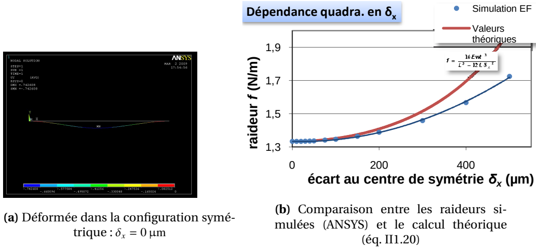
FIG. III - 9 – Simulation par éléments finis de la déformation d'une poutre 3\,000 \times 300 \times 5 \mu\text{m}^3 lors de l'application d'une charge ponctuelle avec une erreur de positionnement longitudinale.
