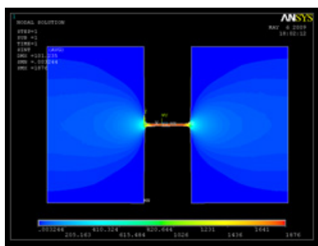
FIG. II3 - 16 – Simulation par éléments finis (ANSYS TM ) d'un essai de traction sur une éprouvette de section 200 \times 1 \mu\text{m}^2 , constituée d'un matériau élastique ( E = 70 \text{ GPa} ) et isotrope. Les conditions aux limites imposées sur les ancrages ( u_z = 0 \mu\text{m} ) simulent un film autoportant sans adhérence sur le substrat. L'hypothèse d'indéformabilité des ancrages est invalide dans ce cas.
