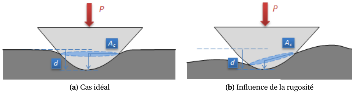
FIG. III2-17 – Assimilation du défaut de pointe à un contact de Hertz : modification du coefficient de forme K (relation entre l'aire de contact A_c et le déplacement du poinçon d ) en raison de la rugosité de surface.
