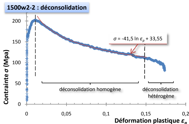
FIG. III3 - 8 – Aluminium, éprouvette « 1500w2-2 ». La déconsolidation plastique se décompose en deux phases : une déconsolidation homogène, jusqu'à 15 % environ d'allongement, puis une déconsolidation hétérogène jusqu'à la rupture finale. La première phase peut s'exprimer analytiquement sous la forme d'une relation logarithmique.
