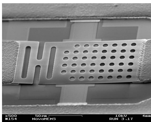
FIG. I1 - 9 – Exemple de structure collée par « stiction » (fabrication BOSH/IMEC, dans le cadre du projet MIPA).
