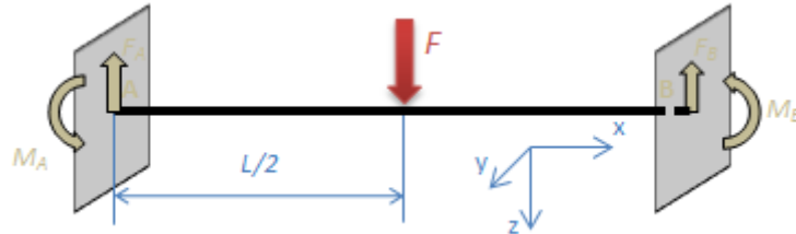
(b) Poutre doublement encastree de dimensions L \times w \times t chargée en son centre. Compte tenu des deux encastrements, ce modèle est hyperstatique d'ordre 2. Cependant, la symétrie du problème permet de réduire cet ordre d'une unité.
