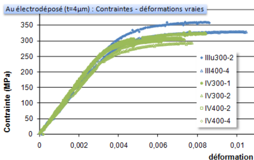
FIG. III1 - 2 – Superposition des résultats obtenus pour 6 éprouvettes d'or issues des lots 3 et 4 du LAAS. Ces courbes représentent les contraintes et déformations vraies. En particulier, aucune différence significative ne semble apparaître entre deux largeurs d'éprouvettes différentes.
