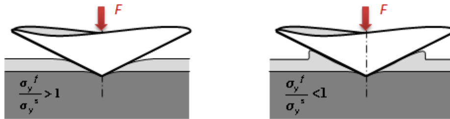
FIG. I3 - 6 – Nanoindentation sur un film mince. a) film « dur » sur substrat « mou » : Le substrat accomode plastiquement la déformation, l'enfoncement autour de l'empreinte est renforcé. b) film « mou » sur substrat « dur » : le bourrelet est renforcé car le substrat empêche la matière de s'enfoncer.
