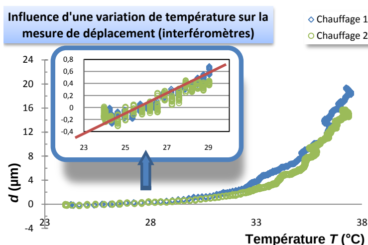
FIG. II2 - 14 – Variations de la mesure de déplacement en fonction de la température. L'encart présente une vue agrandie de la plage [24-26]°C dans laquelle les essais de traction sont réalisés. La caractéristique est considérée comme linéaire sur cette plage de fonctionnement.
