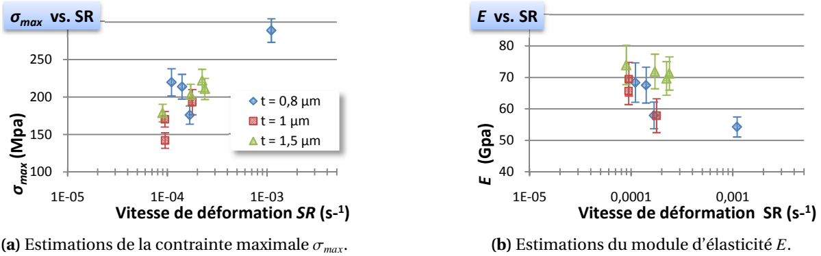
FIG. III-14 – Représentation des estimations de la contrainte maximale \sigma_{max} et du module d'élasticité E en fonction de la vitesse de sollicitation exercée. Pour l'estimation du module, les barres d'erreurs représentent l'amplitude de l'intervalle sur lequel le coefficient de corrélation de la régression linéaire dépasse 99 % de sa valeur maximale. Dans le cas de la contrainte maximale, elles représentent le niveau de bruit résultant du bruit blanc gaussien du capteur de force.
