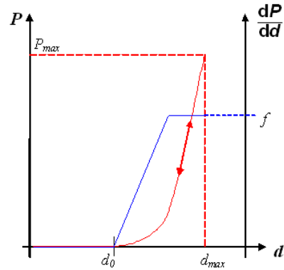
FIG. I3 - 9 – Courbe Charge-Déplacement dans le cas d'un essai de microflexion, avec des faibles déplacements. Pour un matériau linéaire, la charge et la décharge sont superposées et la raideur f est donnée par la dérivée de F(d) .
