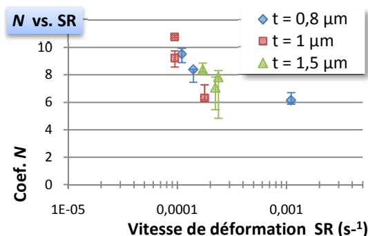
FIG. III3 - 6 – Éprouvettes d'aluminium : dépendance du coefficient d'écrouissage N à la vitesse de déformation. Les barres d'erreur représentent l'incertitude de détermination de N en fonction de la délimitation du domaine de la courbe de consolidation qui est exploité pour la régression logarithmique.
