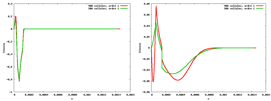
FIG. 2.5.5 – Vitesse à 1 \mu\text{s} et 10 \mu\text{s} .
