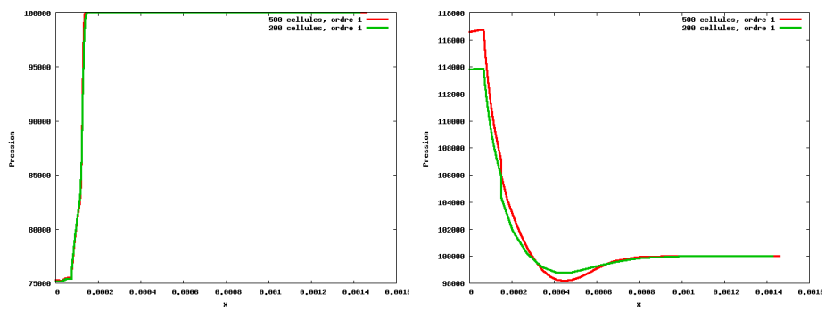
FIG. 2.5.6 – Pression à 1 \mu\text{s} et 10 \mu\text{s} .
