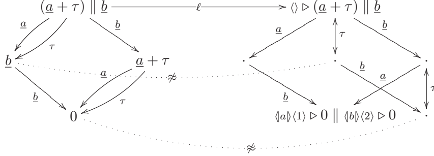
EXEMPLE 4.1.1 – Les systèmes ne sont pas bisimilaires : les choix non validés sont réversibles.
