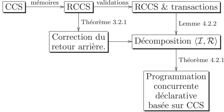
FIG. 7.1 – Programmation déclarative avec RCCS.
