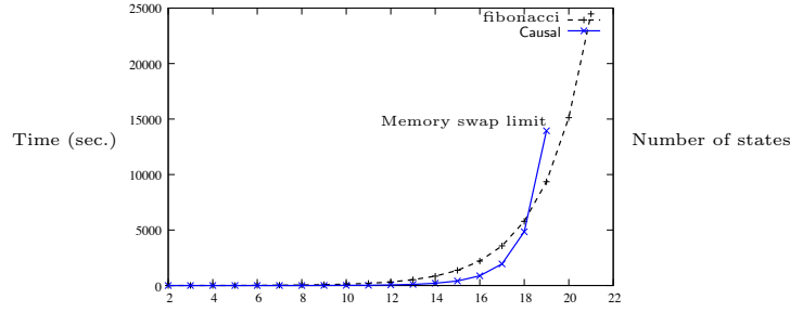
FIG. 6.5 – Méthode indirecte utilisant le CTS de p_{part} .
