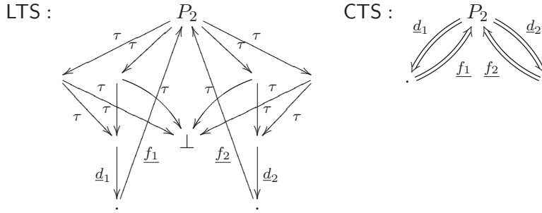
EXEMPLE 4.2.1 – LTS et CTS du code des philosophes avec état verrou.
