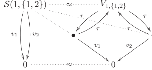
FIG. 1.5 – Correction des m votants avec retour arrière.
