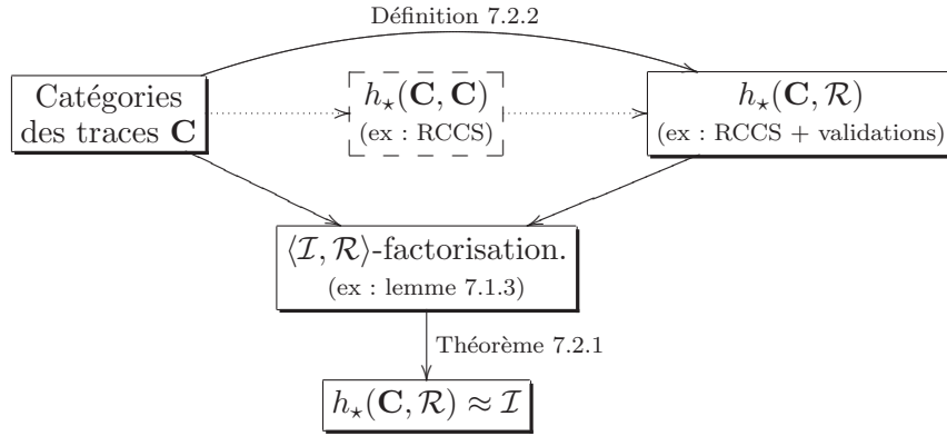
FIG. 7.2 – Programmation déclarative généralisée.
