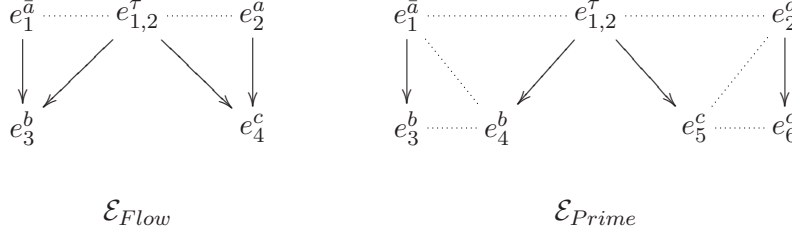
FIG. 5.2 – Structures d'événements de p := \bar{a}.b \mid a.c , avec \lambda(e_i^\alpha) = \alpha .
