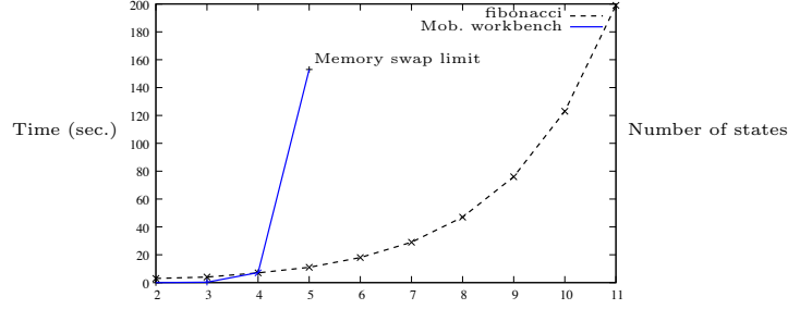
FIG. 6.4 – Test de bisimulation pour le code complet p_{comp} .
