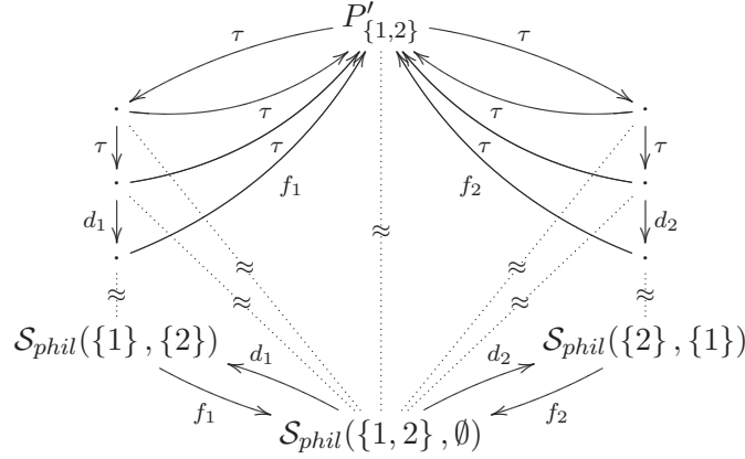
FIG. 1.6 – Correction du système à 2 philosophes avec retour arrière.
