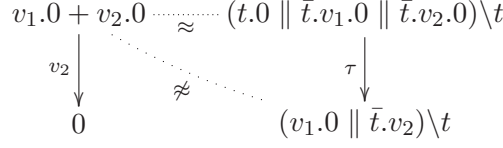
FIG. 1.4 – Les systèmes ne sont pas bisimilaires.
