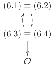
FIG. 6.2 – CTS à états dans les structures récursives.
