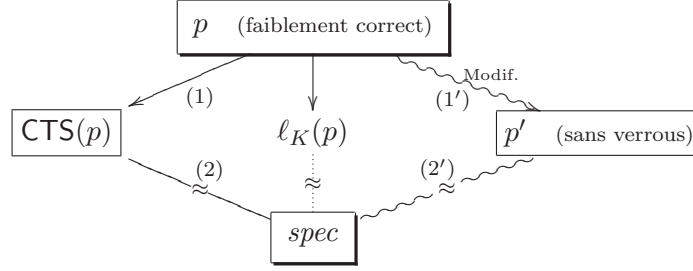
FIG. 5.1 – Programmation concurrente déclarative et méthode standard.
