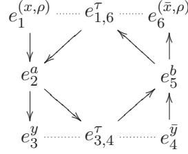
EXEMPLE 5.2.1 – Structure de flot résultant de \mathcal{U}(p) .
