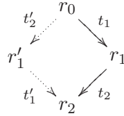
LEMME 3.1.1 – Diamant de concurrence.
