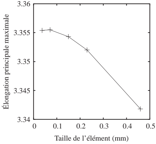
FIG. 5.8 – Elongation principale maximale pour une torsion de 175° en fonction de la taille des éléments.
