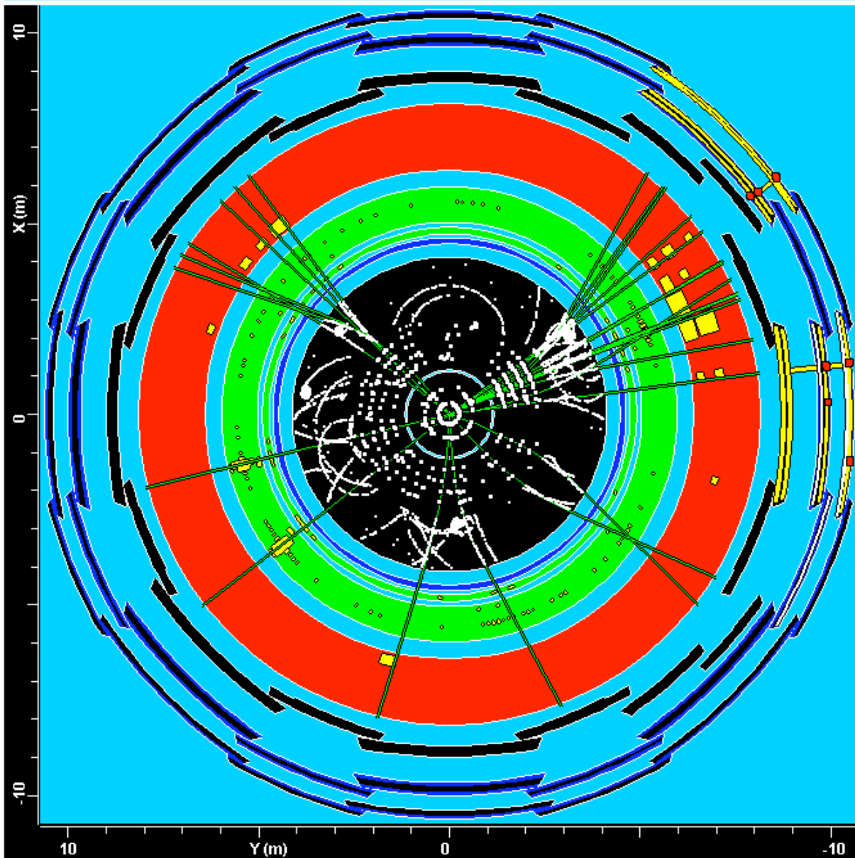
FIGURE 3.37: Représentation d'un événement du signal Z_H \rightarrow ll q\bar{q}ll avec M_{Z_H} = 1 TeV. En haut à droite sont visibles une paire de muons et les jets, issus du Higgs, et de l'autre côté une paire d'électrons
