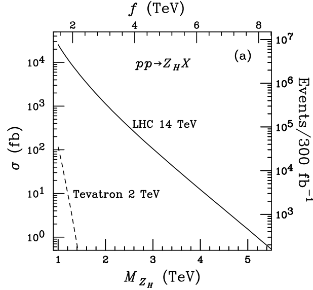
FIGURE 3.23: Section efficace de production du boson de jauge lourd Z_H , en fonction de sa masse et de f , pour \cot \theta = 1 [16]. La section efficace de production de W_H est double.
