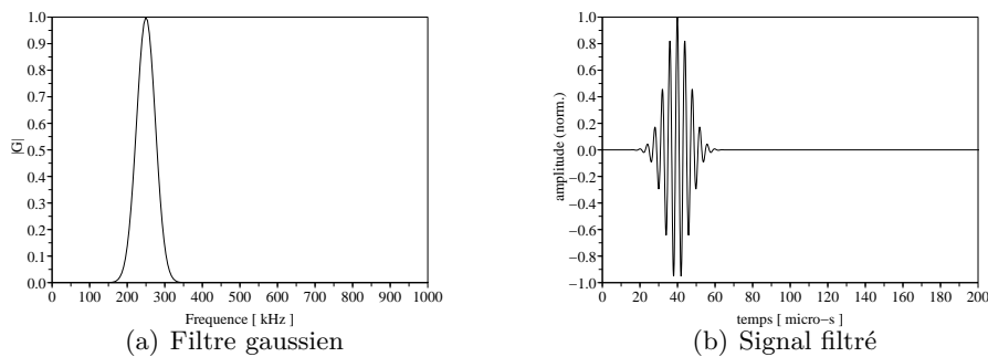
FIG. 4.16 – Exemple du filtrage d'un Dirac par un filtre gaussien centré en f_i = 250 kHz de largeur 0.07f_i (a) le signal filtré est présenté en (b)
