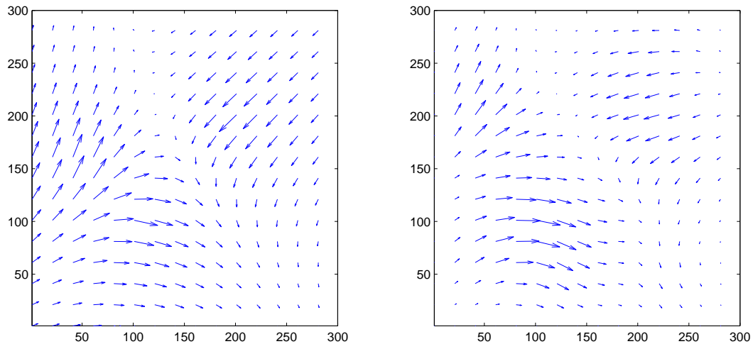
Fig. 5.3 – Gradient exact (gauche) et après inversion (droite) à partir de la décomposition en circlets et suivi des éléments.
