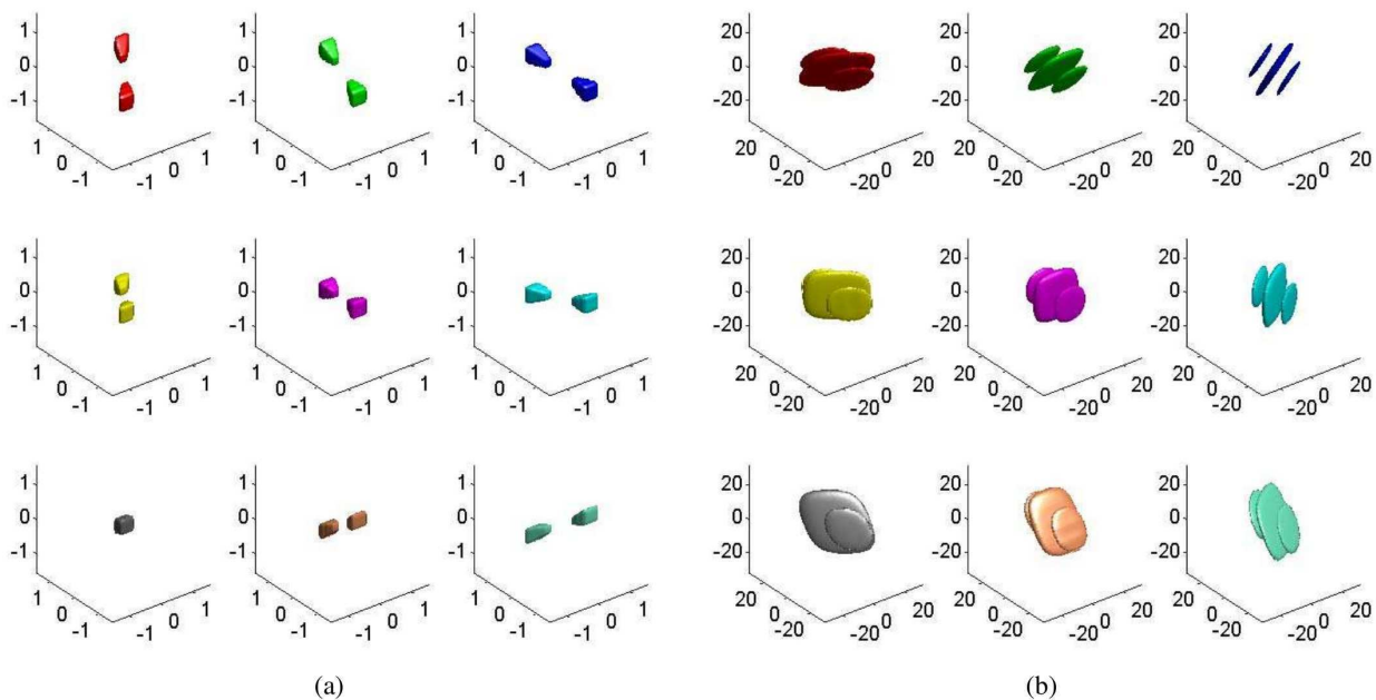
Fig. 4.10 – Exemples de curvelets 3D dans le domaine spatial (a) et dans le domaine des nombres d'onde (b) [Nguyen and Chauris, 2010].
