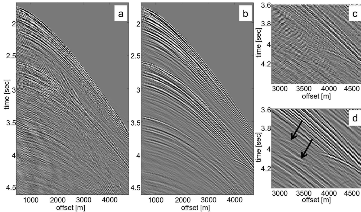
Fig. 4.12 – Prédiction des multiples pour un jeu de données réelles, (a et c) avec la méthode classique SRME, Surface-Related Multiple Elimination [Verschuur et al., 1992], (b et d) avec la prédiction dans le domaine des curvelets et la prise en compte de l'aliasing [Donno et al., 2010].
