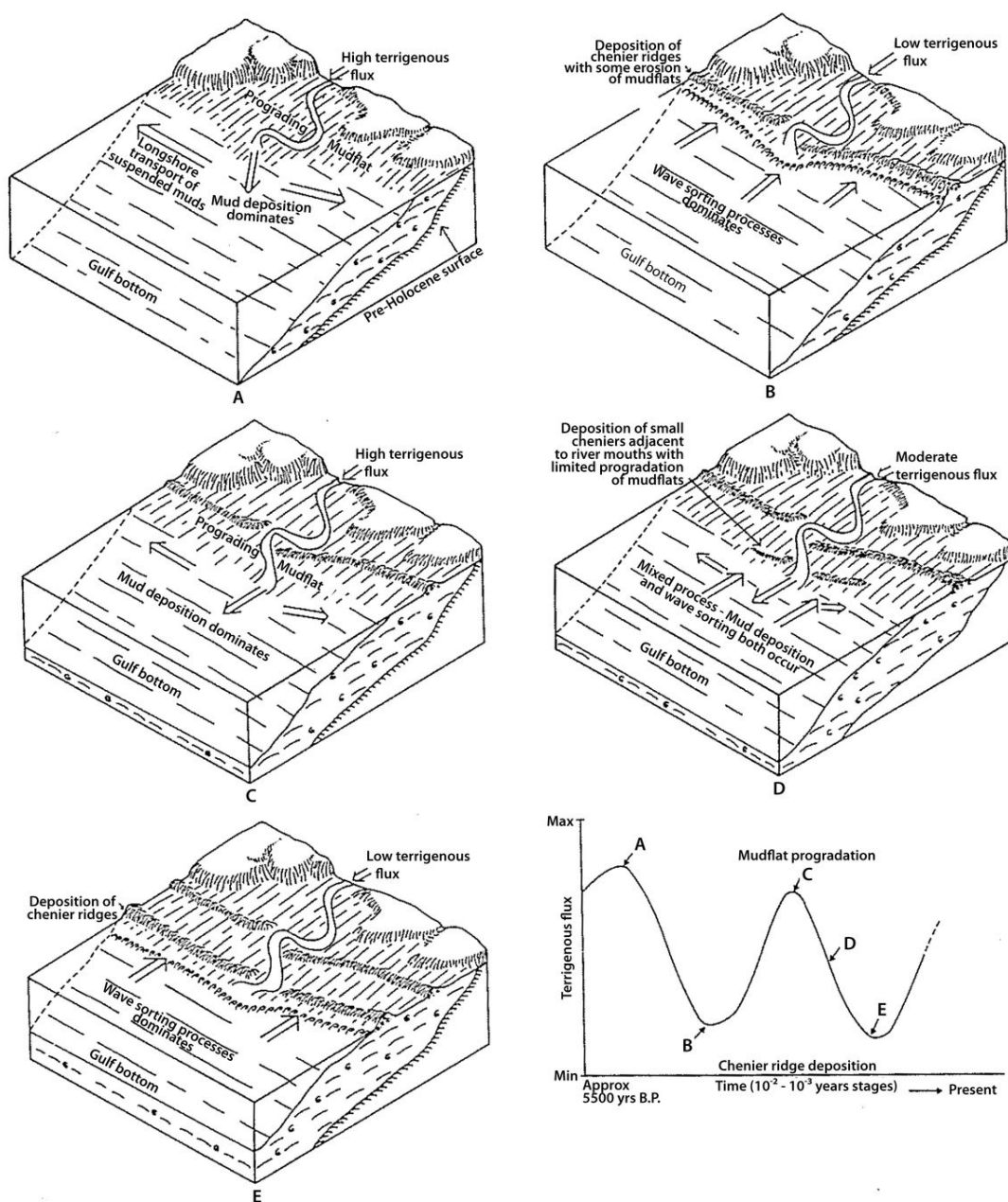
FIG. I.6 – Progradation d'une plaine de cheniers en Australie forcée par des variations du flux sédimentaire (Rhodes, 1982). Les périodes de fort apport fluvial (fortes pluies - A,C) entraînent la progradation du mudflat, alors que les périodes de faible apport (sécheresse - B,E) favorisent le remaniement des particules grossières en cheniers.
