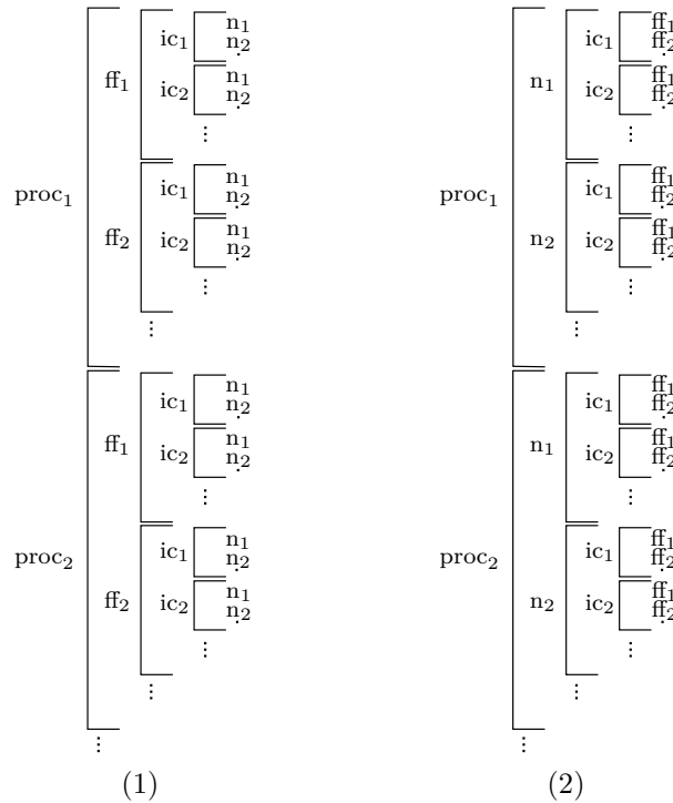
FIG. III.5 – Numérotation des inconnues en parallèle dans la librairie PELICANS
