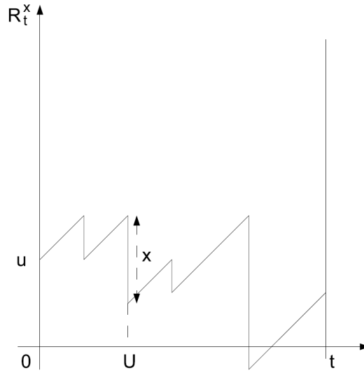
FIGURE 3. Une trajectoire du processus de risque (R_t^x)_{t \geq 0} partiellement translaté de x .
