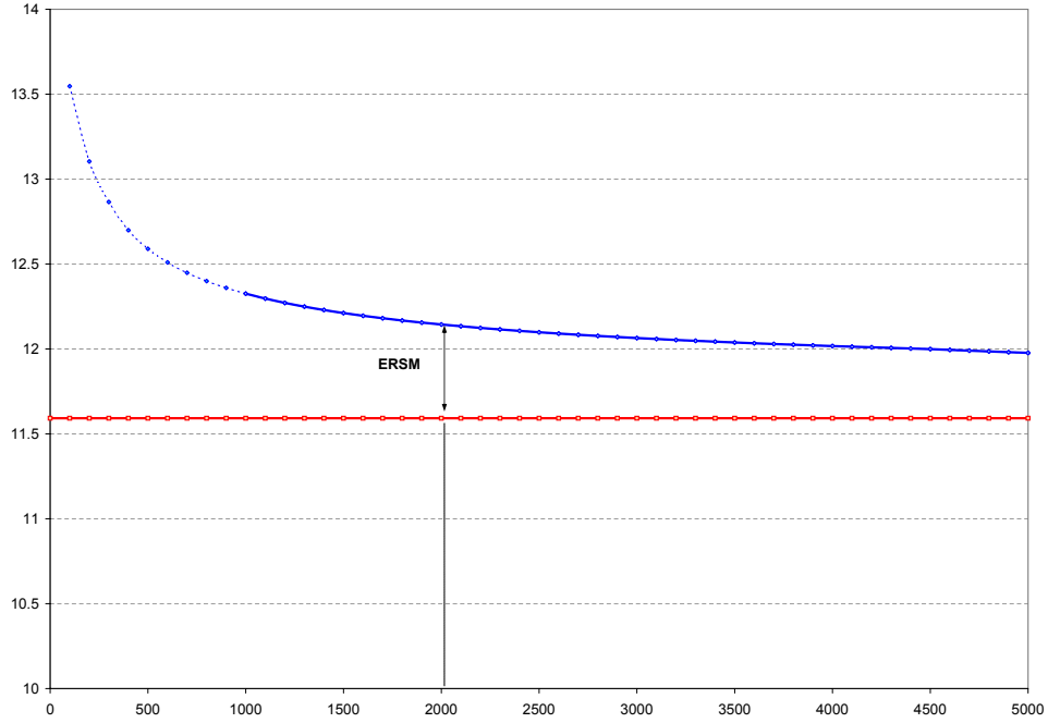
FIGURE 5. Valeurs de u_\eta et u_{\eta,\varepsilon} > u_\eta comme fonctions de N , telles que \psi(u_\eta, t) = 2\% et \tilde{\psi}_{1-\varepsilon\%}^{O_N \text{ reliable}}(u_{\eta,\varepsilon}, t) = 2\% , \lambda_0 = 1, c = 1.1, t = 10, \delta = 1, \varepsilon = 5\% .
