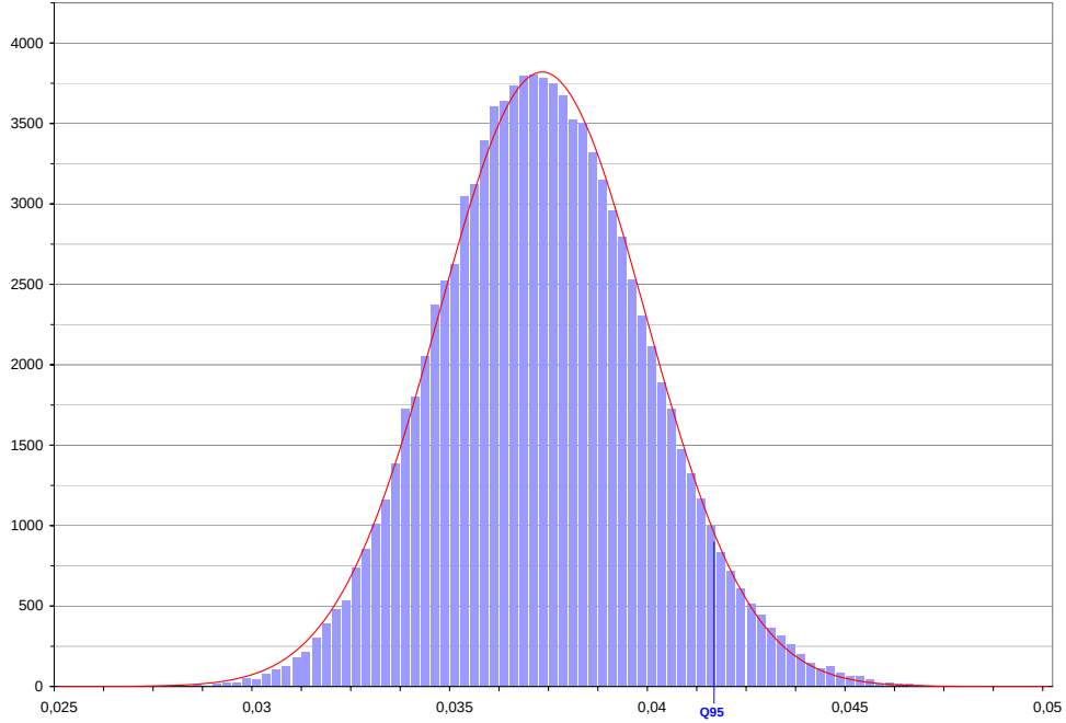
FIGURE 4. Histogramme de 100000 probabilités de ruine empiriques \psi^N(u, t) pour N = 5000 et densité d'une loi normale de moyenne \mu = \psi(u, t) et de variance Var(\text{IF}_Y[\psi(u, t)])/N , \lambda_0 = 1, c = 1.1, t = 10, u = 10, \delta = 1 . Q_{95} désigne le quantile à 95% de la probabilité de ruine.
