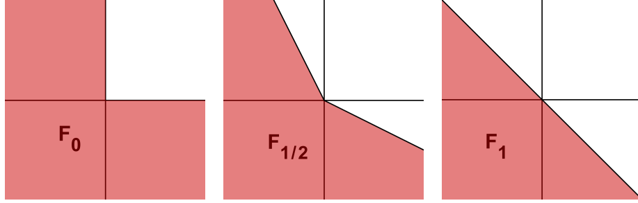
FIGURE 10. F_\beta pour \beta = 0, \frac{1}{2} et 1 en dimension 2
