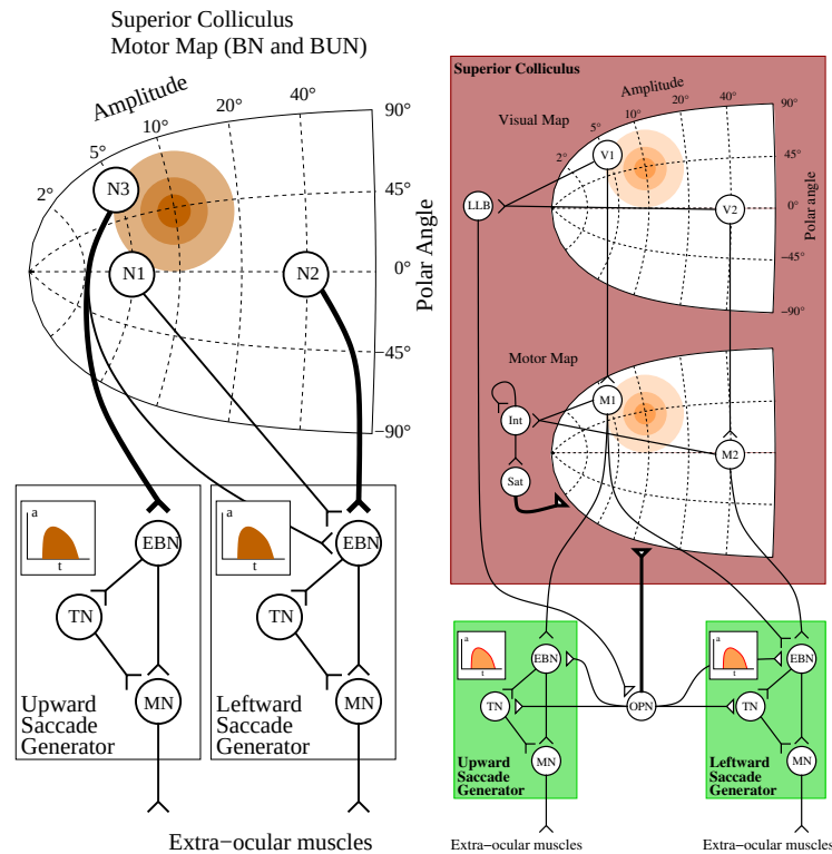
FIG. 4.1 – Gauche : Représentation du problème de la transformation spatio-temporelle. La bouffée d'activité stéréotypée dans la carte colliculaire motrice (en haut) doit être transformée en deux bouffées d'activités proportionnelles à l'amplitude des mouvements sur les axes des générateurs de saccades (en bas). Droite : Modèle computationnel de la STT de type "somme, saturation et inhibition" proposé dans (Tabareau et al., 2007).
