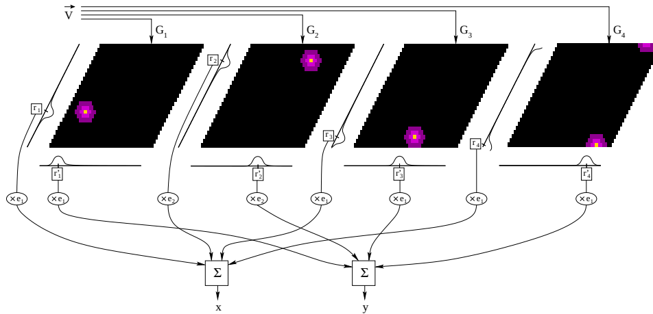
FIG. 3.7 – Modèle de décodage des cellules de grilles. La vitesse courante \vec{V} permet de mettre à jour l'activité de 4 grilles de périodes différentes ; le calcul des barycentres circulaires de l'activité des grilles projetées sur deux axes permet le décodage explicite des coordonnées du rat (pour des valeurs inférieures à 5km).
