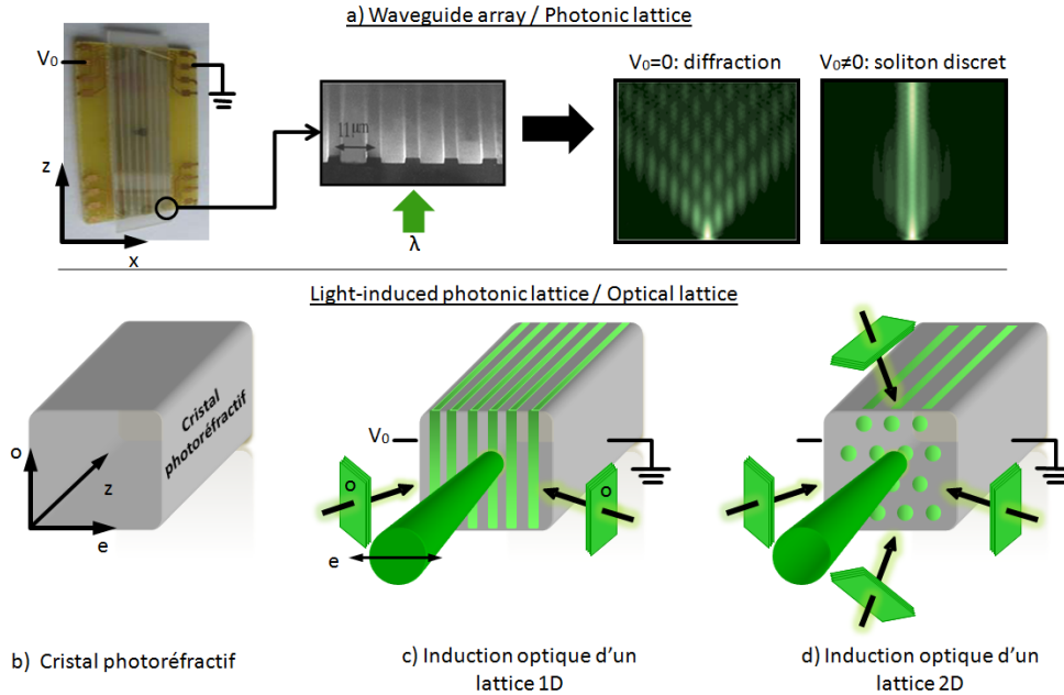
FIG. 3.2: Exemples de lattices photoniques. a) Waveguide array / photonic lattice, créé par le biais d'une technique lithographique. b-d) Schéma de l'inscription optique d'un lattice photonique (optical lattice) à l'intérieur b) d'un cristal photoréfractif par la méthode d'interférences d'ondes. c) Induction optique par 2 faisceaux cohérents (polarisés ordinairement (o)) : cas 1D. d) 4 faisceaux cohérents : cas 2D. Le faisceau vert polarisé extraordinairement (e), est utilisé pour sonder le matériau. Une tension extérieure V_0 peut être appliquée en a),c), et d) dans le cas d'étude de la formation de solitons discrets [158].
